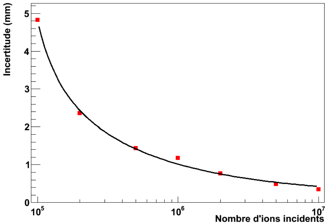
figure IV-42 : évolution de l'incertitude sur la position du point médian en fonction du nombre d'ions 12 C incidents. L'énergie du faisceau est fixe et vaut 200 MeV/u.
