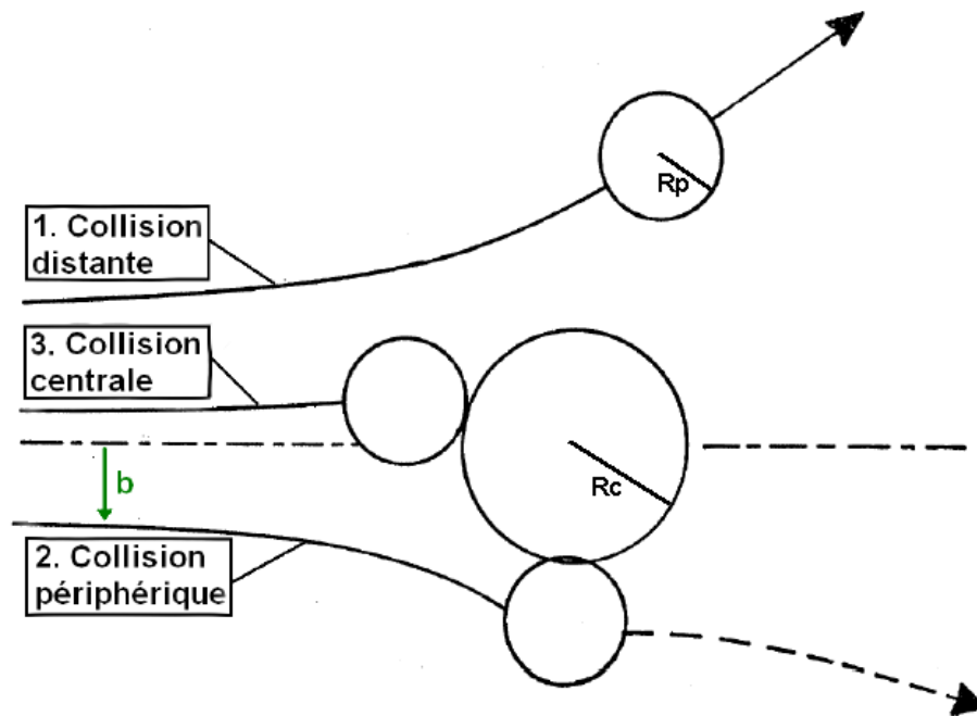
figure II-2 : schéma représentant les trois types d'interaction noyau-noyau. Si b est grand devant R_c+R_p , il s'agira d'une collision distante. Si b est de l'ordre de R_c+R_p , on aura affaire à une collision périphérique. Lorsque b tend vers 0, la collision est dite centrale.
