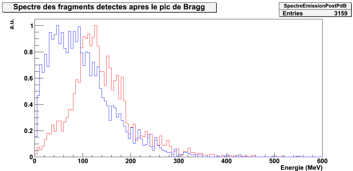
figure IV-37 : Spectre de l'énergie des fragments à l'émission (rouge) et à la détection (bleu). Tous ces fragments ont été générés en aval du pic de Bragg.
