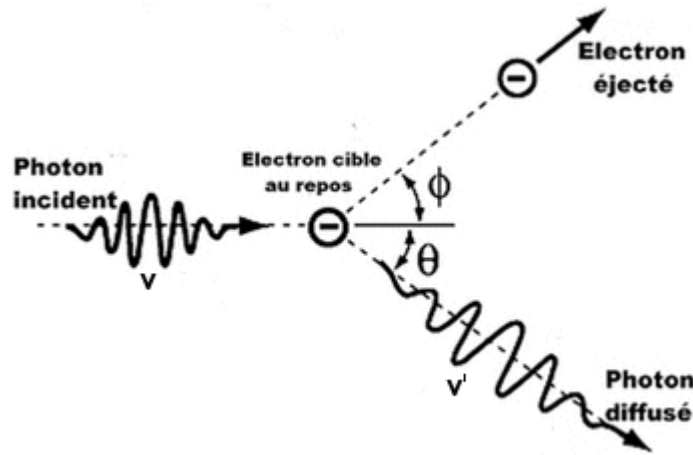
figure I-1 : Cinématique de l'effet Compton. Un photon incident de fréquence \nu interagit avec un électron libre. Il résulte de cette interaction un électron possédant une énergie cinétique E_c et un photon diffusé de fréquence \nu'
