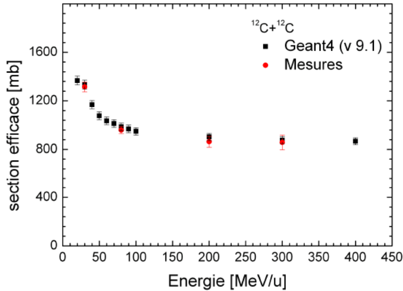
figure II-6 : Comparaison entre sections efficaces mesurées (rouge) et simulées (noir) pour la réaction ^{12}\text{C}-^{12}\text{C} en fonction de l'énergie du projectile. Un bon accord (inférieur à 10%) est observé sur l'ensemble de l'intervalle de test (tiré de [120]).
