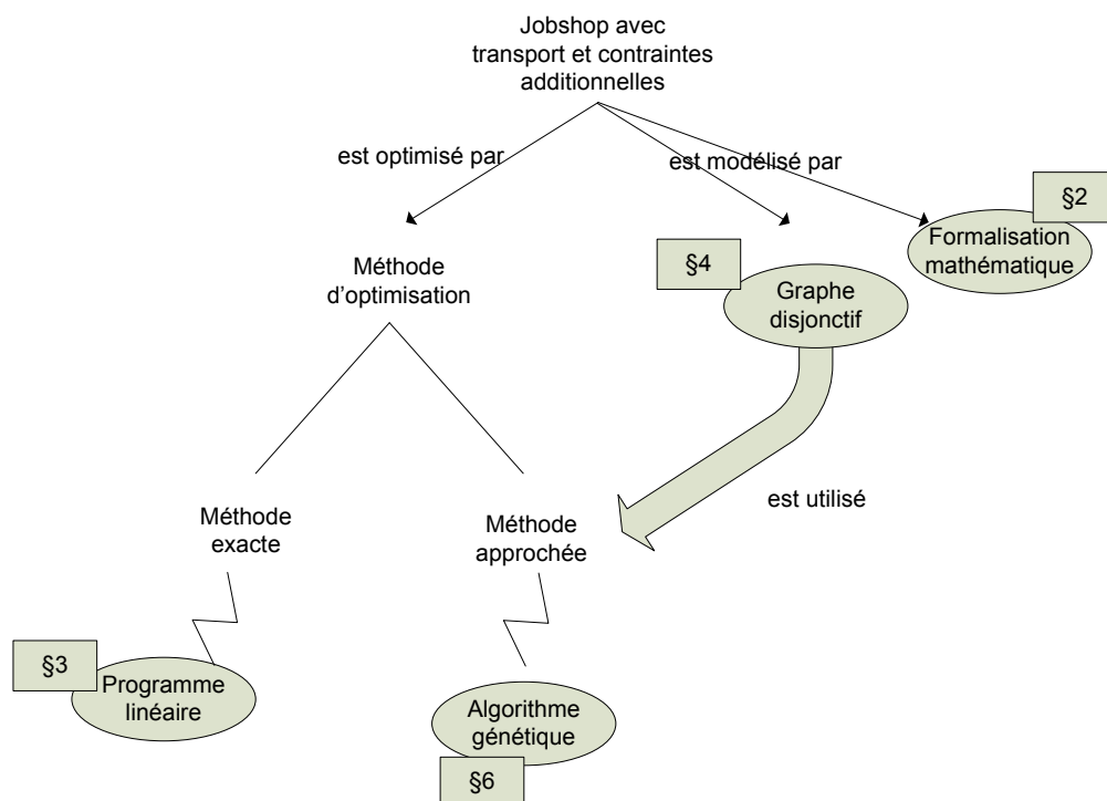
Figure 4-1. Synoptique de nos propositions pour le jobshop avec transport et contraintes additionnelles
