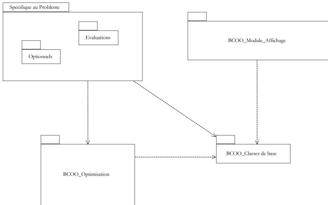
Figure 5-5. Vues globales des paquetages
