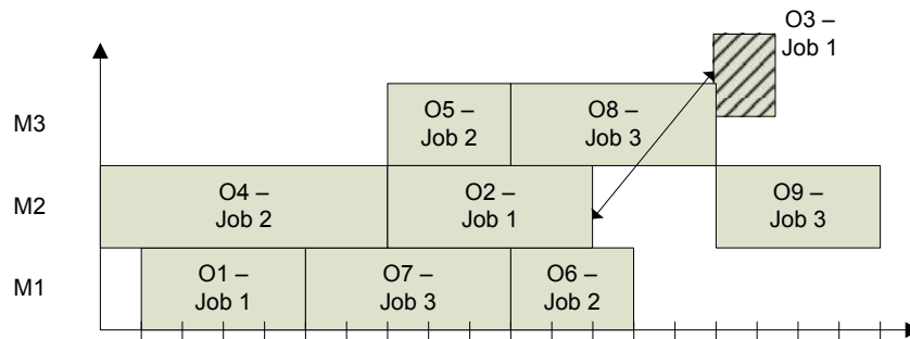
Figure 3-4. Ordonnancement partiel et contrainte de time lag maximum à respecter
