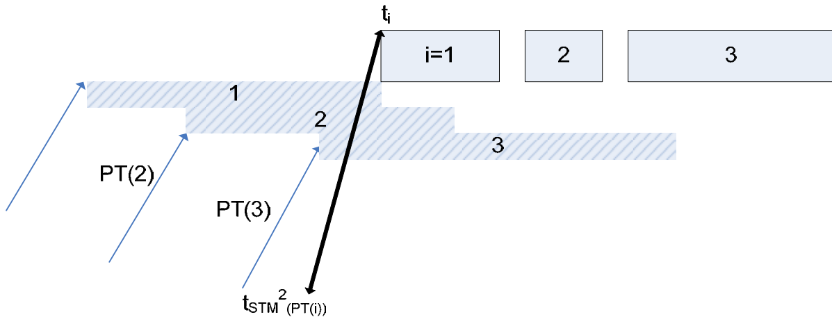
Figure 4-13. Contrainte limitant le nombre de jobs dans le stock d'entrée (ordonnancement non valide)
