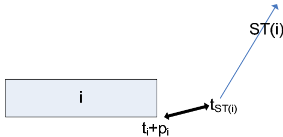
Figure 4-5. Contrainte entre les opérations machine et les opérations transport (sans anticipation)
