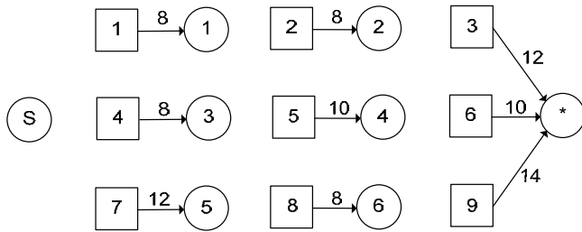
Figure 4-24. Arcs C(1) avec anticipation
