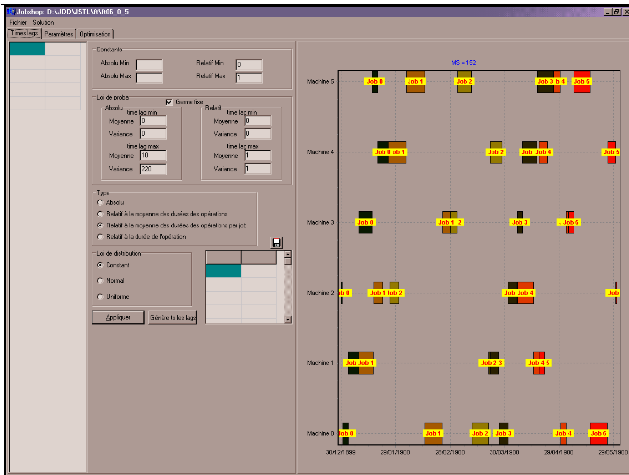
Figure 5-14. Exemple de mise en œuvre du module affichage graphique
