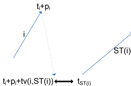
Figure 4-9. Contrainte de disjonction sur le transporteur
