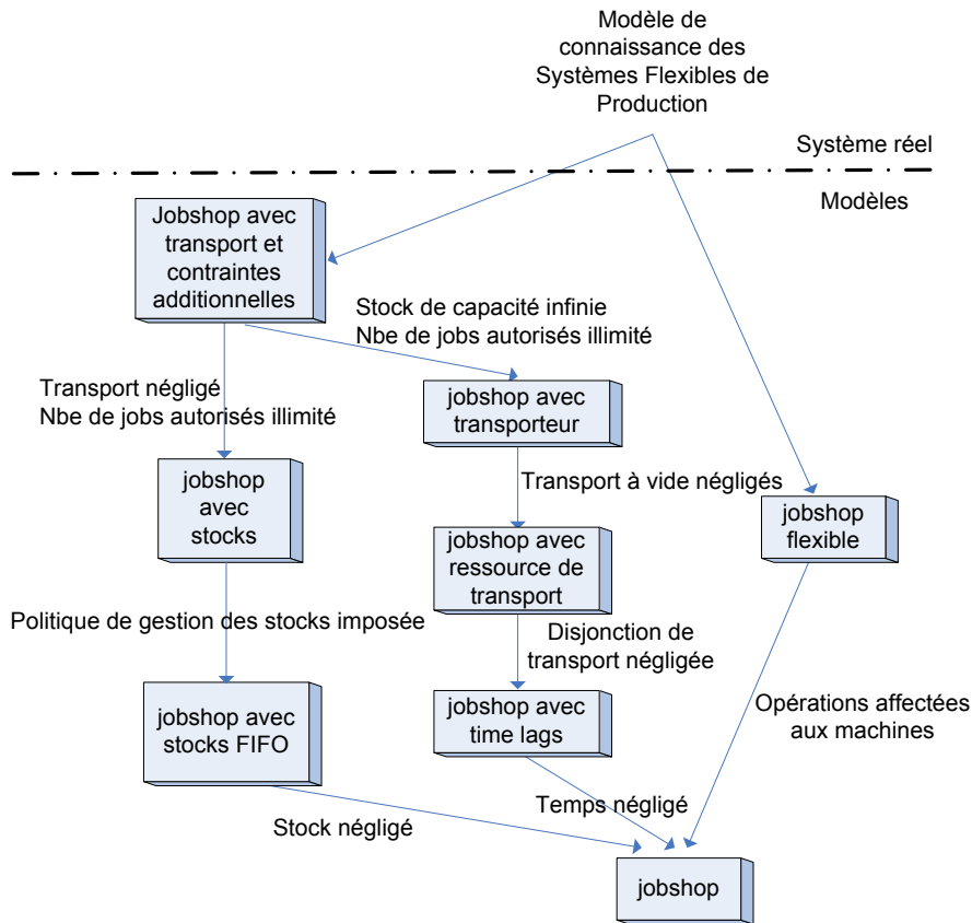
Figure 1-18. Démarche de modélisation appliquée au Systèmes Flexibles de Production
