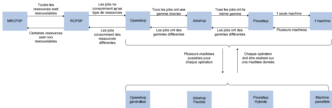
Figure 1-5. Typologie des problèmes d'ordonnement
