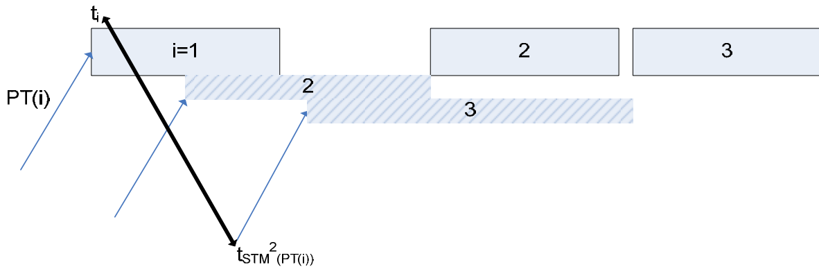
Figure 4-12. Contrainte limitant le nombre de jobs dans le stock d'entrée
