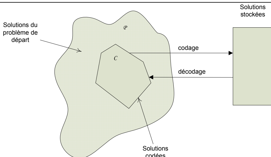
Figure 1-8. Schéma de principe de la représentation
