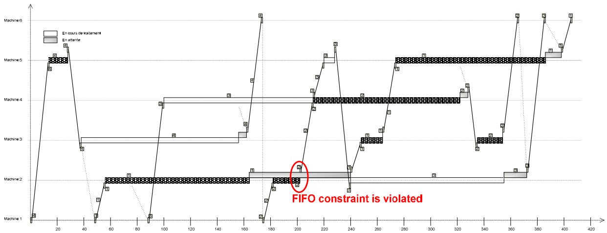
Figure 4-22. Gantt d'une solution pour le Jobset 1H, n = 4 , N = 3 et gestion optimale des stocks
