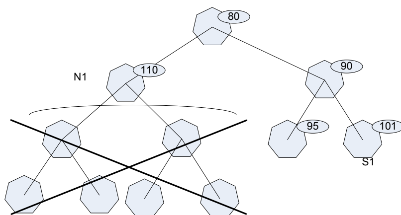
Figure 1-14. Méthode de séparation / évaluation
