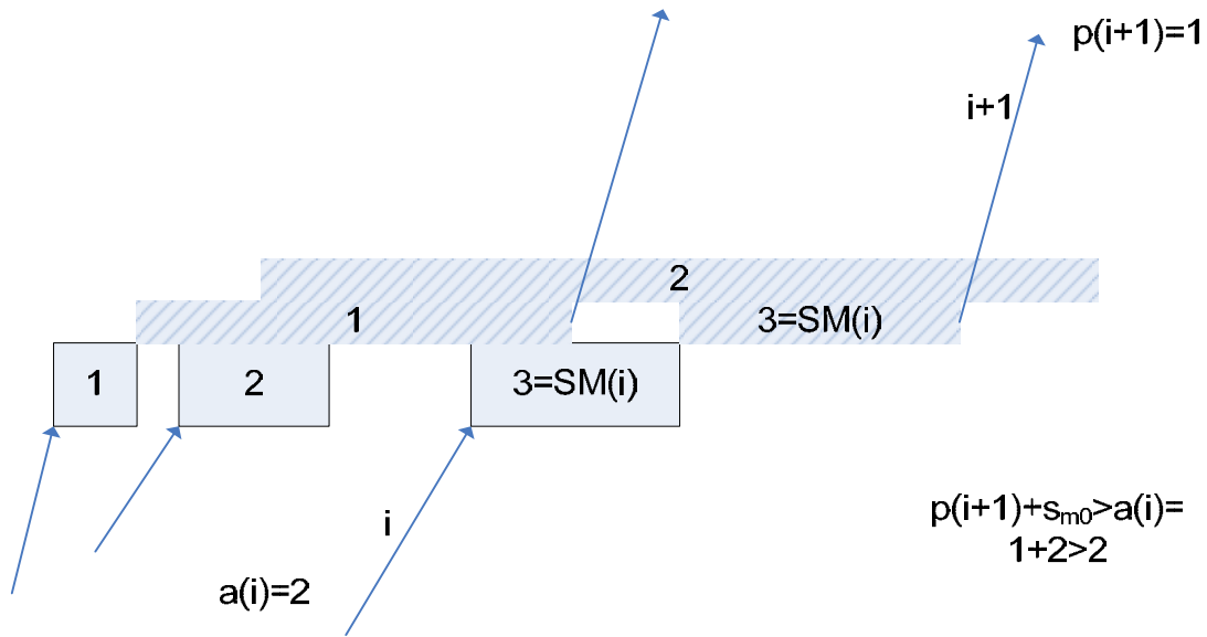
Figure 4-15. Contrainte limitant le nombre de jobs dans le stock de sortie (contrainte vérifiée)
