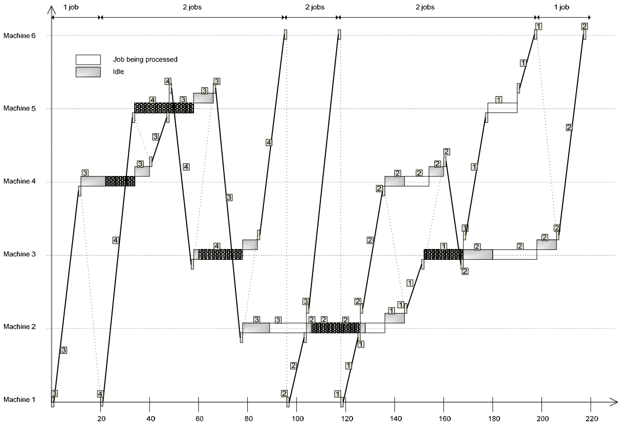
Figure 4-18. Ordonnancement optimal pour la politique optimale de gestion des stocks (N=2)
