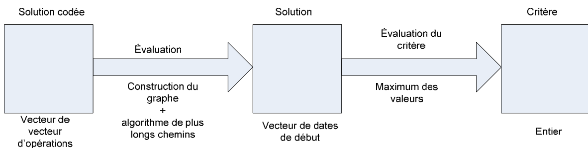
Figure 5-3. Détails de la transformation de la représentation semi active pour le jobshop
