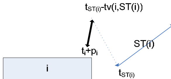
Figure 4-6. Contrainte entre les opérations machine et les opérations transport (avec anticipation)
