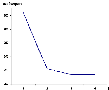
Figure 4-21. Variation du makespan en fonction de N pour le jobset 1, n=4 et p_{ij} \times 1 , t_{ij} \times 1
