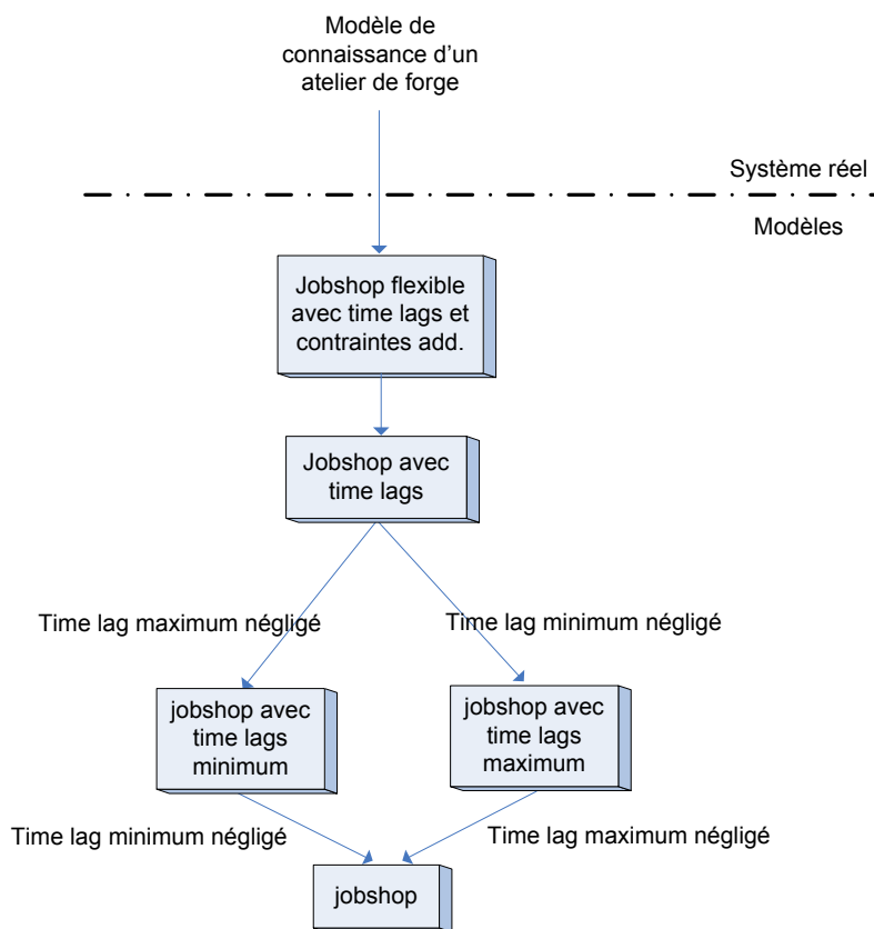
Figure 1-17. Démarche de modélisation appliquée au problème d'atelier de forge
