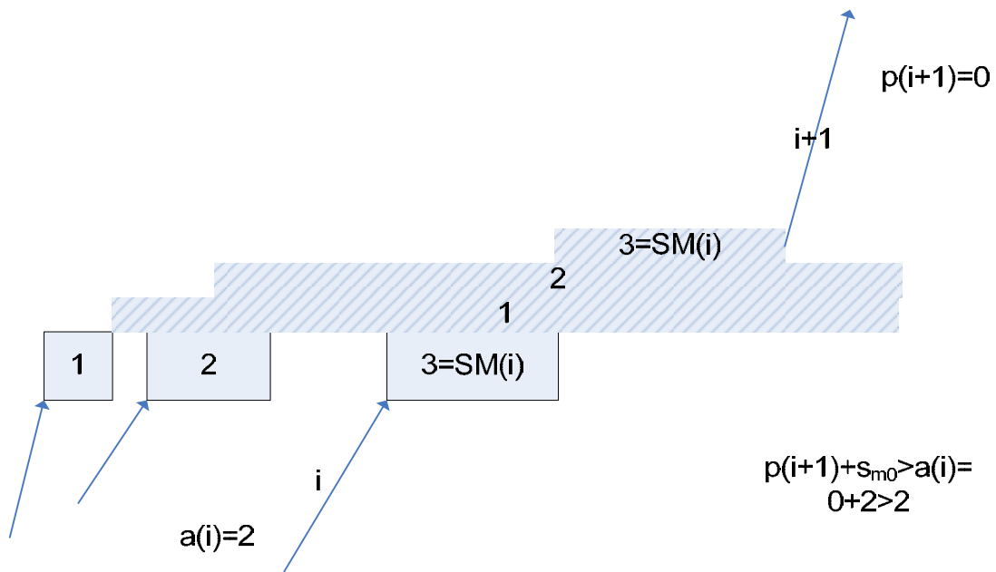
Figure 4-16. Contrainte limitant le nombre de jobs dans le stock de sortie (contrainte violée)
