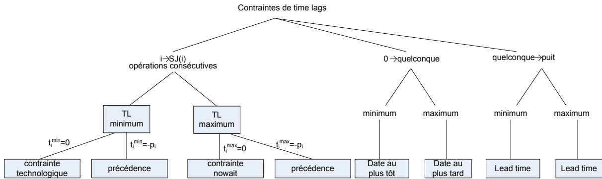
Figure 3-5. Typologie des contraintes de time lag
