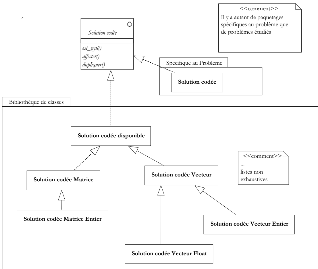
Figure 5-7. Solution codée
