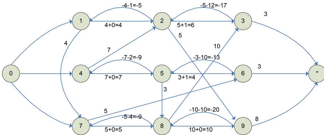
Figure 3-7. Graphe conjonctif du problème J1 avec time lags minimum et maximum
