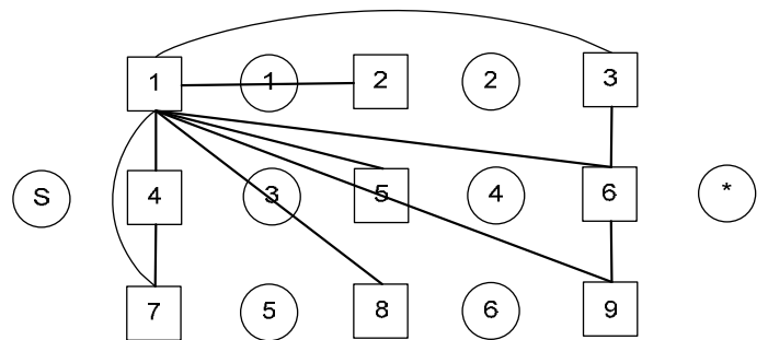
Figure 4-27. Arêtes C(4) partant de T1
