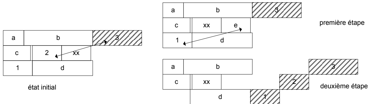
Figure 3-12. Procédure de réparation
