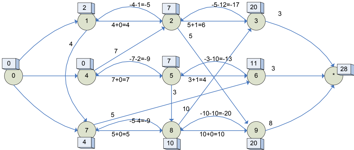
Figure 3-9. Première itération de l'algorithme
