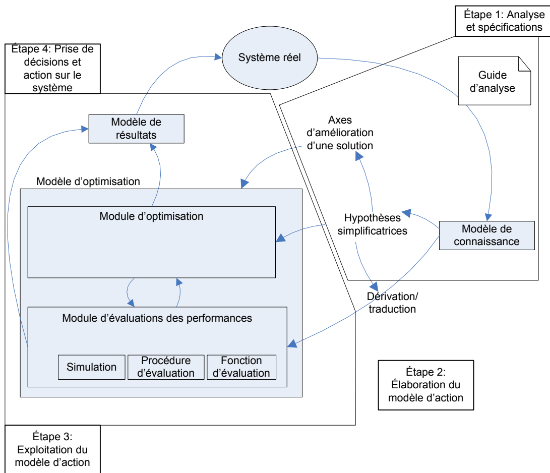
Figure 1-11. Processus de modélisation adapté aux problèmes d'optimisation
