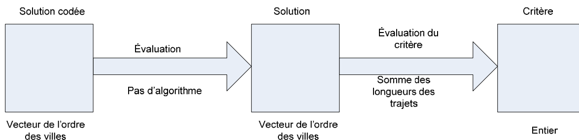
Figure 5-4. Détails de la transformation de la représentation semi active pour le TSP
