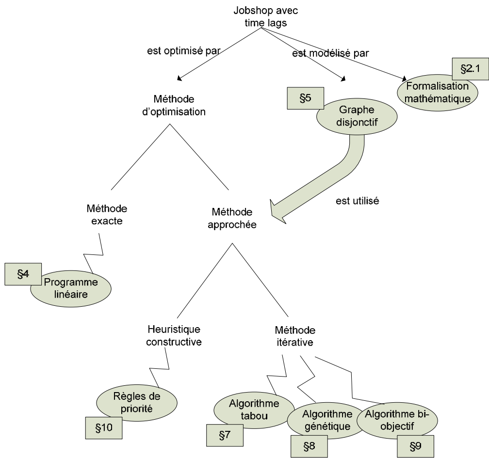
Figure 3-1. Synoptique de nos propositions pour le jobshop avec time lags
