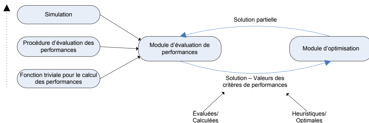
Figure 1-7. Principaux types de modules d'évaluation des performances (Sarramia, 2002).
