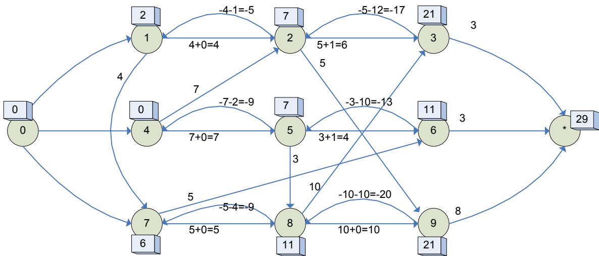
Figure 3-10. Deuxième itération de l'algorithme
