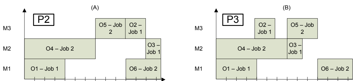
Figure 2-2. (A) est un ordonnancement optimal et non actif et (B) est l'ordonnancement actif correspondant
