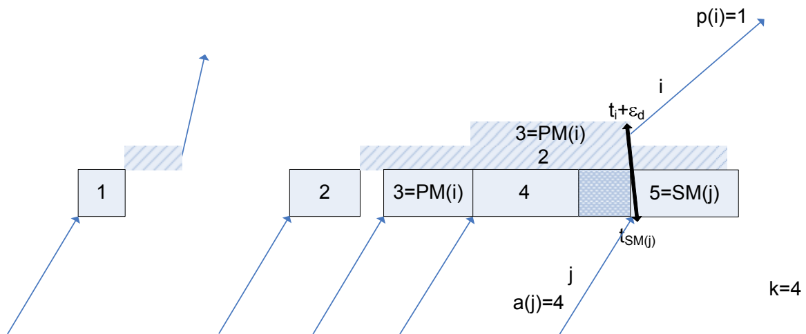
Figure 4-14. Contrainte de blocage de l'unité de traitement
