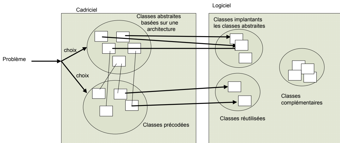
Figure 5-1. Un cadriciel en général
