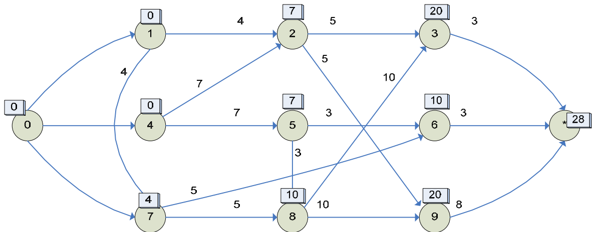
Figure 2-15. Graphe conjonctif évalué
