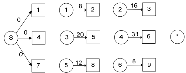
Figure 4-25. Arêtes C(3)
