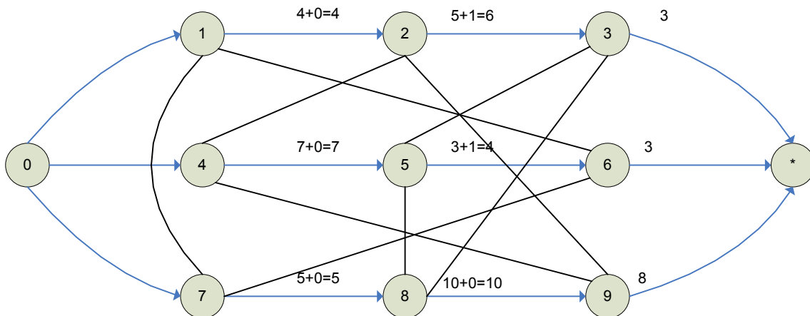
Figure 3-6. Graphe conjonctif - disjonctif du problème J1 avec time lags minimum
