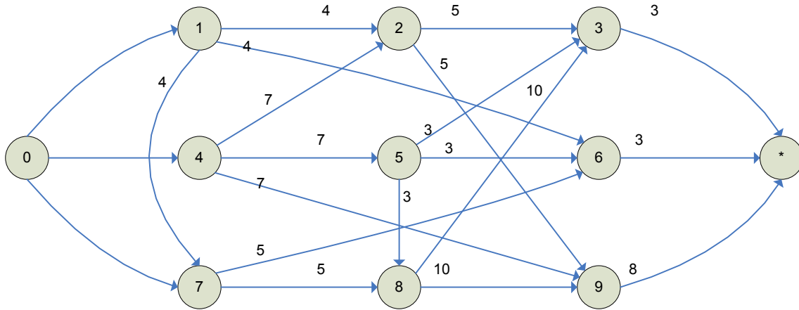
Figure 2-10. Graphe conjonctif orienté de la solution S1
