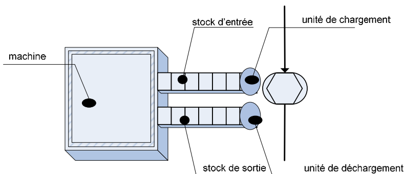
Figure 4-3. Une station
