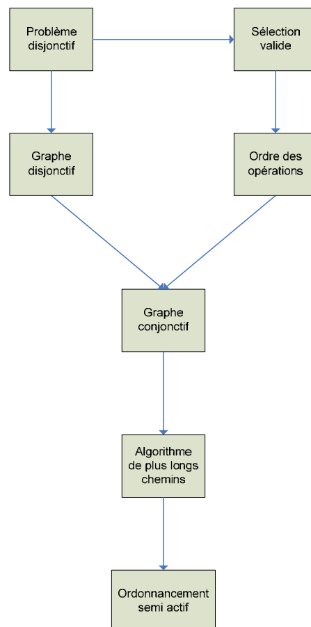
Figure 0-2. Graphe conjonctif -disjonctif
