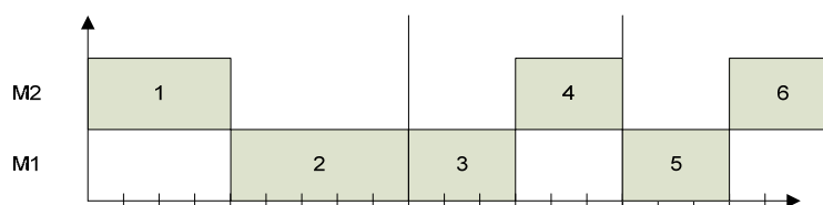
Figure 3-13. Ordonnancement réalisable
