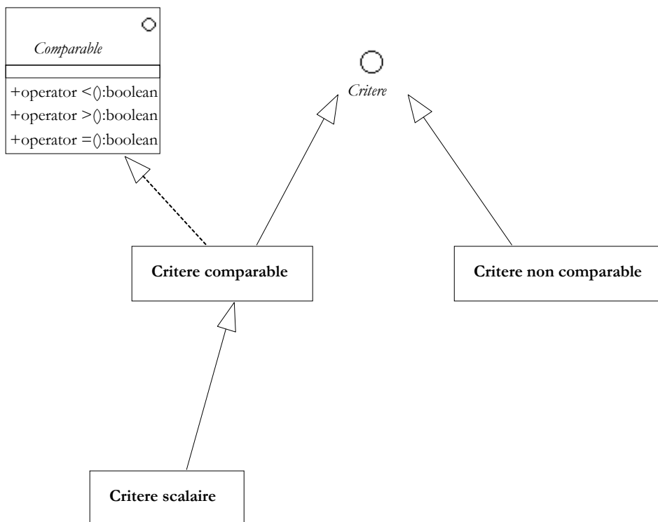
Figure 5-10. Critères
