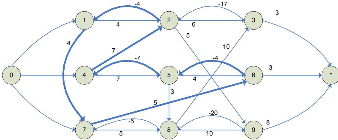
Figure 3-11. Graphe avec cycle
