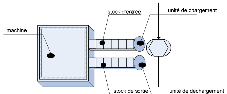
Figure 1-3. Une station
