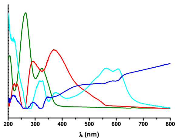
Figure 90 : Spectres des espèces pures obtenus suite à la décomposition par MCR-ALS de la matrice M\text{-FER} ( M = \text{H}^+ et \text{Ag}^+ )
