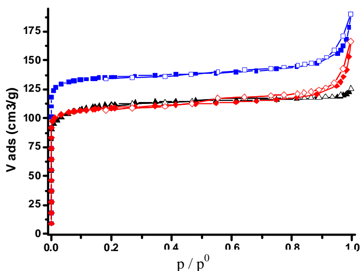
Figure 70 : Isothermes d'adsorption (symboles pleins) et de désorption (contours des symboles) de N_2 à 77 K de la mordénite (courbes bleues), de la ZSM-5 (courbes noires) et de la Ferrièreite (courbes rouges)
