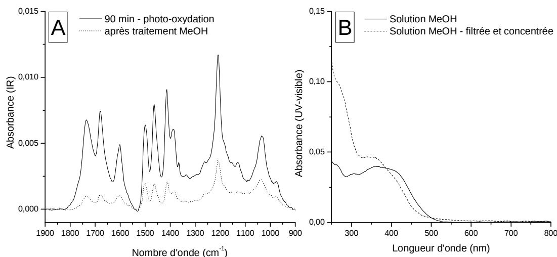
Figure 31 : (A) Spectres IR d'échantillons de MDMO-PPV photo-oxydés 90 min avant (trait plein) et après (trait pointillé) traitement méthanol. (B) Spectres UV-visible de la solution d'extraction méthanolique (B).
