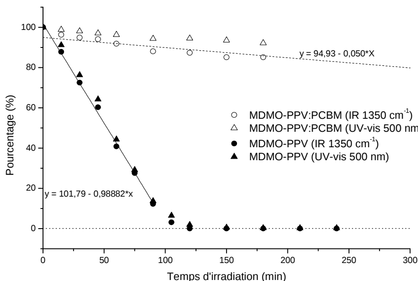
Figure 36 : Influence de la présence de PCBM sur la vitesse de dégradation du MDMO-PPV au cours de la photo-oxydation. Evolution normalisée de l'absorbance de la bande UV-visible (500 nm - \Delta ) et de la bande IR à 1352 cm -1 (Ether - \circ ) d'échantillons de MDMO-PPV (marques noires) et de MDMO-PPV:PCBM (marques blanches).
