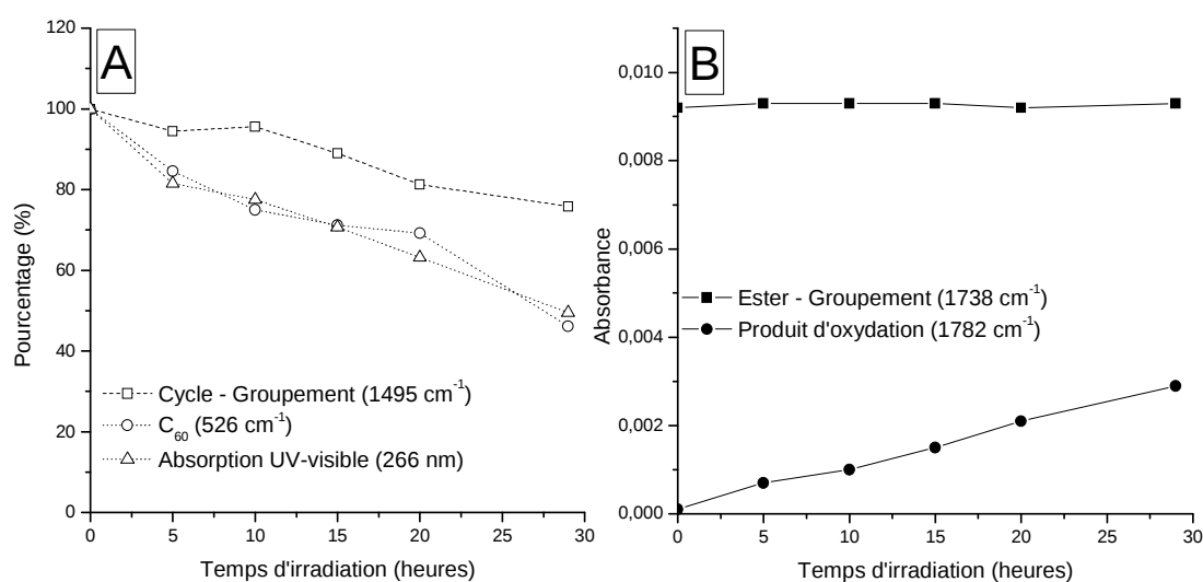
Figure 71 : Cinétique de dégradation du PCBM au cours de la photo-oxydation. (A) Décroissance normalisée de l'absorbance IR et UV-visible : 1504\text{ cm}^{-1} (Cycles Groupement - □), 526\text{ cm}^{-1} ( C_{60} - ○) et absorbance UV-visible à 266\text{ nm} (△). (B) Evolution des absorbances IR à 1782\text{ cm}^{-1} (photo-produit - ●) et 1738\text{ cm}^{-1} (Ester - ■).
