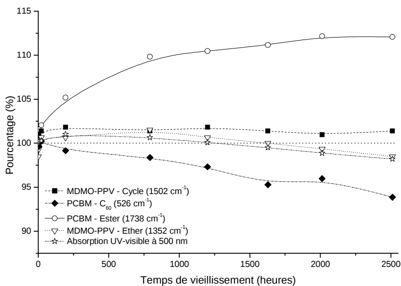
Figure 81 : Cinétique de dégradation du MDMO-PPV:PCBM au cours de la thermo-oxydation à 60°C. Evolution normalisée de l'absorbance IR et UV-visible : 1738\text{ cm}^{-1} (Ester PCBM - ○), 1502\text{ cm}^{-1} (Cycles MDMO-PPV - ■), 1352\text{ cm}^{-1} (Ether MDMO-PPV - ▽), 526\text{ cm}^{-1} ( C_{60} PCBM - ♦) et absorbance UV-visible à 500 nm (☆).
