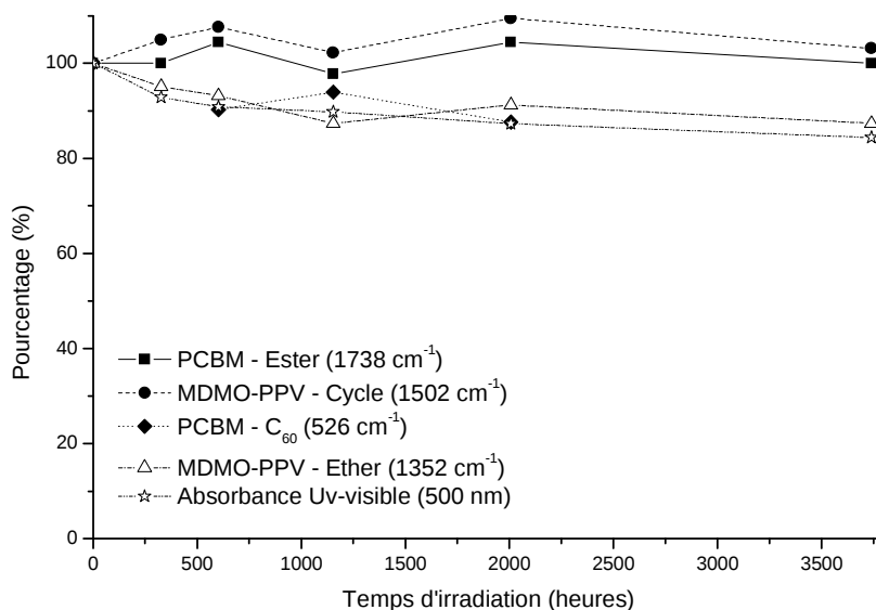
Figure 87 : Cinétique de dégradation du MDMO-PPV:PCBM au cours de la photolyse. Evolution normalisée de l'absorbance IR et UV-visible : 1738\text{ cm}^{-1} (Ester PCBM - ■), 1502\text{ cm}^{-1} (Cycles MDMO-PPV - ●), 1352\text{ cm}^{-1} (Ether MDMO-PPV - △), 526\text{ cm}^{-1} ( C_{60} PCBM - ◆) et absorbance UV-visible à 500 nm (☆).
