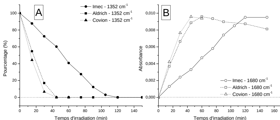
Figure 22 : Cinétiques de vieillissement de trois différents lots de MDMO-PPV. (A) Disparition de la fonction éther et (B) évolution de l'absorbance à 1680 cm -1 au cours de la photo-oxydation pour les polymères « Imec » (rond), « Aldrich » (carré) et « Covion » (triangle).
