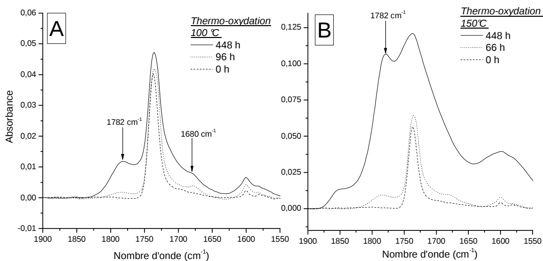
Figure 83 : Evolution du spectre IR d'échantillon de MDMO-PPV:PCBM au cours des vieillissement thermique à 100 (A) et 150°C (B). Zone spectrale comprise entre 1900 et 1550 cm -1 pour des temps de dégradation compris entre 0 et 448 heures.
