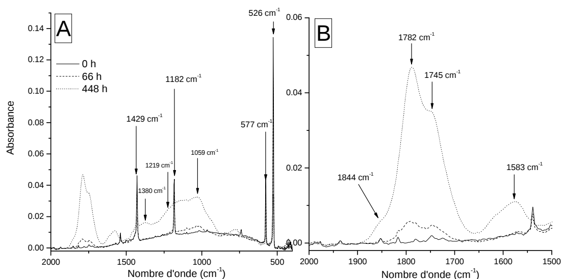
Figure 66 : Evolution du spectre IR du fullerène au cours de la thermo-oxydation à 150 °C. Spectres directs dans les zones 2000 – 400 \text{cm}^{-1} (A) et 2000 – 1500 \text{cm}^{-1} (B) pour des temps de vieillissement compris entre 0 et 448 heures.
