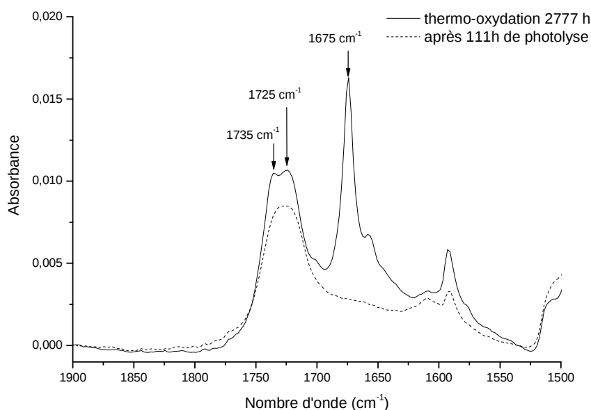
Figure 53 : Spectres IR entre 1900 et 1500\text{ cm}^{-1} d'échantillons de Oct-OPV5 soumis à 2777\text{h} de thermo-oxydation (ligne pleine) puis soumis à 111\text{h} de photolyse (ligne pointillée).
