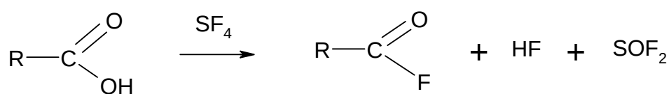
Schéma 17 : réaction de dérivation chimique des acides carboxyliques en fluorures d'acides
