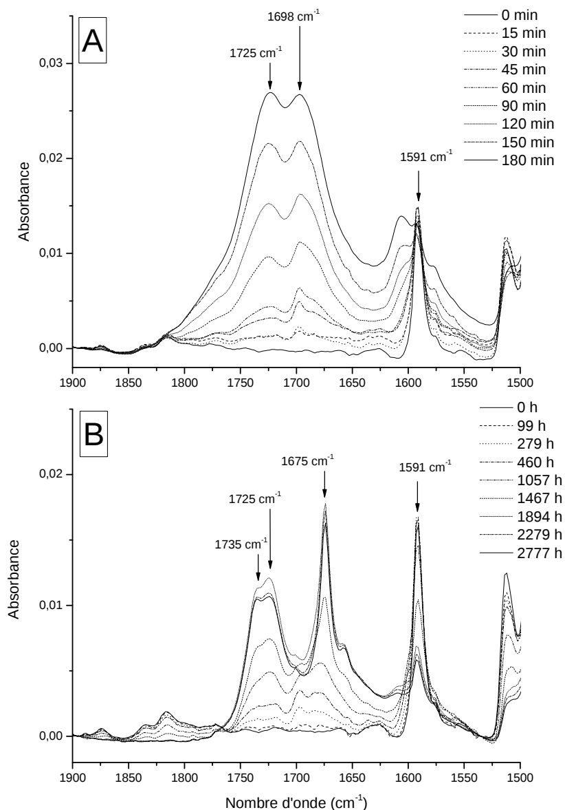
Figure 50 : Evolution du spectre IR de l'Ooct-OPV5 dans la zone des produits carbonylés (1900 – 1500 cm⁻¹) au cours de la photo-oxydation (A) et de la thermo-oxydation à 60°C (B).
