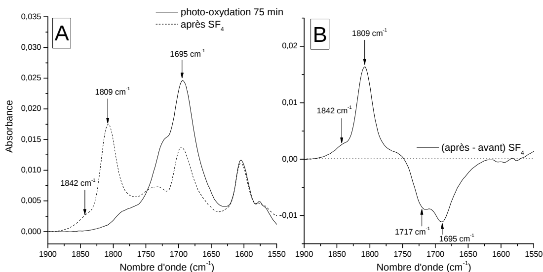
Figure 62 : Spectres IR entre 1900 et 1500 \text{cm}^{-1} d'échantillons de PPV photo-oxydés : (A) avant (ligne pleine) et après (ligne pointillée) traitement SF 4 et (B) spectre de différence (après – avant).
