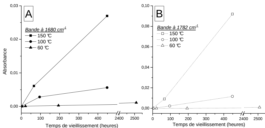
Figure 84 : Cinétique de dégradation du MDMO-PPV:PCBM au cours de thermo-oxydation à 60 (Δ), 100 (○) et 150 °C (□). Evolution de l'absorbance correspondant aux produits d'oxydation caractéristiques du MDMO-PPV à 1680 cm -1 (A) et du PCBM à 1782 cm -1 (B).
