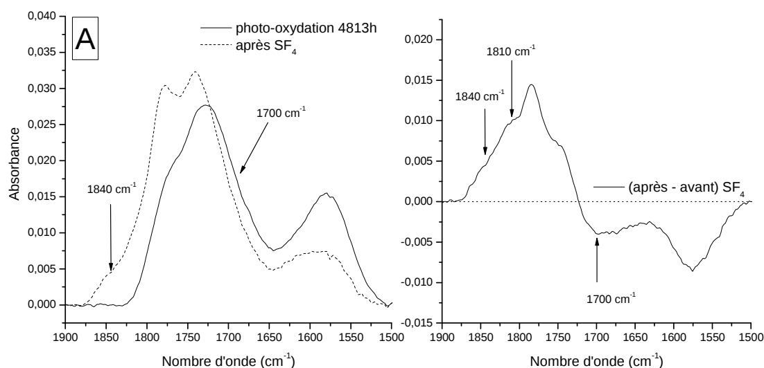
Figure 68 : Spectres IR entre 1900 et 1500 \text{cm}^{-1} d'échantillons de \text{C}_{60} photo-oxydés : (A) avant (ligne pleine) et après (ligne pointillée) traitement \text{SF}_4 et (B) spectre de différence (après – avant).
