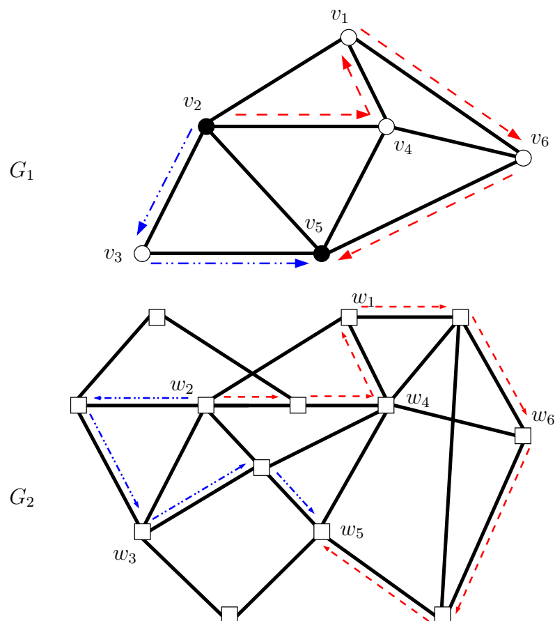
FIG. 7.6 – Solution réalisable
