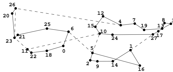
FIG. 3.24 – Point fractionnaire avant r  duction
