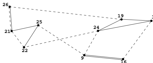
FIG. 3.25 – Point fractionnaire avec r  duction    l'aide de l'op  ration \theta_2
