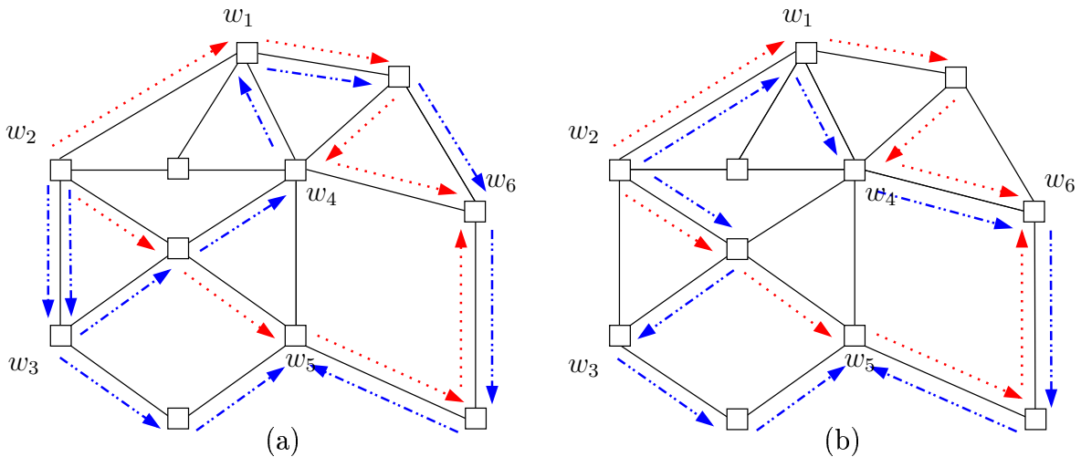
FIG. 7.4 – Solutions non réalisables du problème
