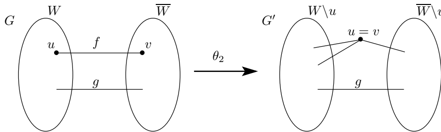
FIG. 3.21 – Opération \theta_2
