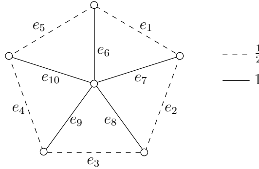
FIG. 3.16 – Un point extrême fractionnaire
