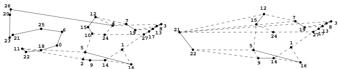
FIG. 3.30 – Instance à 28 sommets et 46 arêtes
