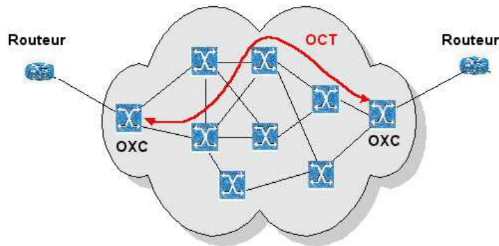
FIG. 2.2 – OTN
