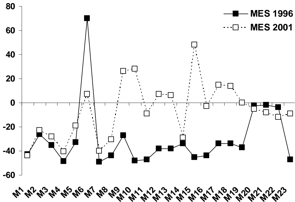
Figure A-1 : Erreurs sur les flux de Nitrate et de MES estimées par 23 méthodes de calculs à partir d'une simulation de surveillance mensuelle pour deux années contrastées : 1996 et 2001
