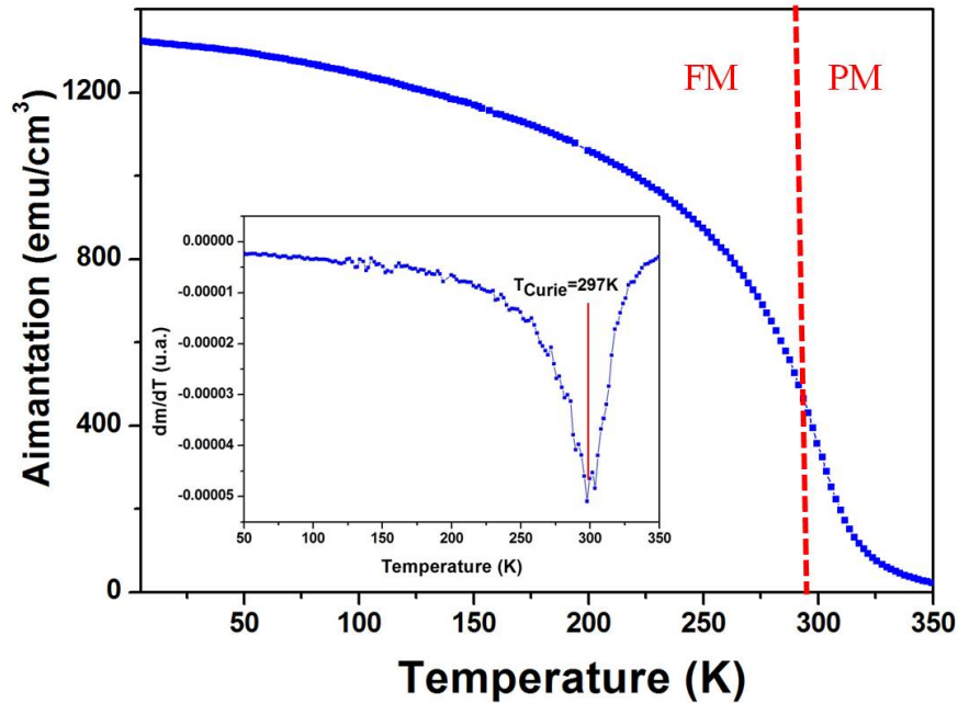
FIGURE 3.2.12 – Dépendance en température de l'aimantation à saturation M_{sat} d'une couche de Mn_5Ge_3 (40 nm)/Ge(111) mesurée par SQUID avec un champ magnétique de 1 T appliqué dans le plan de la couche. La droite rouge en pointillé marque la transition d'un état ferromagnétique (FIM) à un état paramagnétique (MM). En insert, la dérivée de l'aimantation en fonction de la température possède un pic à 297 K.
