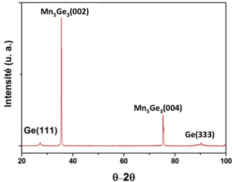
FIGURE 3.2.6 – Spectre de diffraction \vartheta - 2\vartheta d'une couche de \text{Mn}_5\text{Ge}_3 élaborée par SPE. Indexation des pics \text{Mn}_5\text{Ge}_3 (002) et (004).
