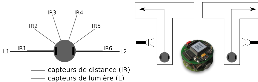
FIGURE 4.7 – À gauche, schéma des capteurs utilisés avec le robot mobile Khepera dans l'expérience originale. À droite, les deux cas de tests de l'expérience reproduite, ainsi que le robot Khepera.
