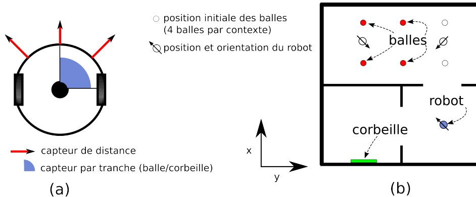
FIGURE 5.5 – (a) Présentation de la tâche de collecte de balles. En plus de ses 3 capteurs de distance, le robot est équipé de 2 capteurs détectant les balles et de 2 capteurs détectant la corbeille. Le champ de détection des capteurs droits est indiqué sur la figure. Celui des capteurs gauches est symétrique. Un réseau de neurones contrôle les vitesses des deux roues motorisées, ainsi qu’un moteur de ramassage de balles. (b) Arène où le robot évolue. Les 6 positions possibles des balles et quelques positions et orientations initiales du robot sont schématisées.
