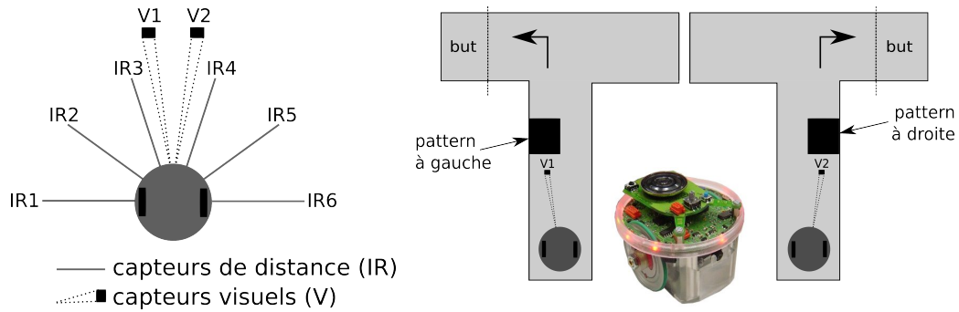
FIGURE 4.8 – A gauche, schéma des capteurs utilisés avec le robot mobile e-puck. A droite, les deux cas de tests de notre dispositif expérimental, ainsi que le robot e-puck.
