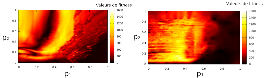
FIGURE 4.19 – À gauche, paysage de fitness (distance parcourue en millimètres) exhaustif obtenu en simulation pour l'application de marche quadrupède. À droite, interpolation du paysage de fitness en réalité basée sur environ 5500 expériences de transfert. Ces expériences ont essentiellement été menées dans la zone p_1 < 0.6 : pour des valeurs plus élevées de p_1 le robot se recroqueville sur lui-même et ne bouge pas efficacement, d'où une région assez uniforme de fitness basses.
