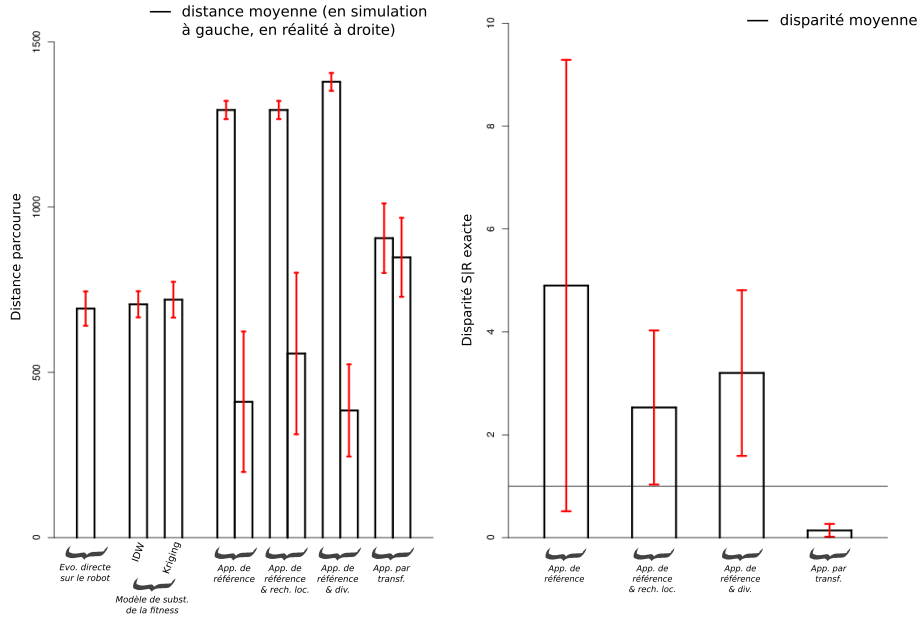
FIGURE 4.18 – Résultats obtenus dans l'application de marche quadrupède : distance parcourue en simulation et en réalité (mm, à gauche) et valeurs exactes de disparité (à droite) des meilleures solutions trouvées avec chaque approche. Moyennes et écarts types sont calculés sur 10 répétitions, sauf pour l'évolution directe sur le robot qui n'a été répétée que 3 fois. Les barres d'erreur indique une unité d'écart-type.
