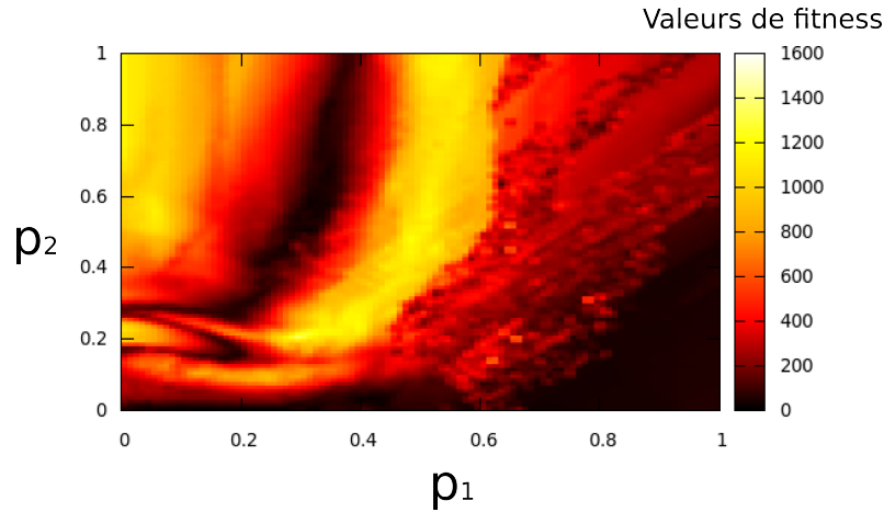
FIGURE 4.15 – Paysage exhaustif de fitness en simulation pour l'application de marche quadrupède : distance parcourue en simulation associée à chaque couple de paramètres (p_1, p_2) (environ 2.6 \cdot 10^5 contrôleurs possibles). Les valeurs des paramètres de contrôle p_1 et p_2 sont respectivement indiquées suivant l'axe x et l'axe y. La couleur représente l'intensité de la valeur de fitness.
