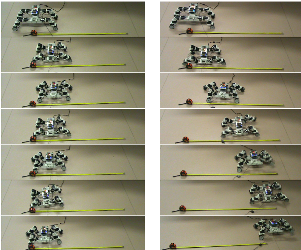
FIGURE 4.20 – A gauche, comportement typique évolué avec l’approche de référence : le comportement est rendu complètement inefficace à cause du glissement des pattes sur le sol. A droite, comportement typique obtenu avec l’approche par transférabilité : le robot effectue une marche quadrupède efficace et similaire au comportement observé en simulation.
