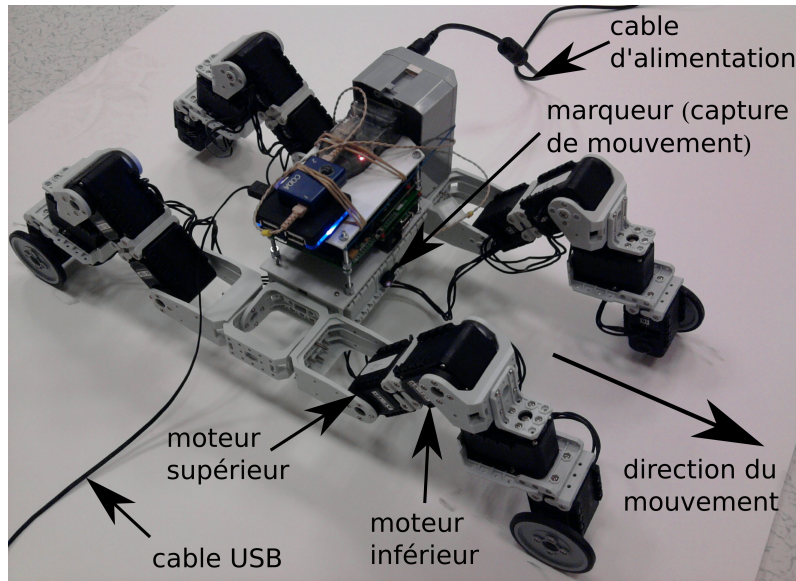
FIGURE 4.14 – Robot quadrupède utilisé dans notre dispositif expérimental.
