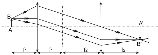
FIG. 10.3 – Schéma d'un système afocal.
