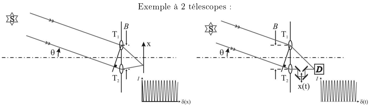
FIG. 1.7 – Schéma de principe de l'expérience des fentes d'Young analysant une source ponctuelle S dans la direction \theta . T_1 et T_2 sont les deux trous, B la distance entre eux appelée base, \delta est la différence de marche entre les champs qui arrivent sur les ouvertures. A gauche, on montre l'exemple d'une modulation spatiale où le phénomène des franges d'interférences est vu sur un écran ou un détecteur multipixel. A droite, on peut voir l'exemple d'une modulation temporelle où la visualisation du phénomène de franges d'interférences se fait par une modulation temporelle d'un chemin optique.
