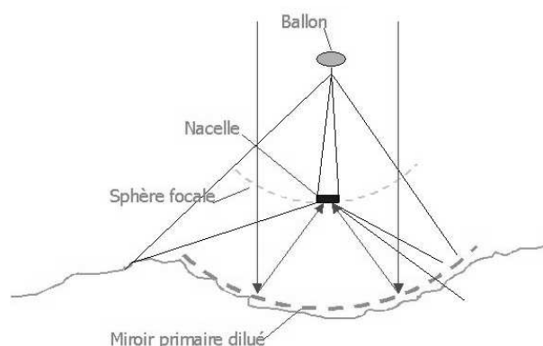
FIG. 2.7 – Schéma de principe du projet Carlina : la pupille diluée se trouve au sol, dans une doline par exemple. La pupille densifiée et le plan image se situent au-dessus, dans une nacelle portée par un ballon ou un cerf-volant
