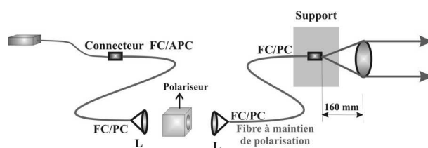
FIG. 5.3 – Le simulateur d'étoile.
