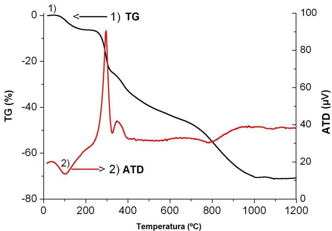
Figura 4.1- TG/ATD do pó precursor BaCeO_{3-\delta} .
