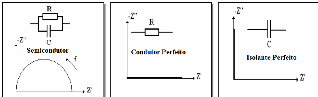
Figura 2.3 - Diagramas de Nyquist para diferentes tipos de materiais.
