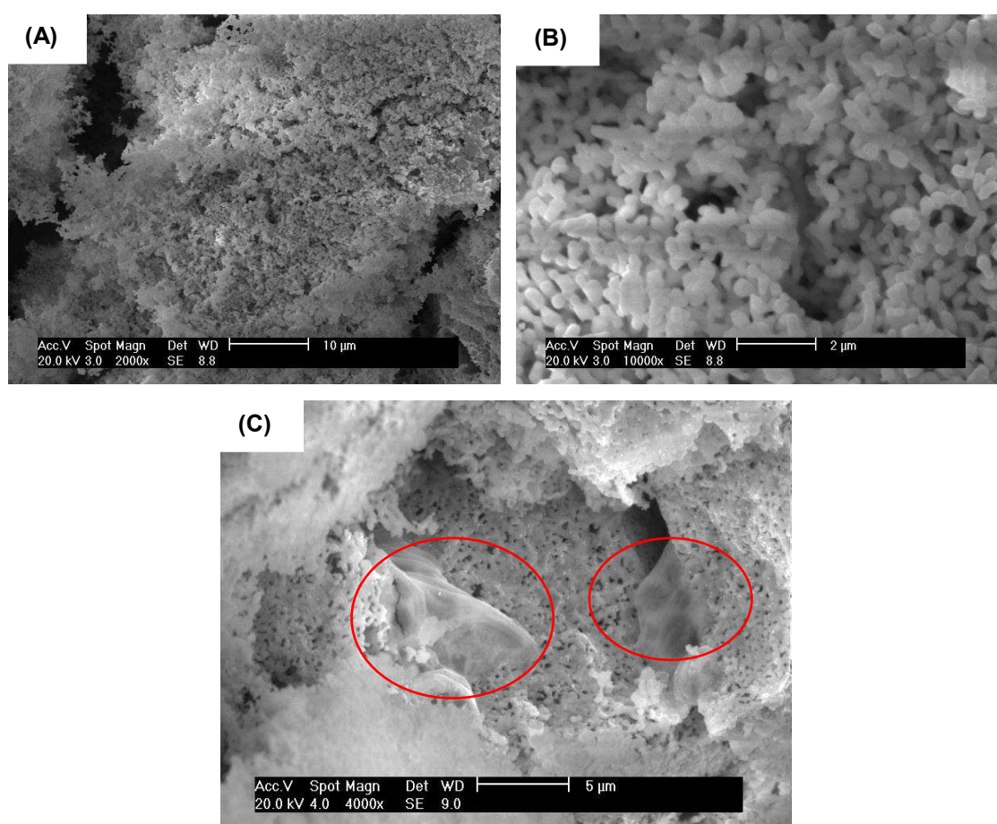
Figura 4.2 - Microscopias eletrônicas de varredura do pó cerâmico BaCeO_{3-\delta} obtido através do método de complexação EDTA – Citrato modificado. Ampliação de (A) 2000x, (B) 10000x e (C) 4000x.
