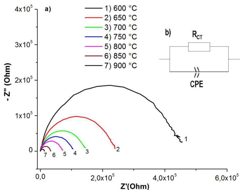
Figura 4.6 – a) Representação de Nyquist de impedâncias elétricas obtidas para BaCeO_3 na faixa de temperatura de 600^\circ\text{C} - 900^\circ\text{C} , e b) modelo de circuito equivalente com os componentes R e CPE.
