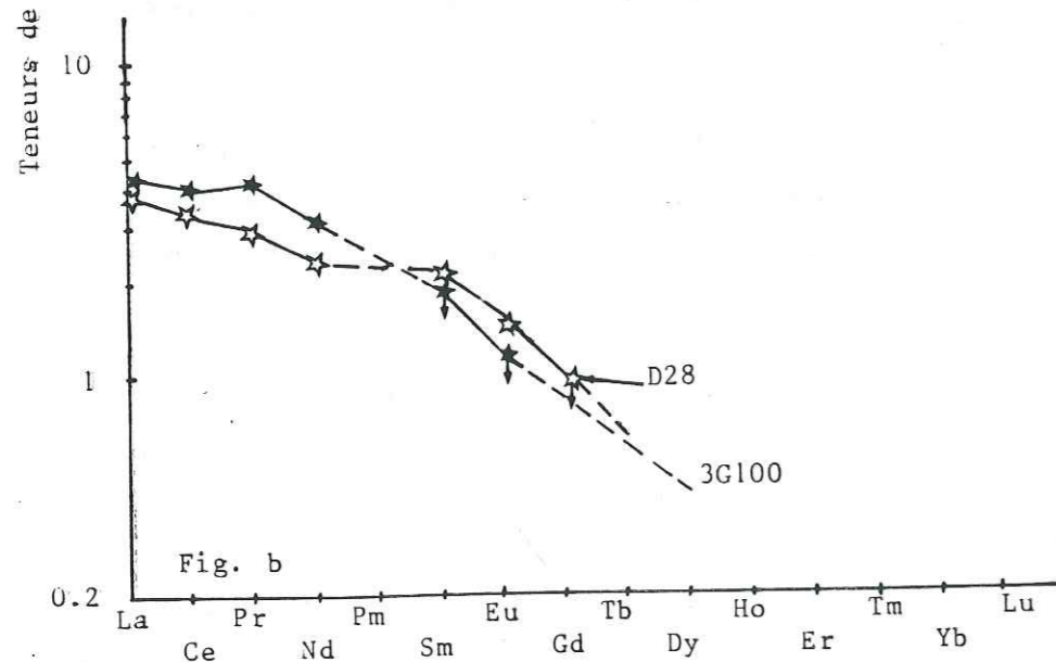
Figure 41 : Profils de répartition des T.R. des carbonates non filoniens (C3,C4) de Bleïda (normalisés par rapport aux chondrites) : a = C3, b = C4
