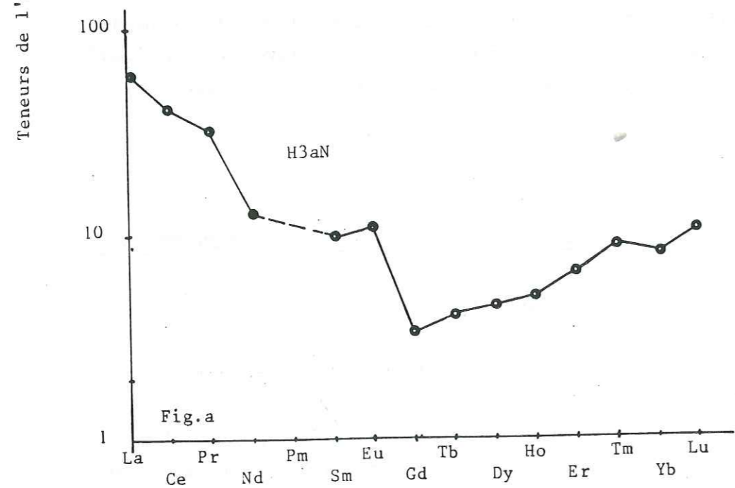
Figure 40 : Profils de répartition des T.R des carbonates filoniens C2 de Bleida normalisés par rapport aux chondrites: a= bord du filon , b = coeur du filon
