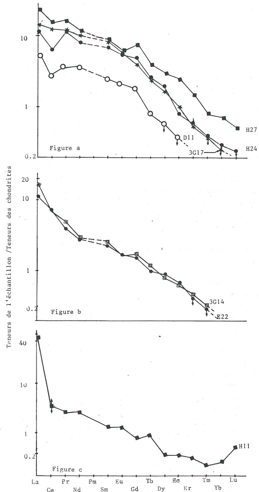
Figure 36 : Profils de répartition des T.R. des carbonates filoniens C1 de Bleida normalisés par rapport aux chondrites
