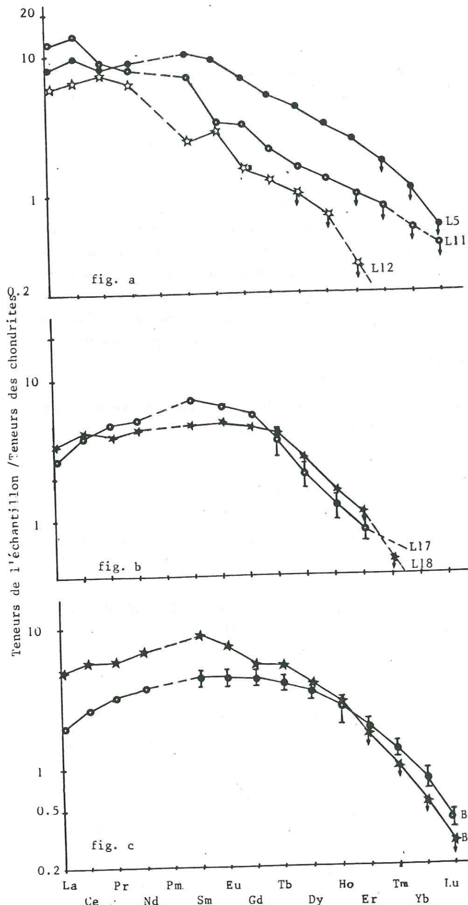
Figure 37 : Profils de répartition des T.R des listvénites : a = échantillon d'Elguir (●), de Mechoui (☆), de Mokhazni (○) b = Bou-Azzer Est; c = Arouli N'Azzougar
