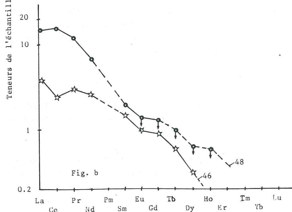
Figure 38 : Profils de répartition des T.R. des échantillons d'Ambed normalisés aux chondrites : a = formation d'Ambed, b = cerne de talc (46) et calcite en gros cristaux près des serpentines
