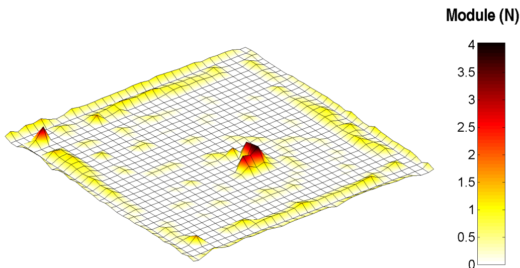
FIGURE 4.14 – Cartographie 3D des amplitudes des forces \mathbf{F}^{\text{d}} identifiées sur la plaque mince en aluminium, après déconvolution. La fréquence d'étude est f = 1404\text{Hz} .
