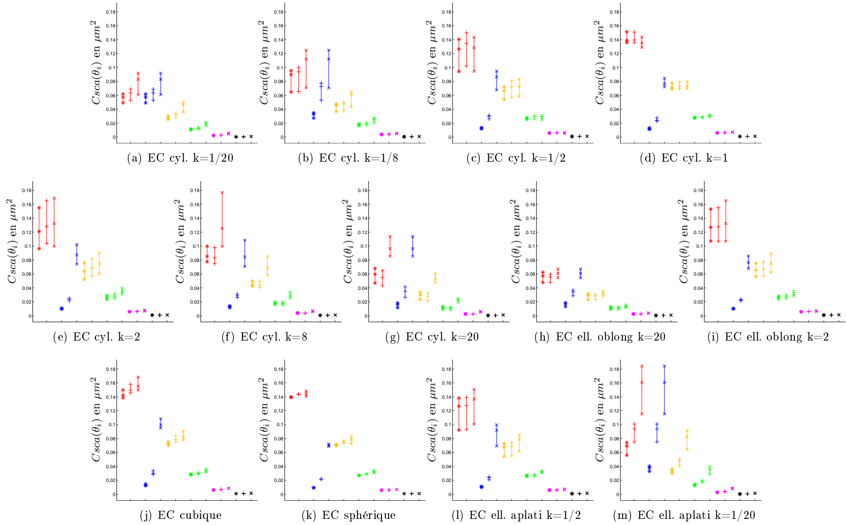
FIG. 3.18 – Distributions en barres de valeurs de C_{sca} non normalisées, pour les agrégats de PV_{EC} = 300 , en maille hexagonale compacte et pour le couple optique (ZnS, HeNe). Légende des couleurs : EC pleine, EC creuse, EC remplie à 75%, EC remplie à 50%, EC remplie à 25%, EC remplie à 10%. Légende des marqueurs sur l'étalement : \star R_{pp} = 10 nm, + R_{pp} = 15 nm, \times R_{pp} = 30 nm
