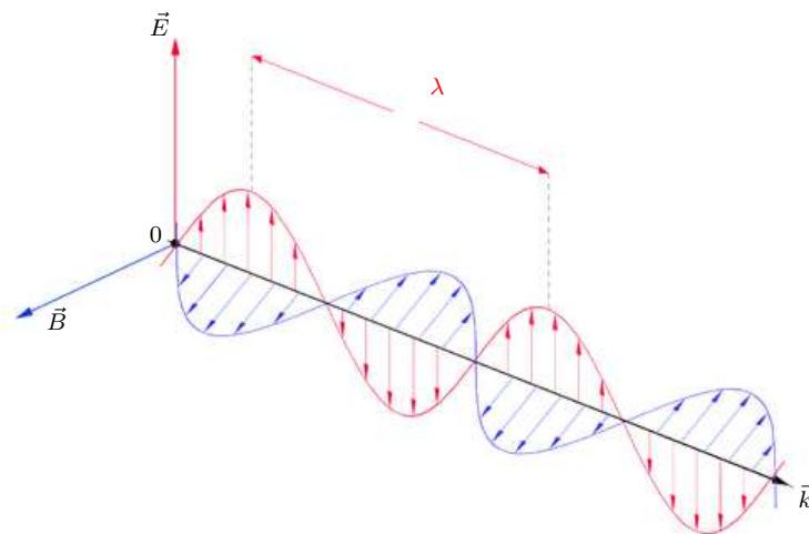
FIG. 2.5 – Schéma d'une onde électromagnétique
