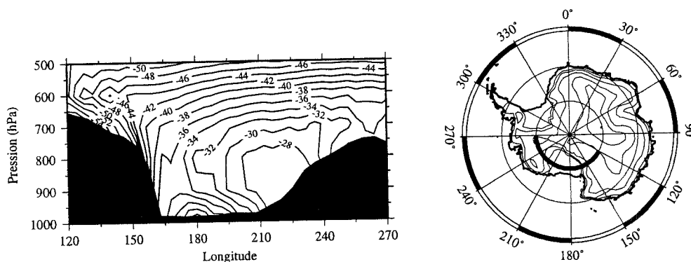
Figure 1.3: Les températures atmosphériques (en °C) en Juillet dans une coupe longitudinale/altitude à 80°S sur une longueur de 2900 km. Le trait épais dans la petite carte à droite indique le tracé de la coupe. À gauche se trouve l'Antarctique de l'Est. La plate-forme glaciaire de Ross est située au centre, et l'Antarctique de l'Ouest à droite. Le niveau de pression 500 hPa correspond à une altitude d'environ 5 km. On voit une inversion de surface à l'intérieur de la calotte, mais aussi sur la plate-forme glaciaire même. Simulation LMDz.
