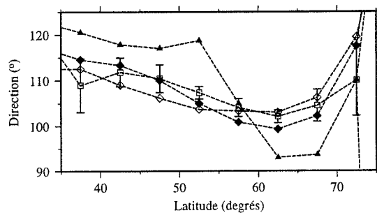
Figure 5.9: Direction des cyclones (en ^{\circ} ). Une direction de 0^{\circ} signifie une propagation vers le Nord ; 90^{\circ} signifie une propagation vers l'Est, et 180^{\circ} , vers le Sud. La direction habituelle des cyclones est, grossièrement, ESE. Carrés grisés : CEPMMT ; losanges noirs : AA0 ; losanges transparents : REG ; triangles noirs : FORT.
