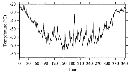
Figure 4.8: T_s (en °C) à Dôme C en 1990. Mesures d'AWS.
