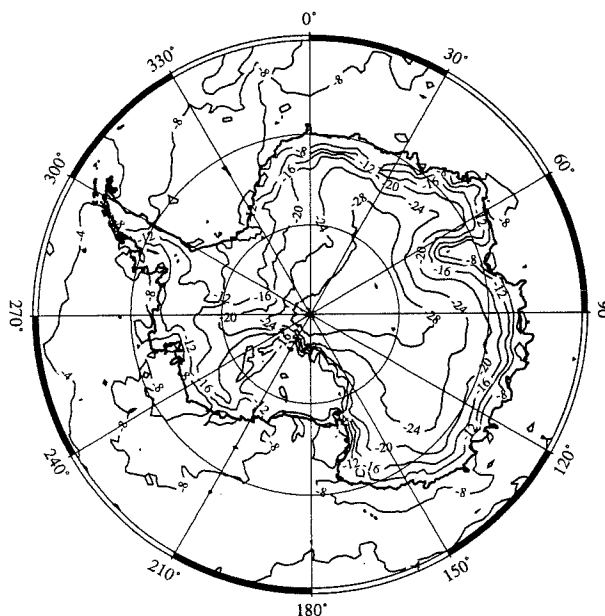
Figure 4.6: Mesures de T_s (en ^{\circ}\text{C} ) pour le mois de Janvier 1979 [Comiso, 1994].
