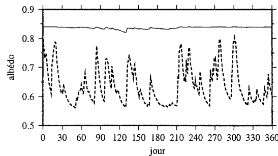
Figure 3.14: Albédo simulé à Dôme C pour 1990 après modification de la formulation du vieillissement de la neige (trait plein), et albédo obtenu pour les mêmes températures et précipitations avec l'ancienne formulation (trait interrompu).
