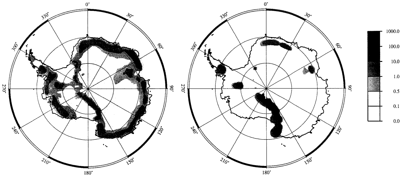
Figure 3.6: A gauche : z_{0,oro} en m selon la formulation originale de LMDz ; à droite : z_{0,oro} en m selon la formulation du CEPMMT.
