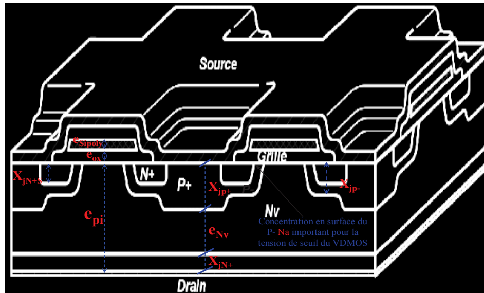
Figure III.3. Structure finale du VDMOS en 3D.
