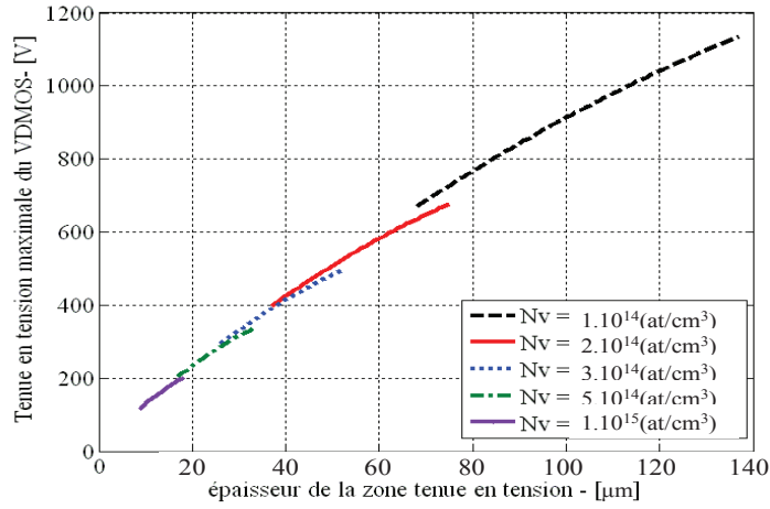
Figure A3.2. Tenue en tension du VDMOS en fonction de l'épaisseur et de la concentration de la zone tenue en tension.
