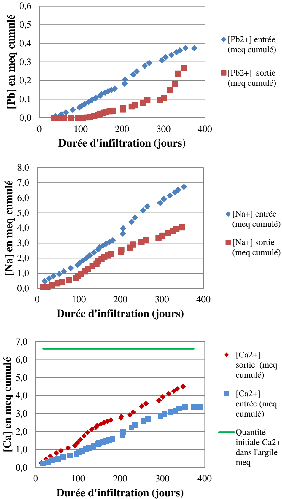
Figure 106 Concentrations des cations \text{Pb}^{2+} , \text{Na}^+ et \text{Ca}^{2+} dosés en solution (en meq cumulé) en entrée et à la sortie des cellules œdométriques Le trait vert continu correspond à la quantité initiale de Ca dans la galette d'argile
