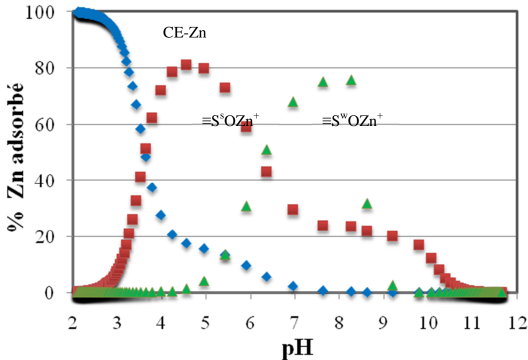
Figure 57 Contribution des différents mécanismes d'adsorption du zinc en fonction du pH dans la montmorillonite Ca-SWy2 ; \diamond : % du Zn adsorbé par échange cationique (CE-Zn), \blacktriangle % du Zn adsorbé par les sites faibles ( \equiv S^wOZn^+ ) ; \blacksquare : % du Zn adsorbé par les sites forts ( \equiv S^sOZn^+ )
