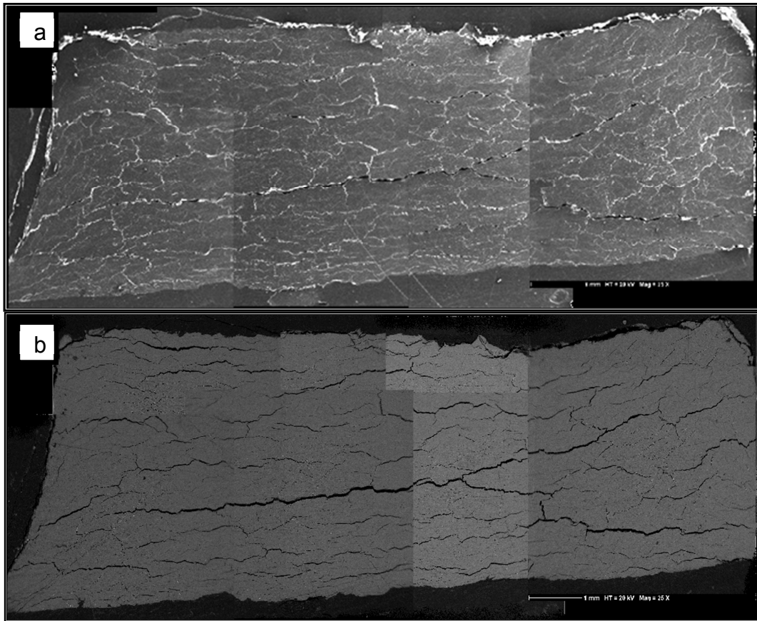
Figure 92 Clichés MEB d'un échantillon Ca-SWy2 percolé avec Pb(NO_3)_2 réalisés à une tension de 20 kV ; (a) mode électrons secondaires et (b) mode électrons rétrodiffusés
