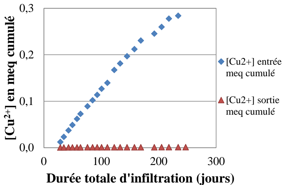
Figure 121 : Concentrations du cuivre en meq cumulé en entrée et à la sortie de l'œdomètre en fonction de la durée d'infiltration (jours)
