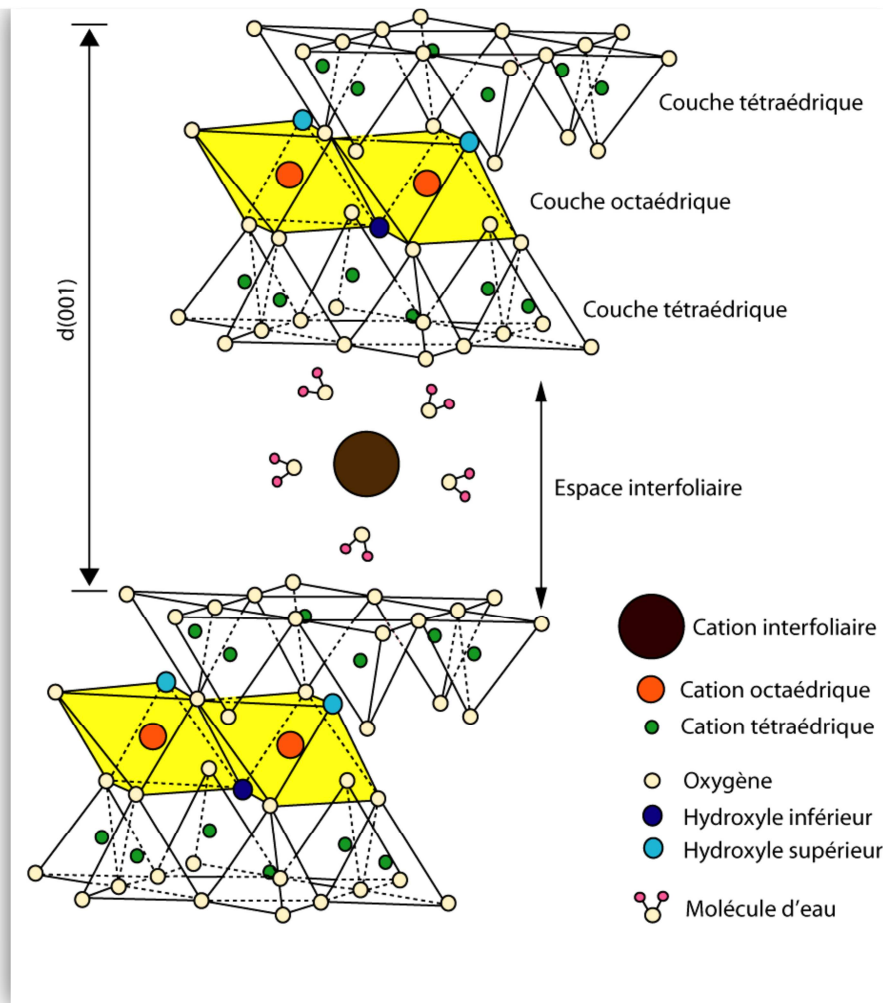
Figure 5 Représentation schématique de la structure d'une montmorillonite (d'après Grim, 1968)
