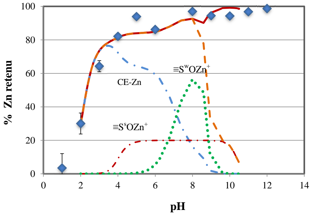
Figure 54 % du zinc retenu dans Na-SWy2 en fonction du pH. \blacklozenge : Données expérimentales. Trait rouge continu : le modèle corrigé présentant le % de Zn retenu ; trait orange interrompu : % Zn adsorbé dans l'argile ; trait bleu interrompu : % du Zn adsorbé par échange cationique (CE-Zn) ; trait vert pointillé : % du Zn adsorbé par les sites faibles ( S^wOZn^+ ) ; trait rouge interrompu : % du Zn adsorbé par les sites forts ( S^sOZn^+ )
