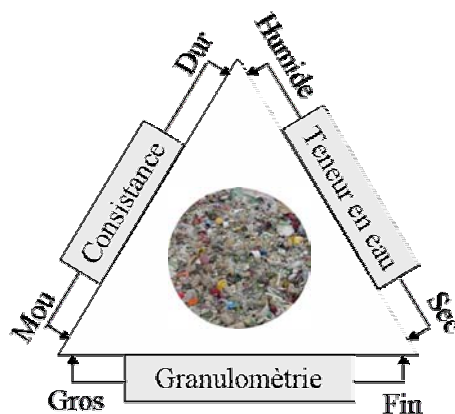
Figure 2.16 Diagramme ternaire applicable au compactage d'après Onyx (2000)
