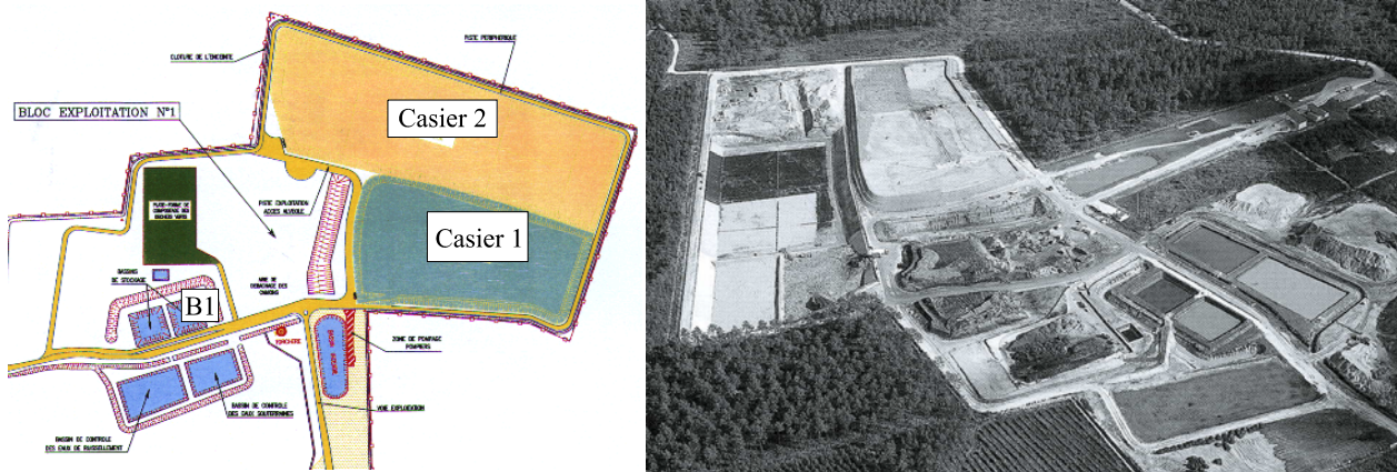
Figure 5.7 (a) Schéma général du CSD de Lapouyade avant construction du casier n°3 (b) Photographie aérienne du site (casier 1 couvert, casier 2 en cours d'exploitation)
