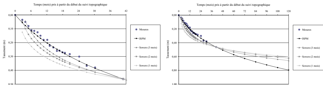
Figure 7.12 (a) Corrélation des tassements modélisés en fonction de t_m - t_m^0 à partir des modèles ISPM et Sowers avec les valeurs de terrain (calage à t_m^{ult} - t_m^0 = 40,90 mois) (b) Prédiction des tassements à 10 ans avec les modèles ISPM et Sowers (Site de Lyndhurst, zone 'Control')
