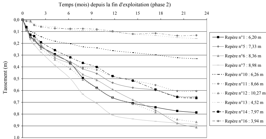
Figure 6.33 Evolution du tassement de la colonne de déchet 2 supérieure en fonction de [t - (t_c)_{Phase 2}] (CSD de Chatuzange, alvéole A''B)
