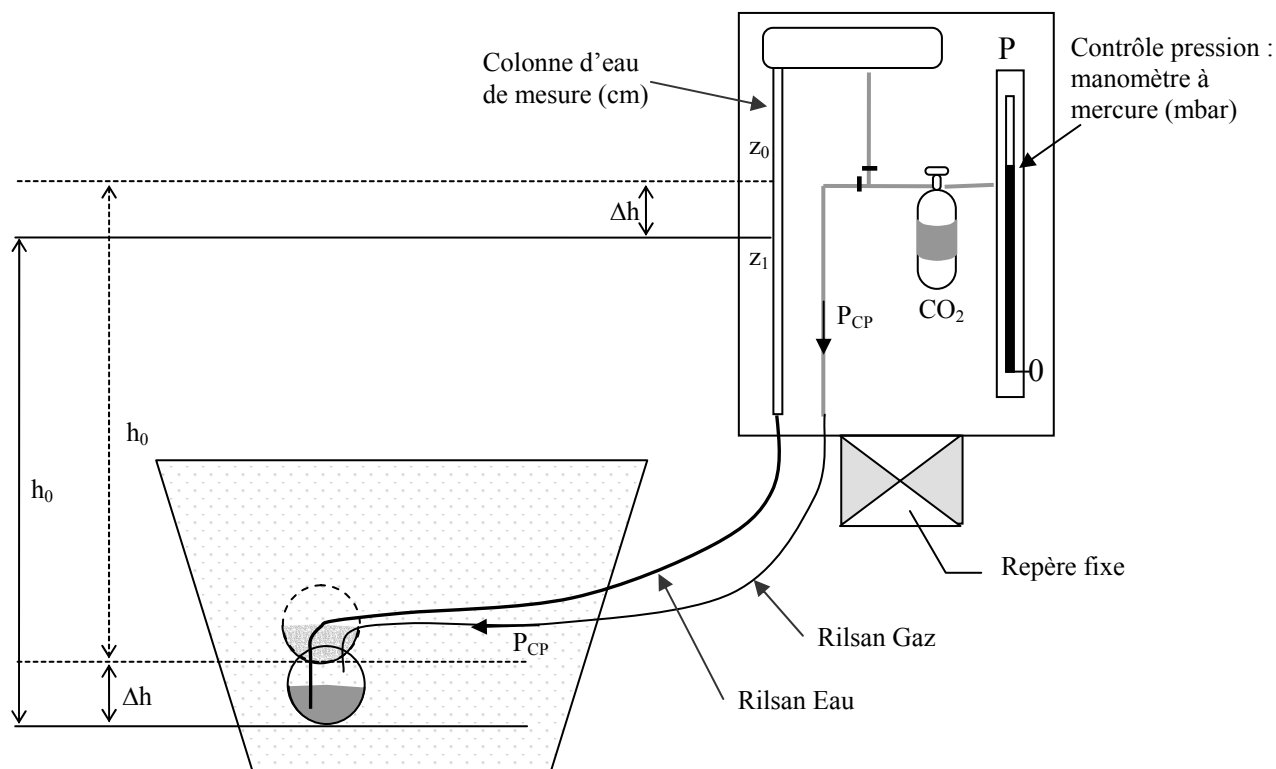
Figure 5.33 Principe de fonctionnement du tassomètre LCPC (Thomas, 2000)
