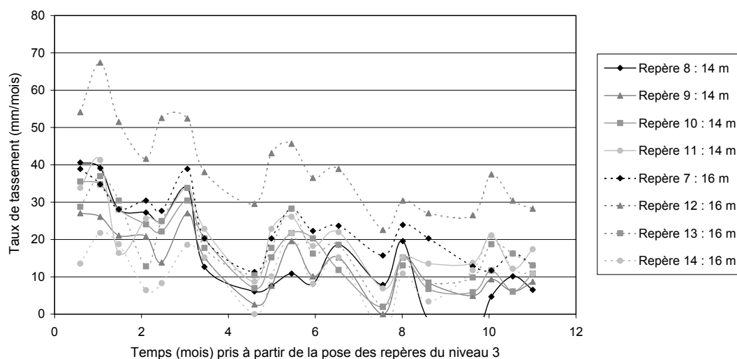
Figure 10.11 Evolution des taux de tassement en fonction de t - t_m^0 (Meruelo, niveau 3)
