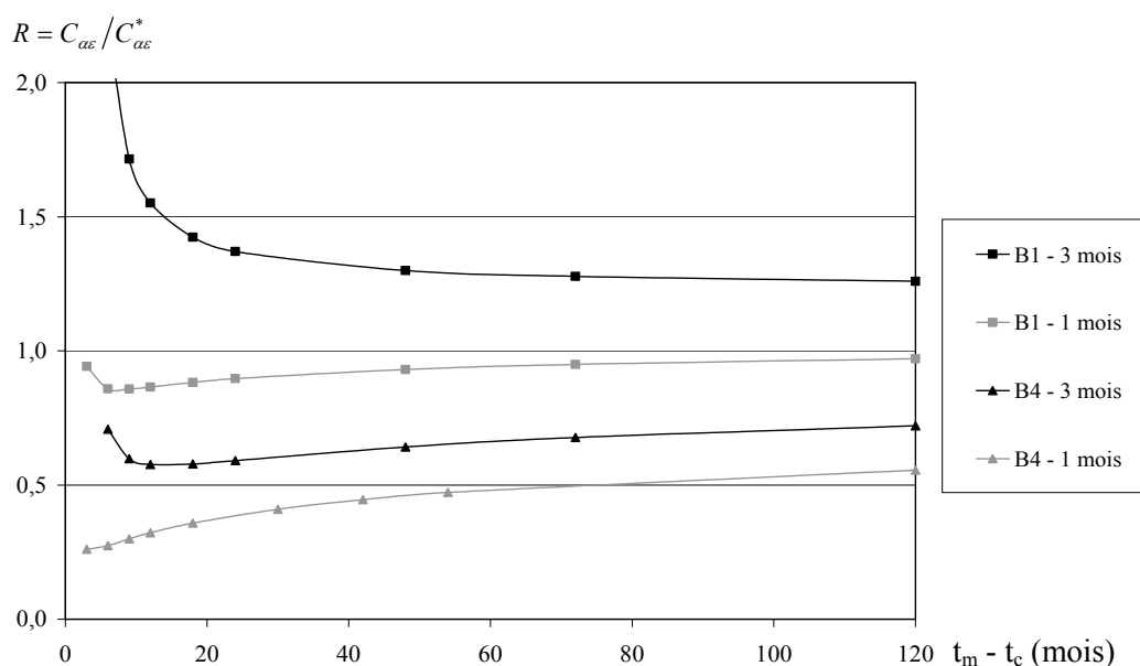
Figure 7.7 Evolution du rapport R = C_{\alpha\epsilon} / C_{\alpha\epsilon}^* en fonction de la valeur de (t_m - t_c) = 1 mois ou 3 mois (colonnes B1 et B4 ; nh_0 = 24 m)
