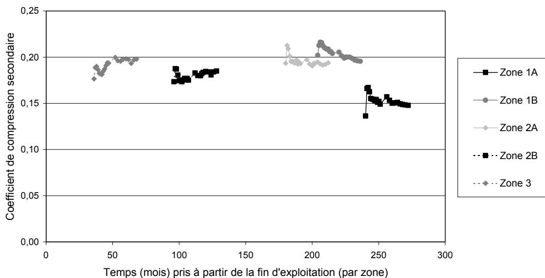
Figure 6.18 Evolution de C_{ae}^* en fonction du temps t - t_c (CSD de Montréal)
