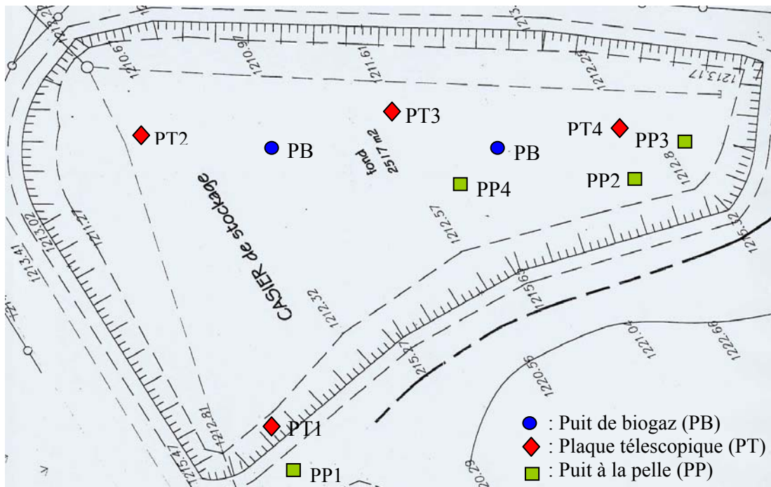
Figure 3.1 Implantation des puits à la pelle (4) et des plaques télescopiques (4)
