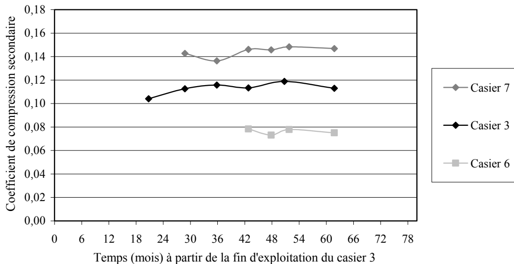
Figure 6.20 Evolution des coefficients C_{ae}^* en fonction de [t_m - (t_c)_{cell3}] (Novellara, casiers 3, 7 et 6)
