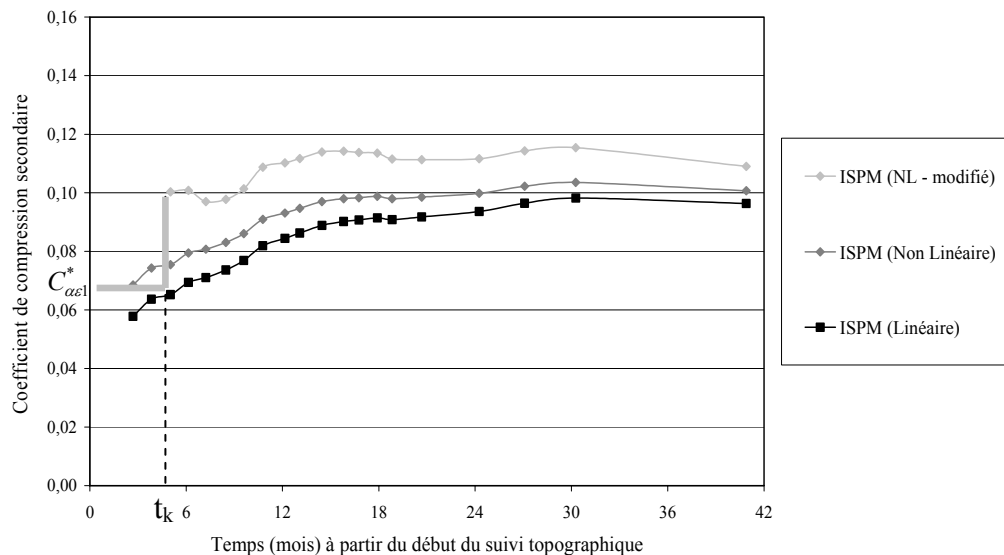
Figure 3.36 Evolution de C_{ac}^* en fonction du temps à partir de 3 hypothèses de modélisation (linéaire, non linéaire à 1 coefficient C_{ac}^* et non linéaire à 2 coefficients C_{ac1}^* et C_{ac2}^* (Site de Lyndhurst, zone 'Control')
