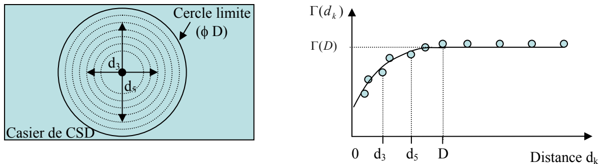
Figure 9.5 Schéma de principe de la méthode du variogramme circulaire
