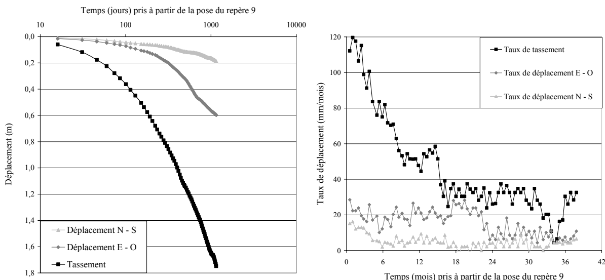
Figure 10.15 (a) Evolution des déplacements ( \Delta u , \Delta v , \Delta w ) du repère 9 en fonction du logarithme du temps (b) Evolution des taux de déplacement en fonction du temps (Site de Hong-Kong)
