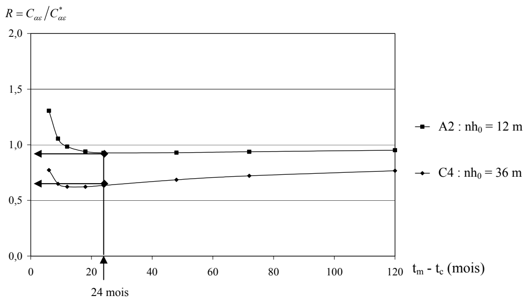
Figure 7.4 Evolution du rapport R = C_{\alpha\epsilon} / C_{\alpha\epsilon}^* en fonction de t_m - t_c (colonnes A2 et C4 : nh_0/t_c = 1 m /mois ; t_1 = t_c + 3 mois)
