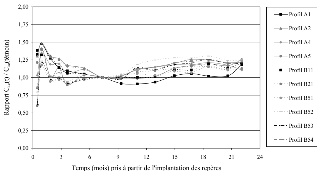
Figure 8.18 Evolution de C_{ac}^*(t)/C_{ac}^* (05/07/2002) en fonction du temps - modélisation non linéaire à 20 couches (NL20) (CSD de Lons-le-Saunier, tous profils sauf A3)
