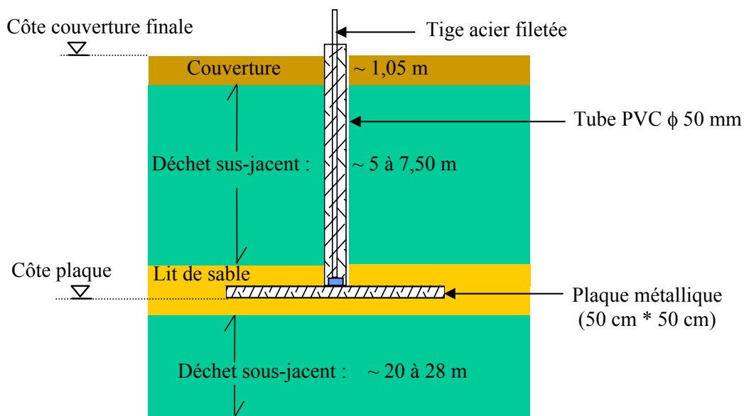
Figure 5.42 Schéma de principe des plaques et tiges télescopiques (Site de Chatuzange)
