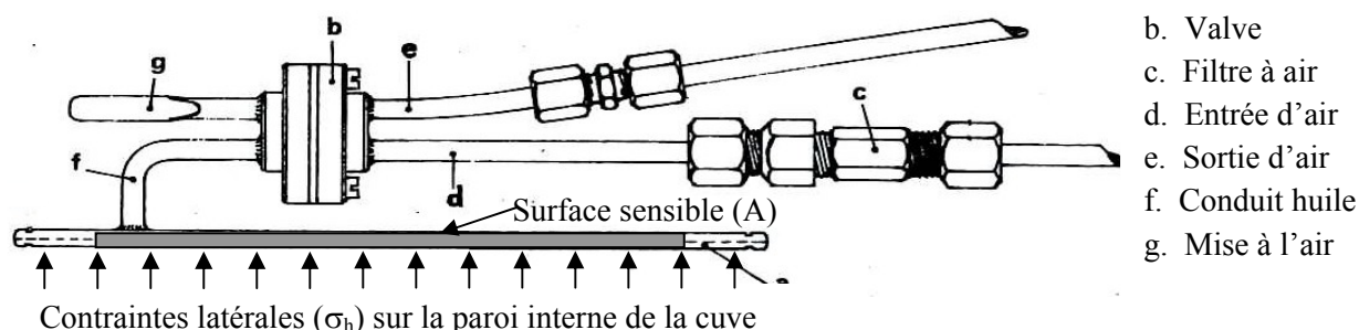
Figure 4.16 Schéma de principe des cellules de contraintes 'Glötz'
