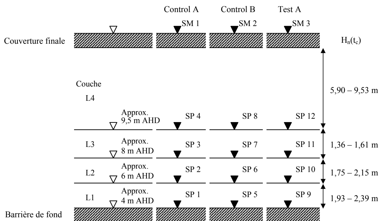
Figure 8.12 Schéma d'implantation des plaques enterrées (SP) et des plaques de surface (SM) repris à partir de Yuen (1999) (Site de Lyndhurst, zones témoin et recirculée)
