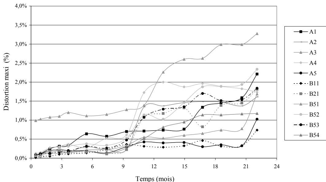
Figure 9.13 Evolution de l'indice de distorsion en fonction du temps (CSD de Lons-le-Saunier)
