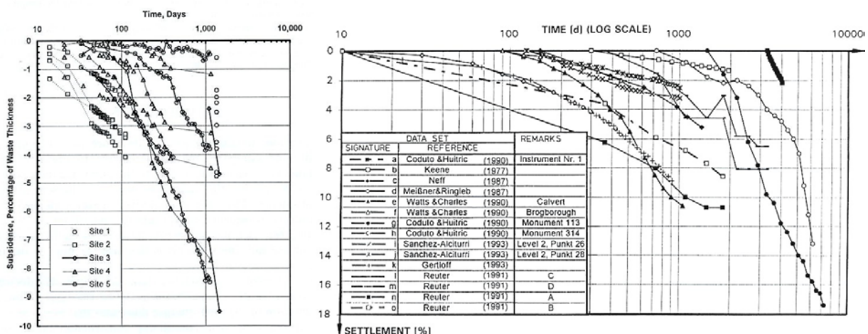
Figure 5.23 Evolution du tassement relatif (de surface) en fonction du temps sur échelle semi-logarithmique (a) 5 sites étudiés par Spikula (1997) (b) 15 sites répertoriés par König et al. (1996) reproduit par Kockel et al. (1997)
