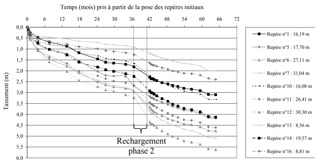
Figure 6.28 Evolution du tassement total de la colonne de déchet 1 inférieure en fonction du temps [t - (t_m^0)_{Phase 1}] (CSD de Chatuzange, alvéole A''B)
