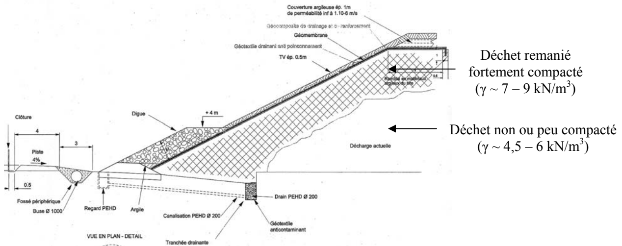
Figure 5.56 Schéma de réaménagement du talus ouest du site de Cognac (Profil P3, hauteur en tête \cong 14 \text{ m} )
