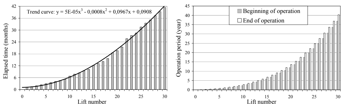
Figure 3.27 (a) Simulation des durées d'exploitation des 30 couches (b) Simulation du phasage d'exploitation cumulé des 30 couches (tassement exclu)
