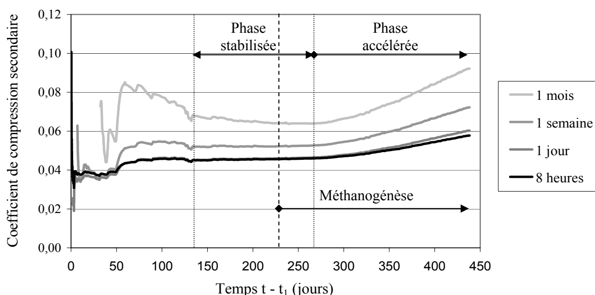
Figure 4.12 Evolution de C_{oe}^* en fonction du temps (suivant 4 valeurs de t_1 - t_0 ).
