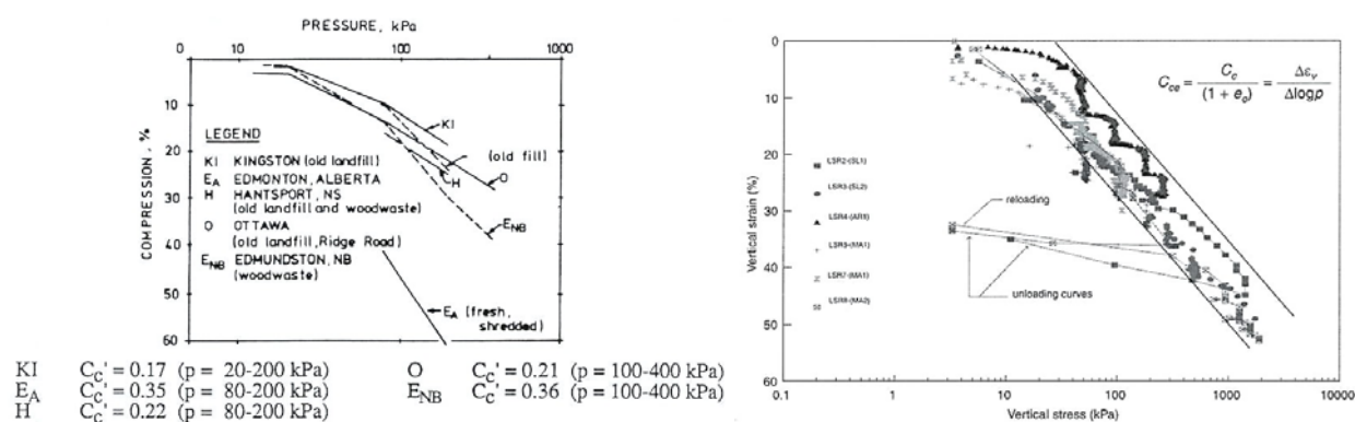
Figure 4.8 Déformation des déchets en fonction de la contrainte verticale (a) test à l'oedomètre 450 mm (Landva et Clark, 1990) (b) test à l'oedomètre 600 mm (Landva et al., 2000)
