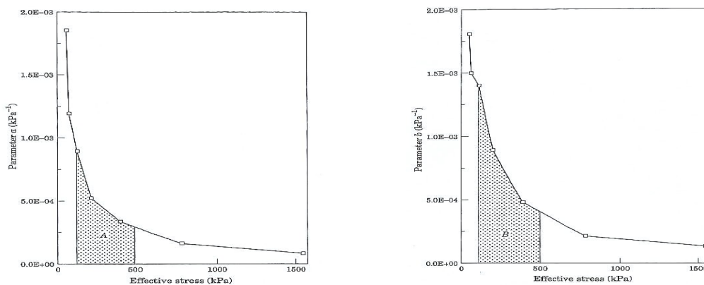
Figure 3.12 Valeurs de a et b proposées par Rao (1977)
