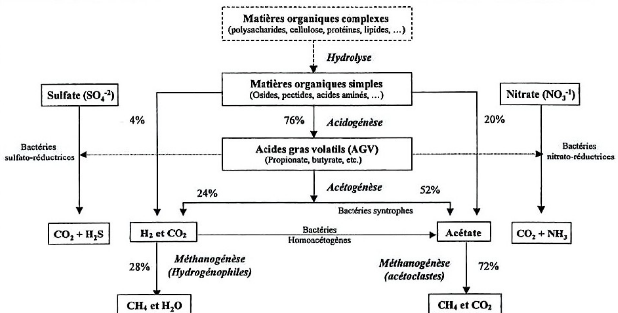
Figure 2.11 Processus de dégradation de la matière organique (Aguilar-Juarez, 2000)
