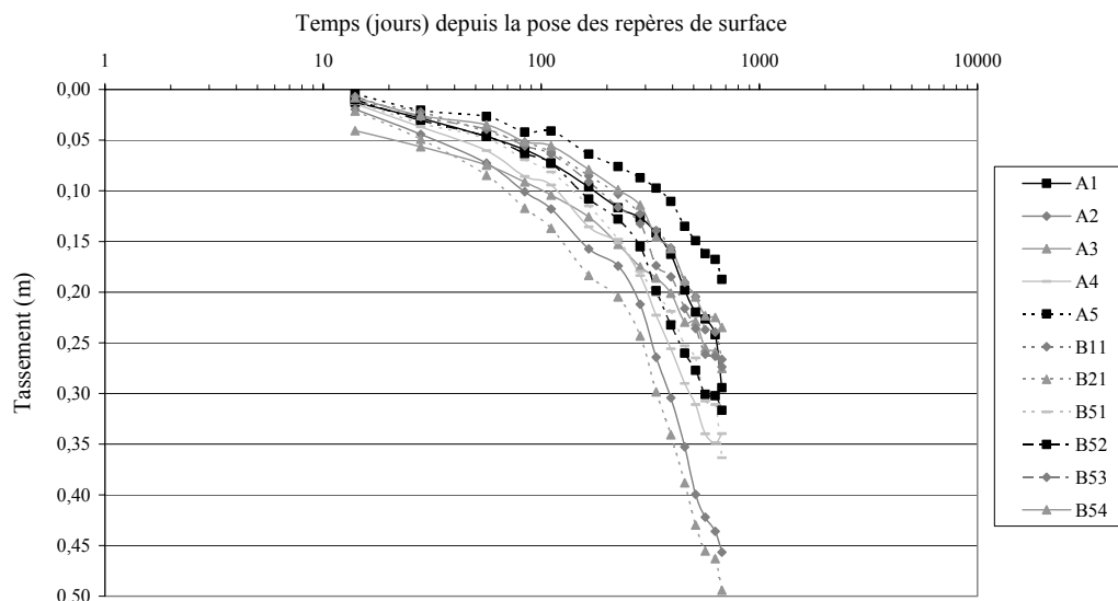
Figure 6.8 Evolution des tassements moyens des 11 profils de surface en fonction du logarithme de t - t_m^0 (Site de Lons-le-Saunier, H_n(t_c) = 10 m sauf A3 : 7 m)
