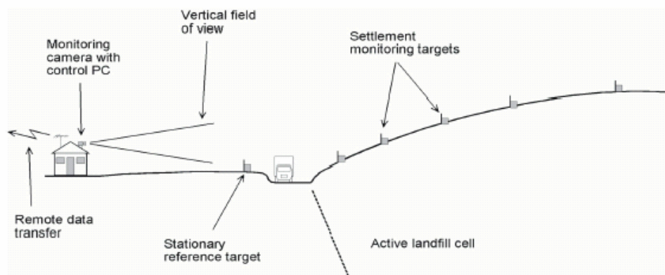
Figure 5.30 Schéma d'une instrumentation des tassements au moyen de cibles suivies par photographie digitale (White et al., 2003)
