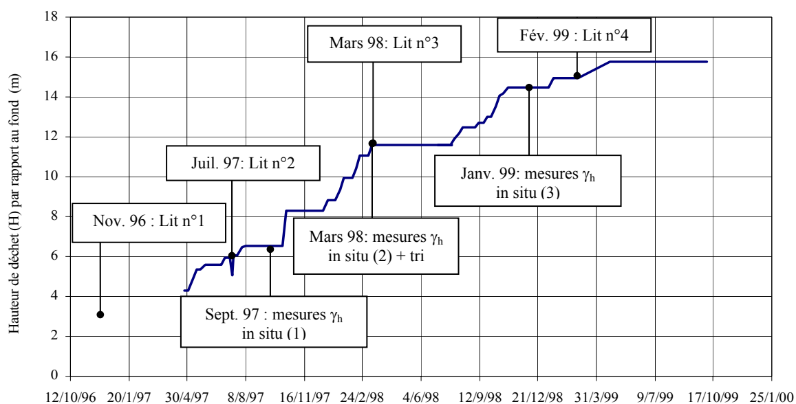
Figure 5.4 Phasage de montée de la colonne de déchet et déroulement des expérimentations
