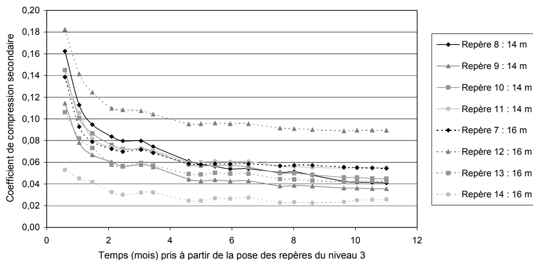
Figure 10.10 Evolution de C_{\alpha}^* en fonction de t - t_m^0 (Meruelo, niveau 3, 14 < H_n(t_c) < 16 m, t_m^0 - t_c = 7,03 mois)
