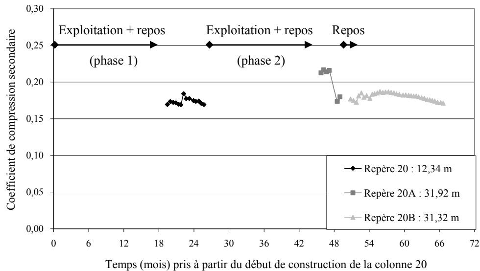
Figure 10.23 Evolution de C_{ac}^* au cours des 3 phases de suivi topographique (Site de Hong-Kong, Repères 20, 20A et 20B)
