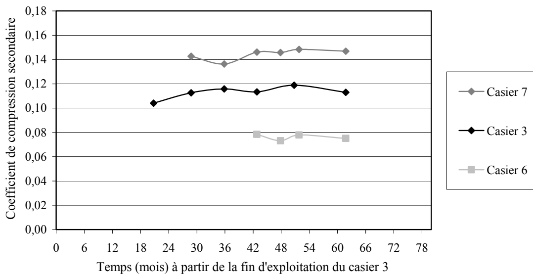
Figure 2.1.2 Evolution des C_{ac}^* en fonction de [t_m - (t_c)_{cell3}] (Novellara, casiers 3, 7 et 6)
