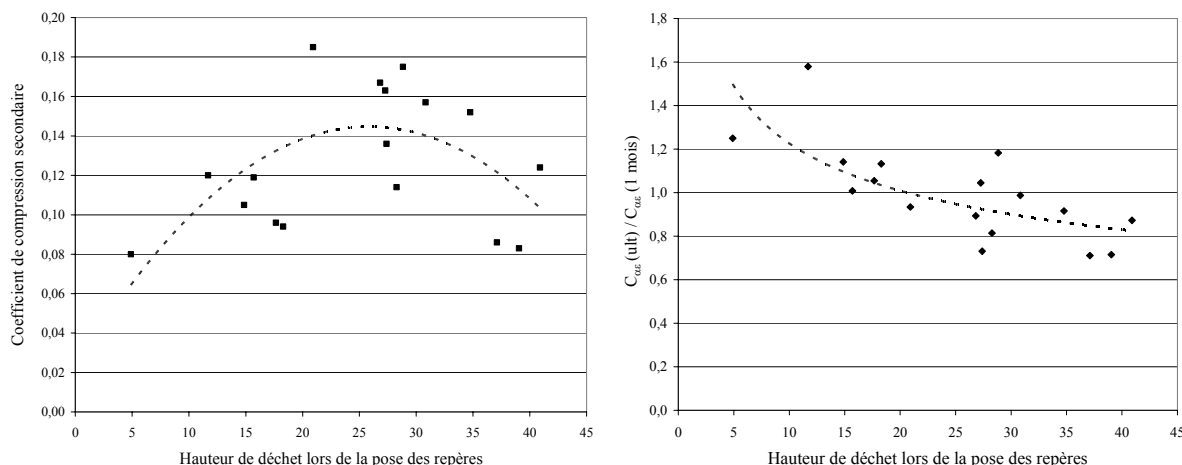
Figure 10.20 (a) Evolution de C_{ae}^* en fonction de la hauteur de déchet (b) Evolution de C_{ae}^*(t_m^{ult})/C_{ae}^*(t_m^2=1\text{ mois}) en fonction de la hauteur de déchet (Site de Hong-Kong, 17 repères du groupe 1)
