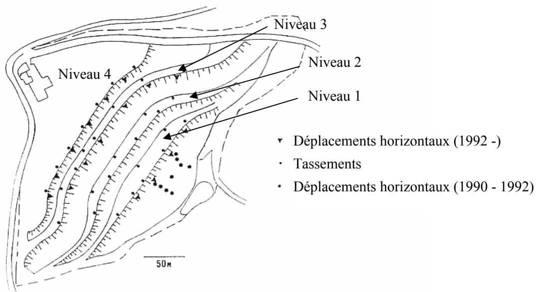
Figure 10.8 Instrumentation du site de Meruelo d'après Sánchez-Alciturri et al. (1993a)
