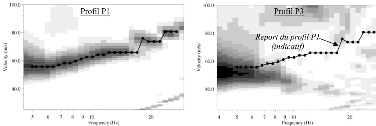
Figure 5.60 Courbe de dispersion de la vitesse des ondes de surface pour les profils P1 (Est) (source S2) et P3 (source S7) (Wathelet, non publié)
