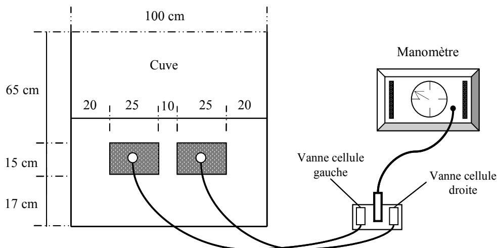
Figure 4.15 Positionnement des cellules de contrainte 'Glötz' à l'intérieur de la paroi avant de la cuve C4DC
