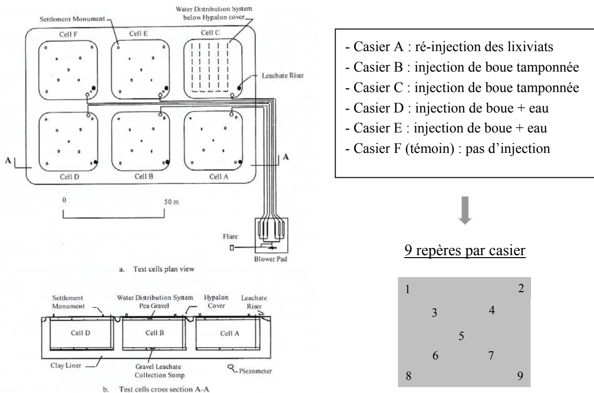
Figure 8.6 Schéma des 6 casiers de Mountain View et implantation des repères topographiques
