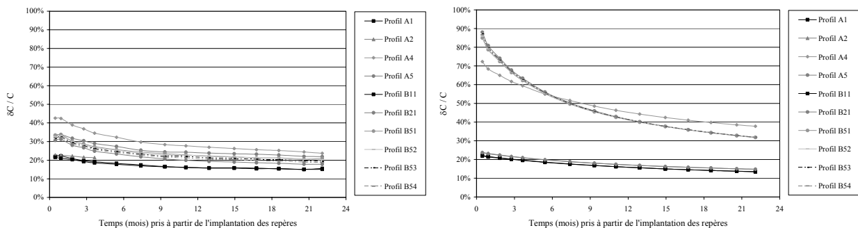
Figure 6.11 (a) Evolution de \left| C_{\alpha\epsilon}^*(t)_{NL20} - C_{\alpha\epsilon}^*(t)_{NL3} \right| / C_{\alpha\epsilon}^*(t)_{NL20} en fonction de t - t_m^0 (b) Evolution de \left| C_{\alpha\epsilon}^*(t)_{NL20} - C_{\alpha\epsilon}^*(t)_{L20} \right| / C_{\alpha\epsilon}^*(t)_{NL20} en fonction de t - t_m^0 (CSD de Lons-le-Saunier, tous profils sauf A3)
