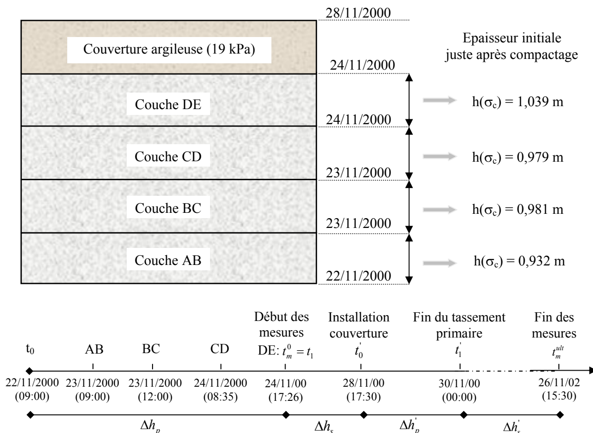
Figure 4.24 Historique complet de l'essai conduit par Watts et al. (2001)
