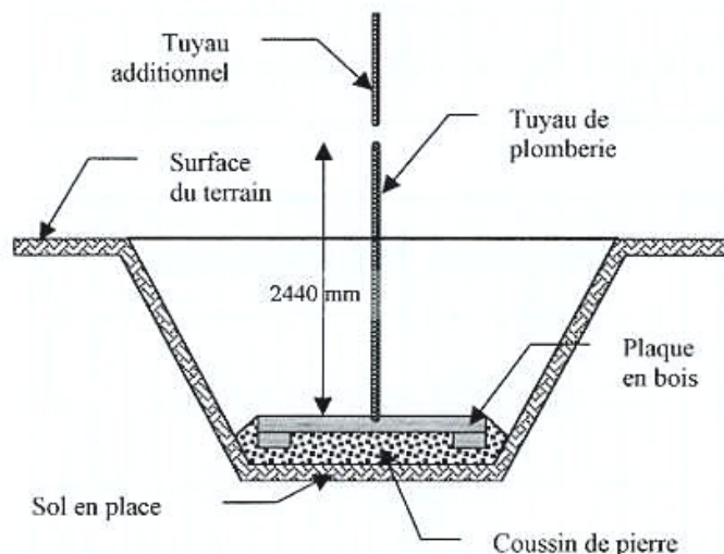
Figure 5.28 (a) Plaques de surface utilisées sur le CSD de Montréal (Moreau, 2001) (b) Exemples de bornes ancrées dans la couverture en terre végétale (CSD de Torcy et Lapouyade)
