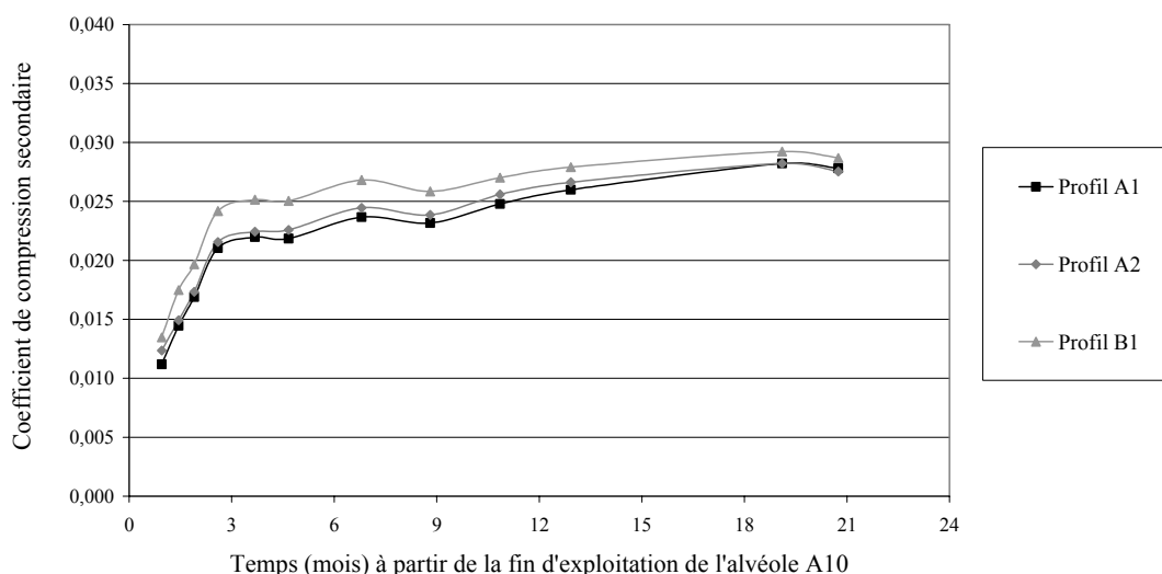
Figure 6.38 Evolution de C_{\alpha\varepsilon}^* en fonction de t - t_c (CSD de Lapouyade ; casier n° 2 ; alvéole A10 ; colonne 1 inférieure non surchargée : phase 1)
