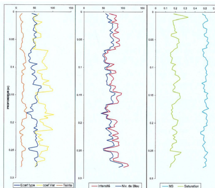
Figure 4.22 Evolution des paramètres de l'endoscope avec la profondeur (test n° 1 – C4DC essai n°2) (a) Ecart-type, coefficient de variance du niveau de gris et teinte (b) Intensité et niveau de gris (c) Saturation
