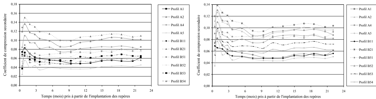
Figure 6.10 Evolution de C_{\alpha\epsilon}^* en fonction de t - t_m^0 (CSD de Lons-le-Saunier, tous profils sauf A3) (a) Modélisation non linéaire à 3 couches (NL3) (b) Modélisation linéaire à 20 couches (L20)
