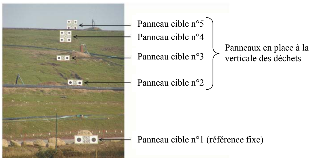
Figure 5.29 Illustration des panneaux cible sur le site de White's Pit (White et al., 2003)
