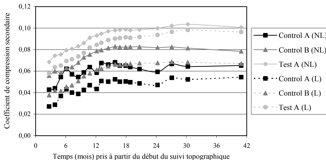
Figure 3.34 Evolution de C_{ac}^* en fonction du temps à partir de 2 hypothèses de modélisation : montée d'exploitation non linéaire (NL) / linéaire (L) (Site de Lyndhurst, zone 'Control')
