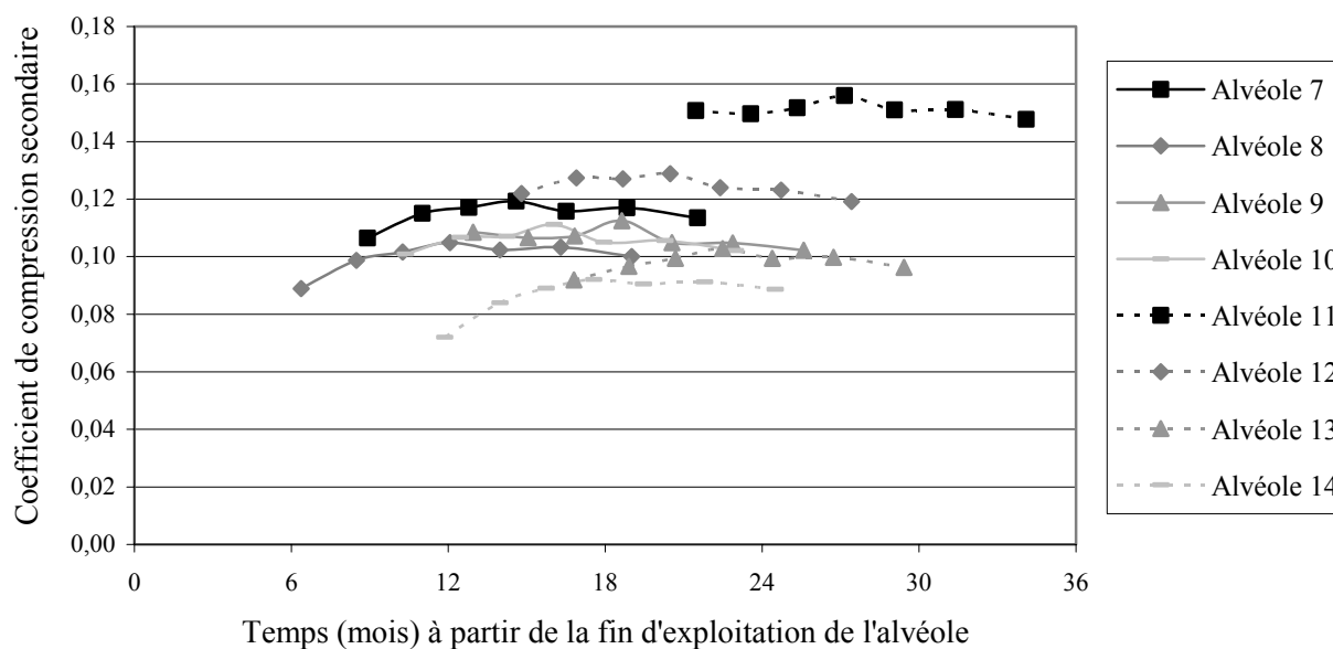
Figure 6.41 Evolution de C_{\alpha\epsilon}^* en fonction du temps ( t - t_c ) (CSD de Lapouyade, casier n° 2)
