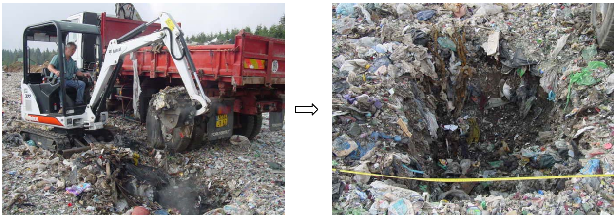
Figure 3.2 Excavation du puit à la pelle PP1 et mesure du volume de la cavité (Saint-Paul de Tartas)
