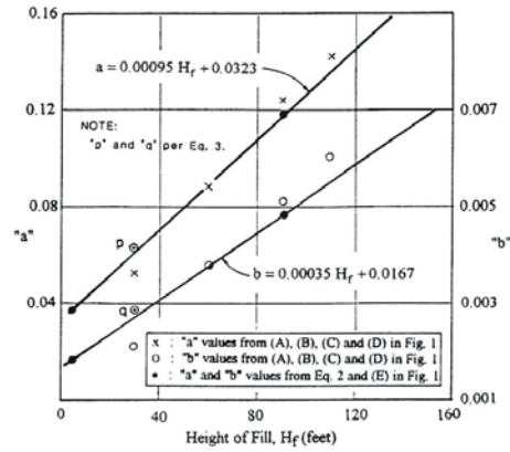
Figure 3.9 Evaluation des coefficients a et b en fonction de H(t_c) (Sohn et Lee, 1994)
