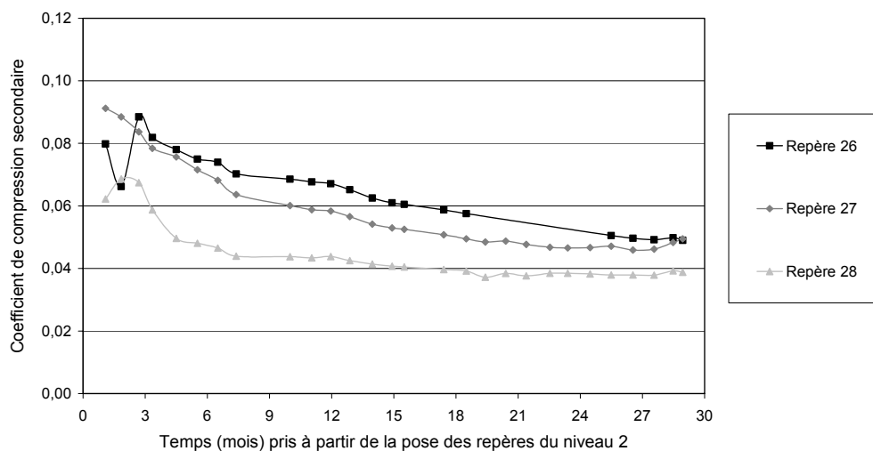
Figure 10.9 Evolution de C_{ac}^* en fonction de t - t_m^0 (Meruelo, niveau 2, H_n(t_c) = 15 m, t_m^0 - t_c = 4,11 mois)
