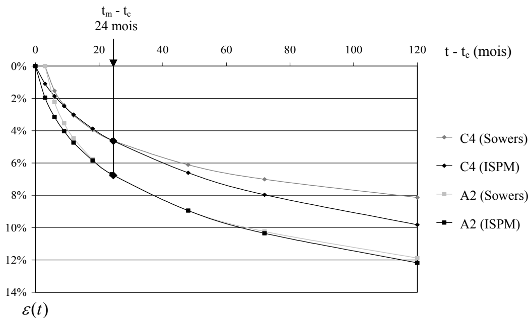
Figure 7.5 Evolution du tassement relatif \epsilon en fonction de t - t_c (colonnes A2 et C4 : nh_0/t_c = 1 m /mois ; t_1 = t_c + 3 mois)
