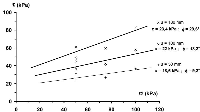
Figure 5.54 Représentation du plan de Mohr pour le déchet de Torcy (Thomas et al., 1999)
