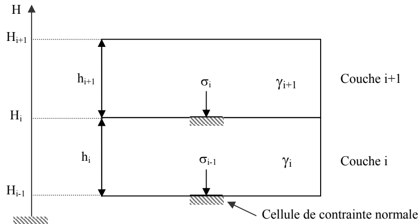
Figure 5.50 Principe du calcul du poids volumique d'une couche élémentaire de déchet d'indice i
