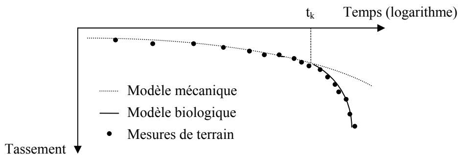
Figure 3.17 Allure générale du tassement modélisé par Edgers et al. (1992)
