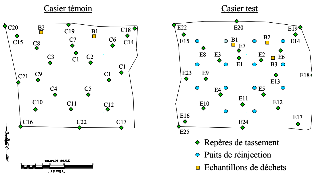
Figure 8.9 Schéma d'implantation des casiers de Yolo County
