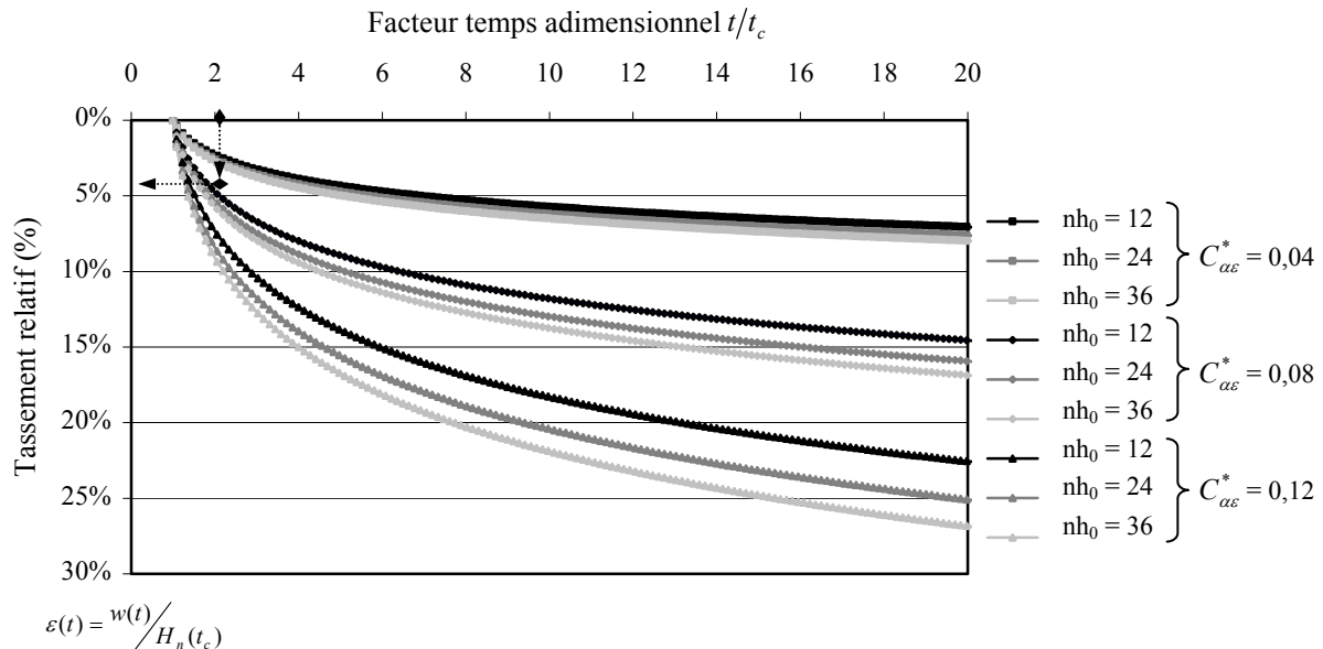
Figure 3.23 Abaque de prédiction des tassements ( C_R^* = 0,2 ; \gamma_0 = 8 \text{ kN/m}^3 ; t_m^0 \cong t_c \cong t_n )
