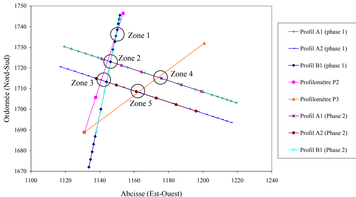
Figure 6.4 Implantation des profils topographiques sur l'alvéole A10 de Lapouyade
