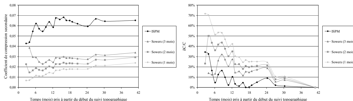
Figure 7.11 (a) Evolution comparée des coefficients de compression secondaire intrinsèques (modèle ISPM) et globaux (modèle de Sowers) en fonction de t_m - t_m^0 (b) Evolution du rapport \delta C/C en fonction de t_m - t_m^0 (Site de Lyndhurst, zone 'Control')
