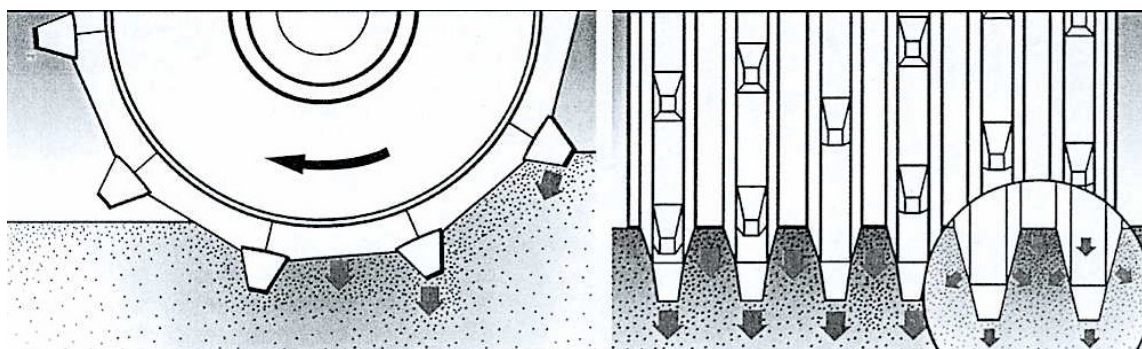
Figure 2.19 Schéma de transmission des contraintes des roues aux déchets
