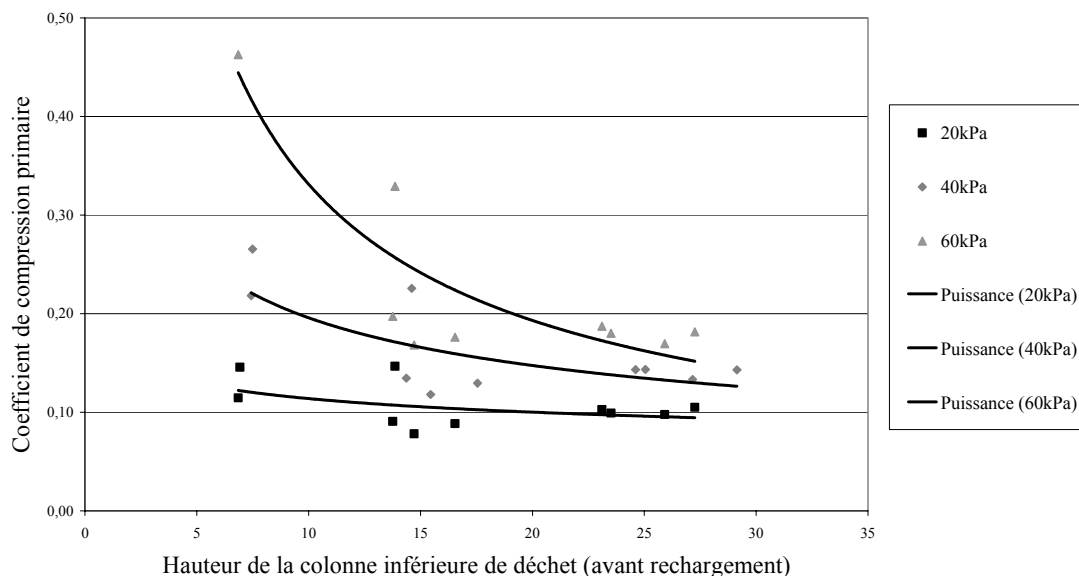
Figure 6.3 Influence de la pré-consolidation supposée (20, 40, 60 kPa) sur la valeur de C_R^* calculée pour des hauteurs de déchet variables (alvéole A''B ; phase de rechargement de la colonne inférieure) ; d(t_m^0) : 19/04/2001 ; d(t_m^{ult}) : 17/09/2001]
