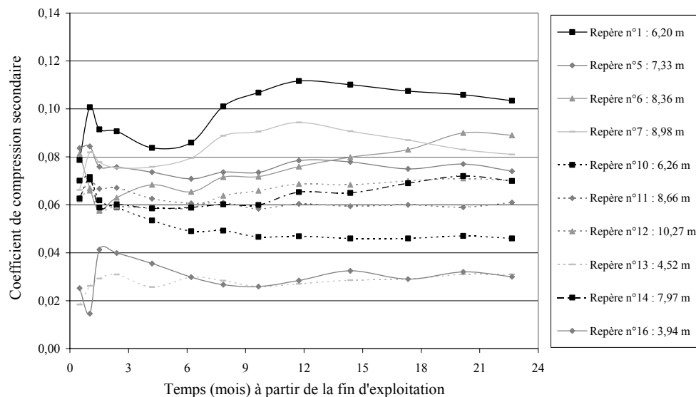
Figure 6.34 Evolution de C_{\alpha\epsilon}^* en fonction de [t - (t_c)_{Phase 2}] (CSD de Chatuzange ; alvéole A''B ; suivi de la colonne de déchet 2 supérieure)
