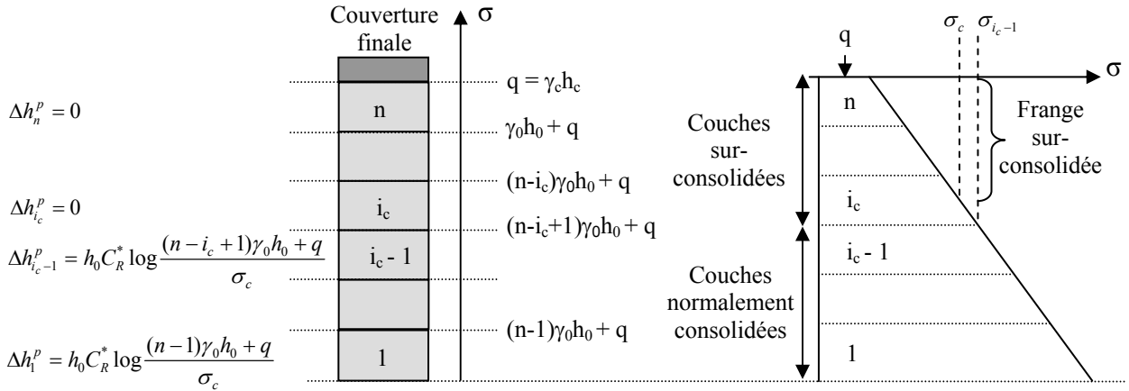
Figure 3.21 Expressions du tassement primaire pour les couches élémentaires d'indice 1 à n
