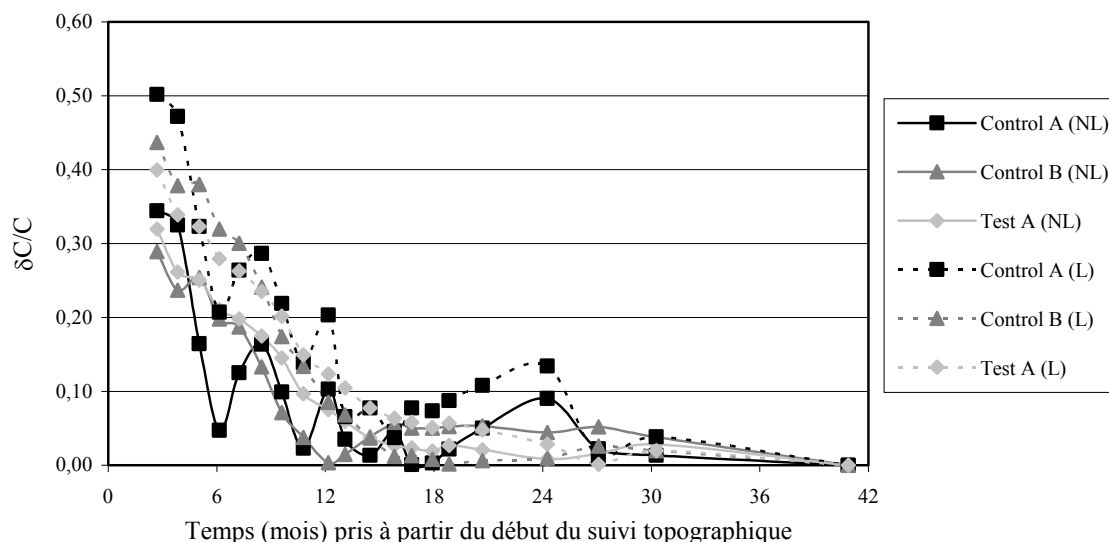
Figure 3.35 Evolution de \delta C / C en fonction du temps à partir de 2 hypothèses de modélisation : montée d'exploitation non linéaire (NL) / linéaire (L) (Site de Lyndhurst, zone 'Control')
