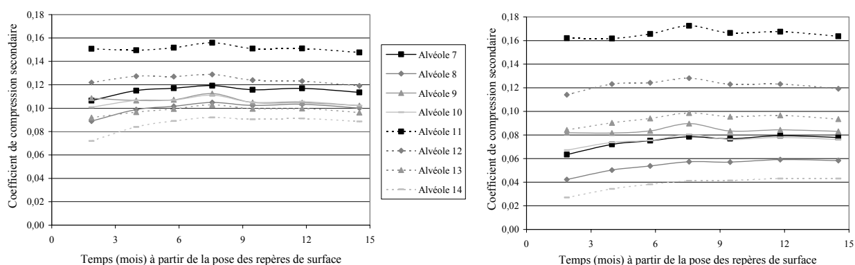
Figure 7.13 Evolution du coefficient de compression secondaire en fonction de t_m - t_m^0 (CSD de Lapouyade, casier n° 2, alvéole A7 à A14) (a) Coefficient C_{\alpha\epsilon}^* tiré du modèle ISPM (b) Coefficient C_{\alpha\epsilon} tiré du modèle de Sowers
