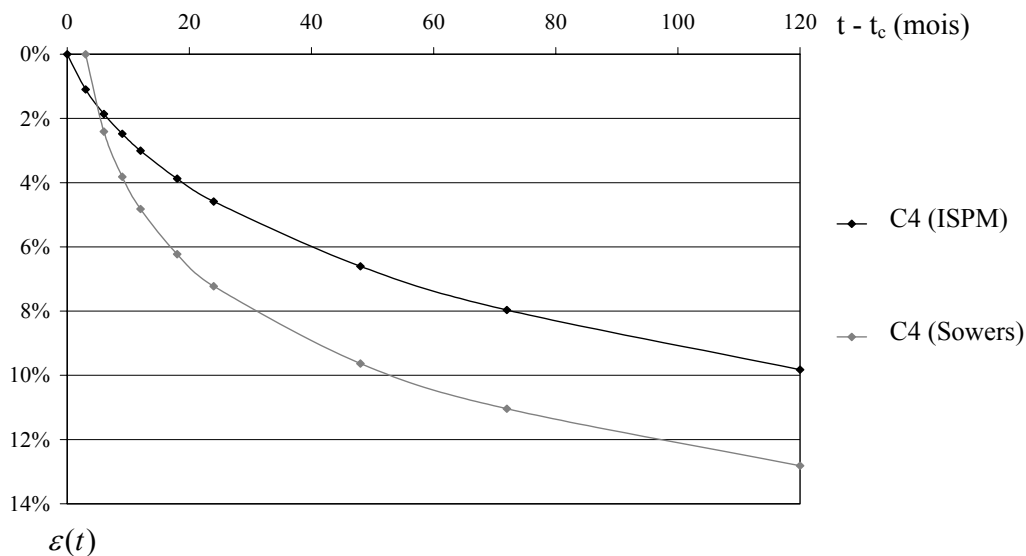
Figure 7.6 Evolution du tassement relatif \varepsilon en fonction de t - t_c (Colonne C4 : nh_0/t_c = 1 m /mois ; C_{\alpha\epsilon} = C_{\alpha\epsilon}^* = 0,08 ; t_1 = t_c + 3 mois)
