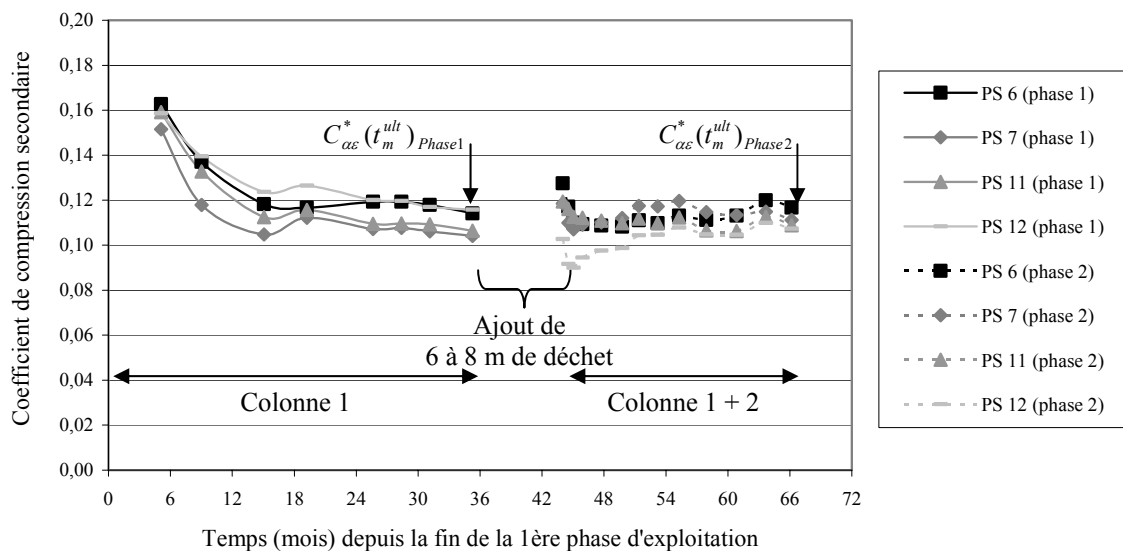
Figure 6.26 Evolution de C_{ac}^* en fonction de [t - (t_c)_{Phase1}] (CSD de Chatuzange ; alvéole A''B ; Phase 1 : suivi de la colonne 1 inférieure ; Phase 2 : suivi de la colonne 1 + 2)
