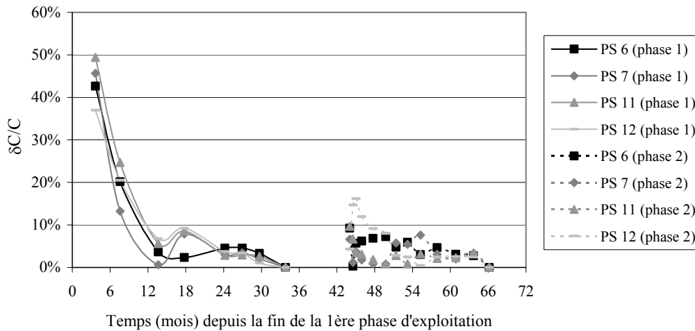
Figure 6.27 Evolution de \left| \frac{C_{ae}^*(t) - C_{ae}^*(t_m^{ult})}{C_{ae}^*(t_m^{ult})} \right| en fonction du temps [t - (t_c)_{Phase 1}] (CSD de Chatuzange ; alvéole A''B ; phase 1 : suivi de la colonne 1 inférieure ; phase 2 : suivi de la colonne 1 + 2)
