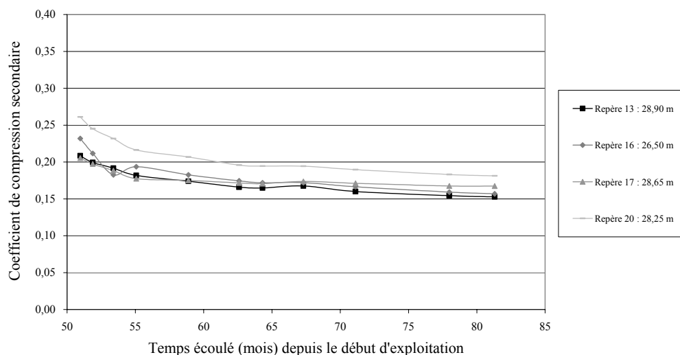
Figure 6.23 Evolution du coefficient (C_{ac}^*)_{\text{colonne 1}} en fonction du temps t depuis le début d'exploitation de l'alvéole AA' (suivi topographique sur couverture provisoire : t_{c1} = 35 mois)
