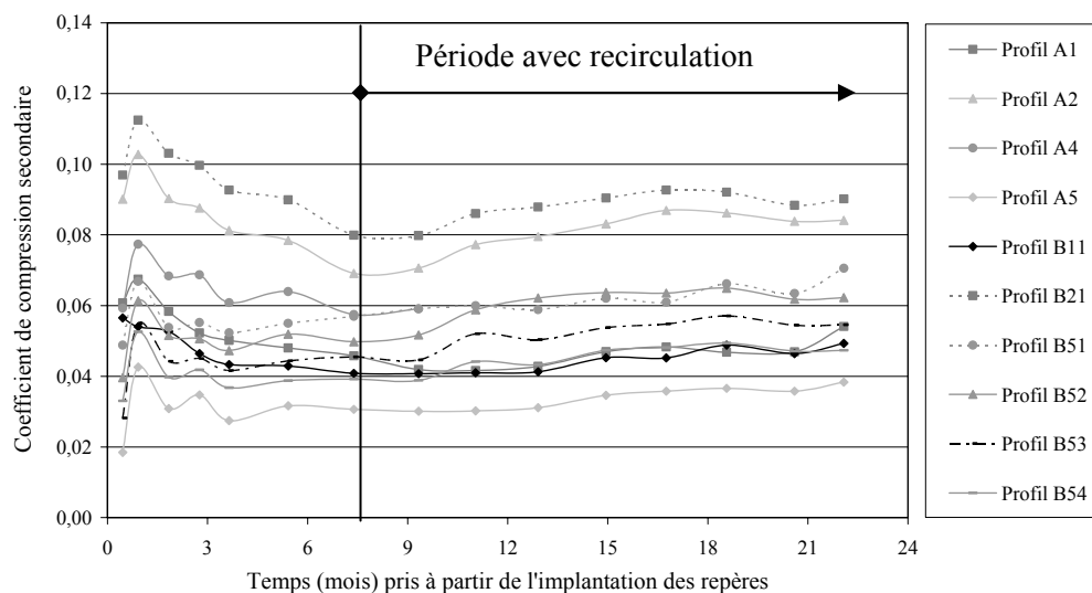
Figure 6.9 Evolution de C_{\alpha\alpha}^* en fonction de t - t_m^0 . Modélisation non linéaire à 20 couches (NL20). (CSD de Lons-le-Saunier, tous profils sauf A3)
