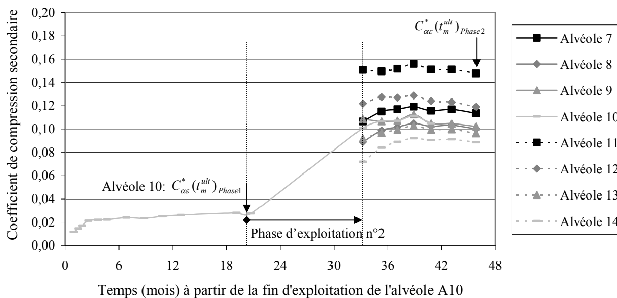
Figure 6.42 Evolution de C_{\alpha\epsilon}^* en fonction du temps [ t - (t_c)_{A10} ] (CSD de Lapouyade, casier n° 2)
