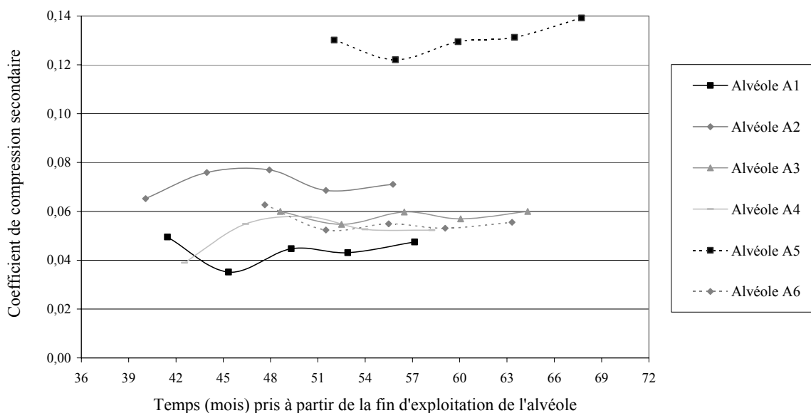
Figure 6.43 Evolution de C_{\alpha\epsilon}^* en fonction du temps ( t - t_c ) (CSD de Lapouyade, casier n° 1)
