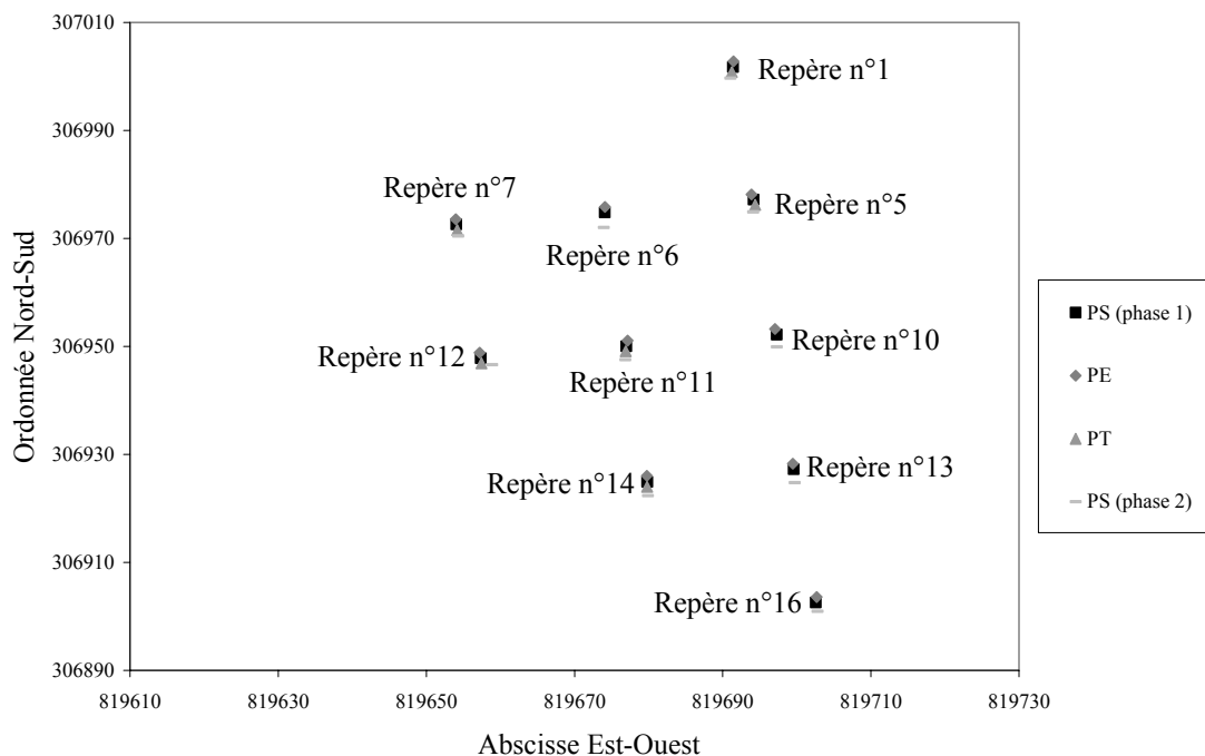
Figure 6.2 Implantation des plaques et tiges topographiques sur l'alvéole A''B de Chatuzange
