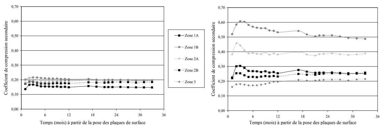
Figure 7.14 Evolution du coefficient de compression secondaire en fonction de t_m - t_m^0 (CSD de Montréal, zones 1A à 3) (a) Coefficient intrinsèque C_{\alpha\epsilon}^* tiré du modèle ISPM (b) Coefficient C_{\alpha\epsilon} global tiré du modèle de Sowers (application différentielle à partir de t_m^0 = t_c + \Delta t )
