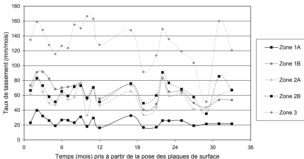
Figure 6.19 Evolution des taux de tassement en fonction de t - t_m^0 (CSD de Montréal)
