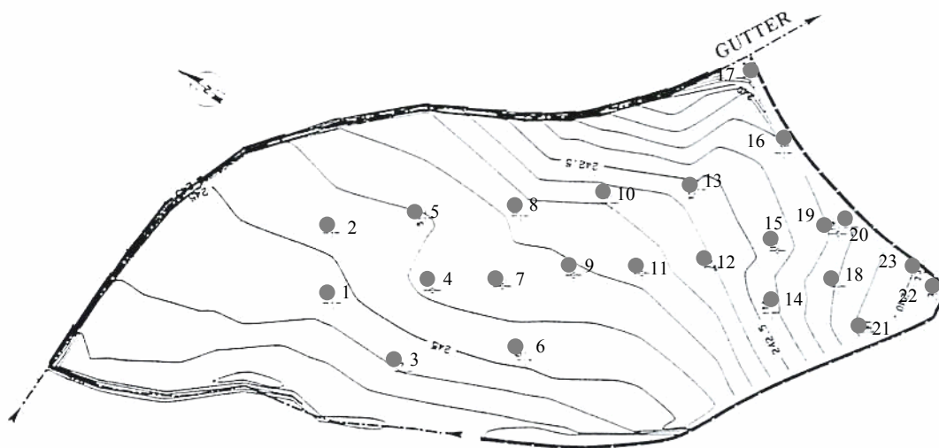
Figure 10.3 Implantation des repères topographiques de Rio Vigne d'après Gasparini et al. (1991)
