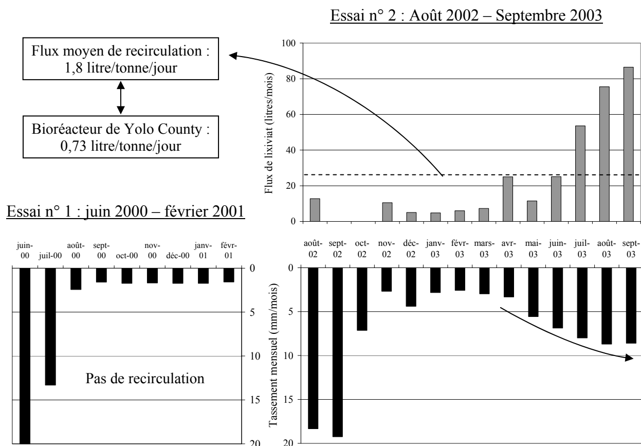
Figure 4.13 Evolution des tassements mensuels en fonction de la recirculation (essais n° 1 et 2).
