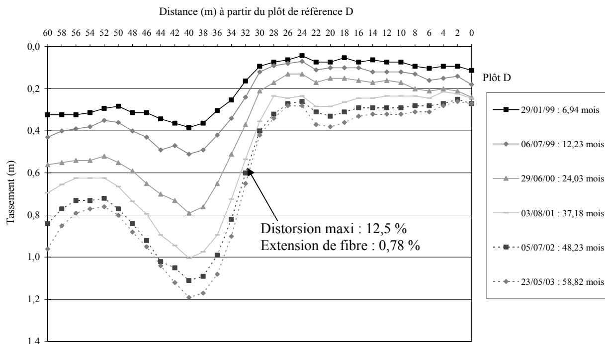
Figure 9.16 Evolution des profils de tassement le long du profilomètre n°2 (Montech, casiers G et H)
