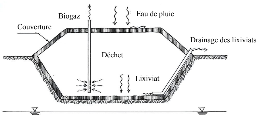
Figure 1.2 Schéma de principe d'un casier de stockage de déchet repris d'après Del Greco et al. (1993)
