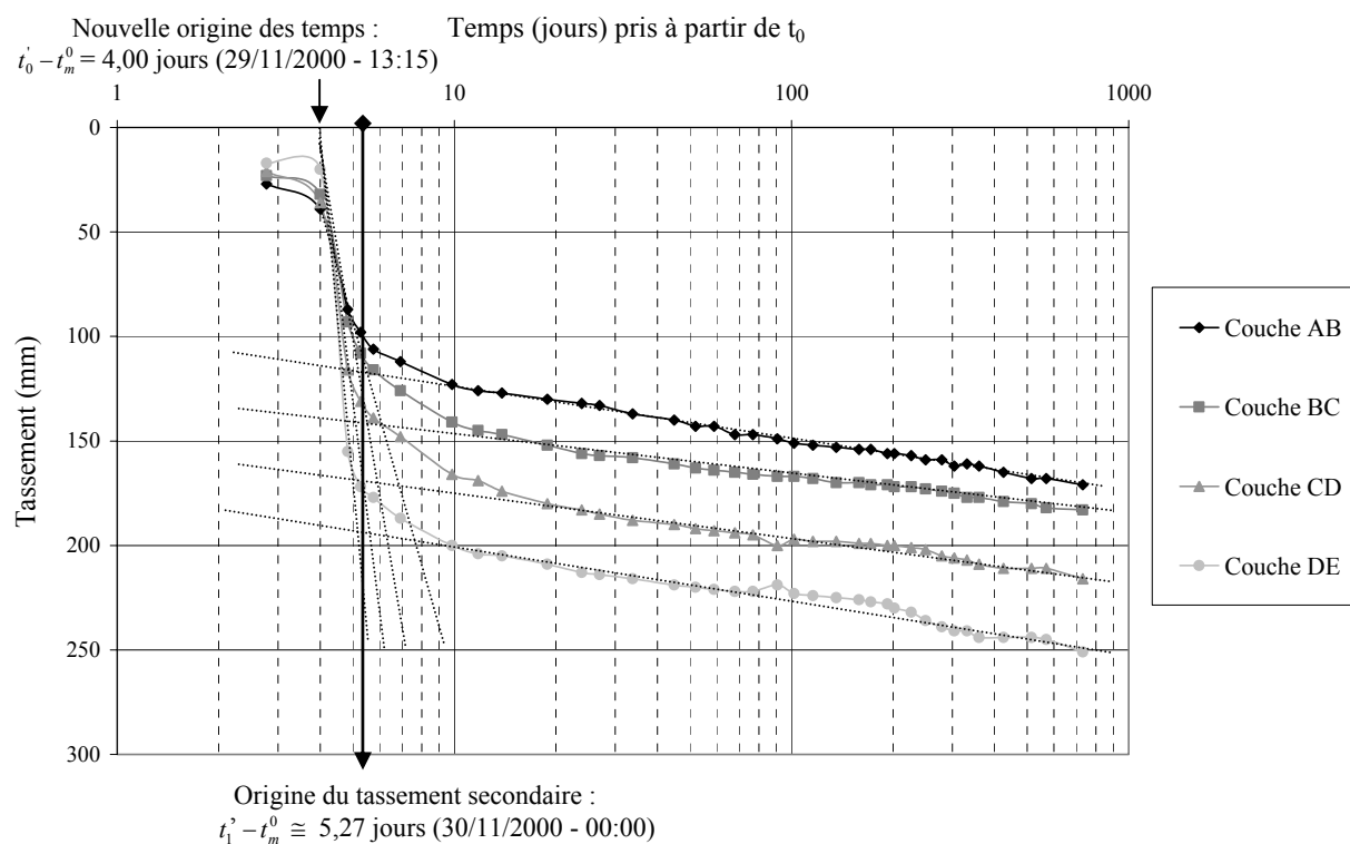
Figure 4.24 Historique complet de l'essai conduit par Watts et al. (2001)
