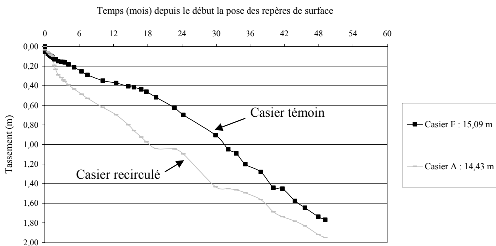
Figure 8.7 Courbes de tassement des mini-casiers A (recirculé) et F (témoin) de Mountain View
