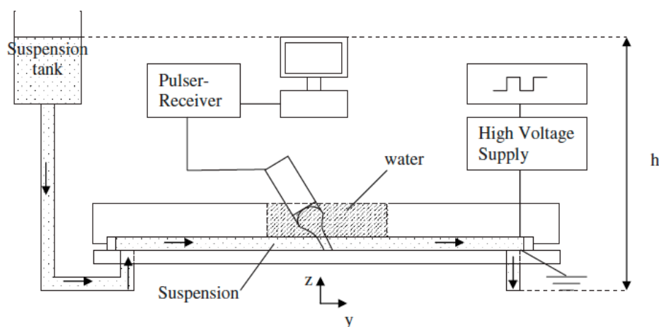
FIGURE 1.10 – Vélocimétrie par diffusion ultrasonore : dispositif expérimental
