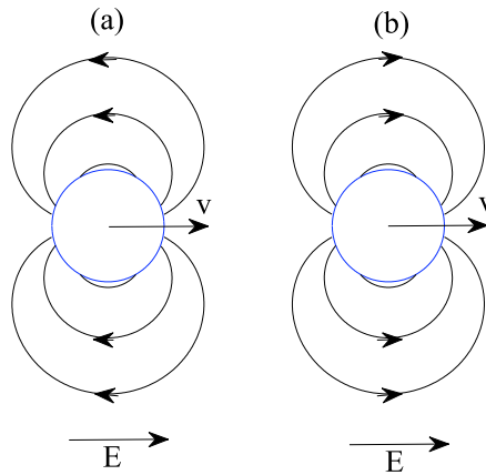
FIGURE 3.4 – Perturbation due au mouvement électrophorétique d'une particule chargée. (a) champ de vitesse (b) champ électrique.
