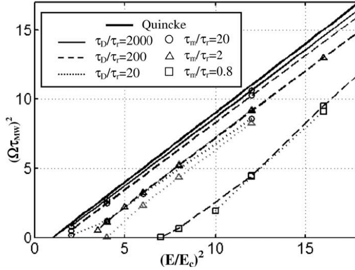
FIGURE 1.15 – Carré de la vitesse de rotation normalisée en fonction du carré de l'intensité du champ normalisée. \tau_{MW} = \tau_{MW}/2 . E_c est l'intensité du champ électrique critique dans le cadre du modèle classique de Quincke.
