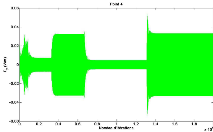
FIG. 2.40: Allure temporelle au point 4 d'une composante du champ à l'intérieur d'une cavité résonnante de conductivité \sigma = 1719\text{S/m} simulée en utilisant un maillage «grossier».
