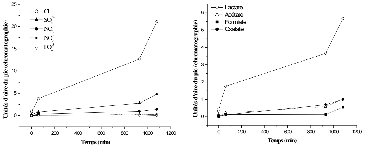
Figure Annexe-83 : Evolution des concentrations en composés inorganiques (à gauche) et des acides organiques (à droite) au cours du temps dans l'eau de nuage artificielle pulvérisée dans la « machine à nuage » (en unités d'aire de chromatographie ionique, proportionnelle pour un même composé à sa concentration).
