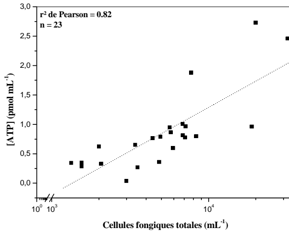
Figure 47 : Relation entre les concentrations en ATP et en cellules fongiques totales.
