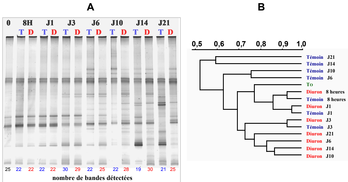
Figure D-13 : (A) Evolution des profils obtenus par TTGE dans les microcosmes témoins (T) et contaminés (D) à J0 (0), après 8 heures (8H) puis de J1 à J21 ; (B) dendrogramme calculé par la méthode DICE-UPGMA à partir du profil TTGE en tenant compte de l'intensité relative de chacune des bandes.
