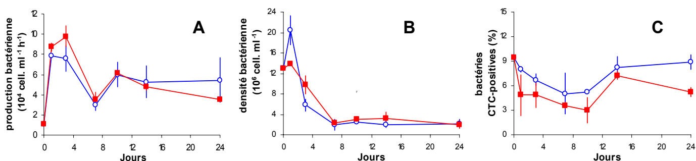
Figure D-23 : Evolution moyenne (et écarts-types) de la production bactérienne hétérotrophe ( 10^4 cell. ml -1 h -1 ) (A), de la densité bactérienne ( 10^6 cell. ml -1 ) (B) et du pourcentage de bactéries CTC-positives (C) dans les microcosmes témoins (○) et contaminés (■).
