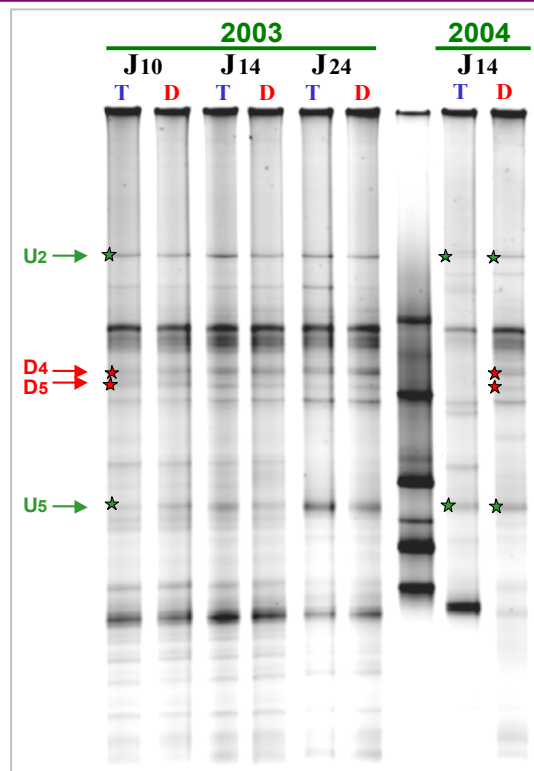
Figure D-26 : Localisation des bandes communes aux deux expériences (2003 et 2004).
