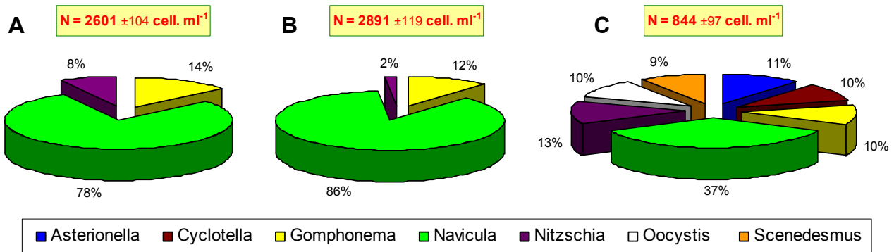
Figure D-32 : Densités algales initiales (cell. ml -1 ) et structure de la communauté lors des études menées en mars 2003 ( A ), avril 2004 ( B ) et août 2004 ( C ).
