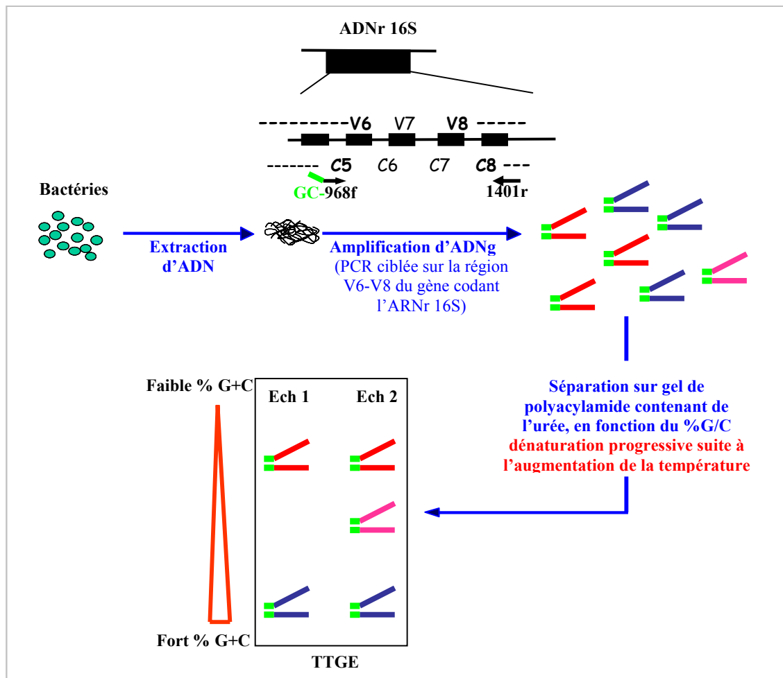
Figure B-5 : Schématisation du principe de l'électrophorèse sur gel à gradient temporel de température.
