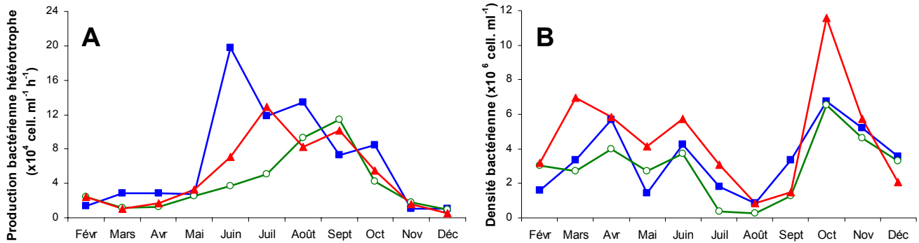
Figure C-22 : Evolution mensuelle de la production bactérienne hétérotrophe ( \times 10^4 cell \text{ml}^{-1} \text{h}^{-1} , A ) et des densités bactériennes ( \times 10^6 cell \text{ml}^{-1} , B ) aux stations JAU1 (■), JAU3 (○) et JAU4 (▲) en 2004.
