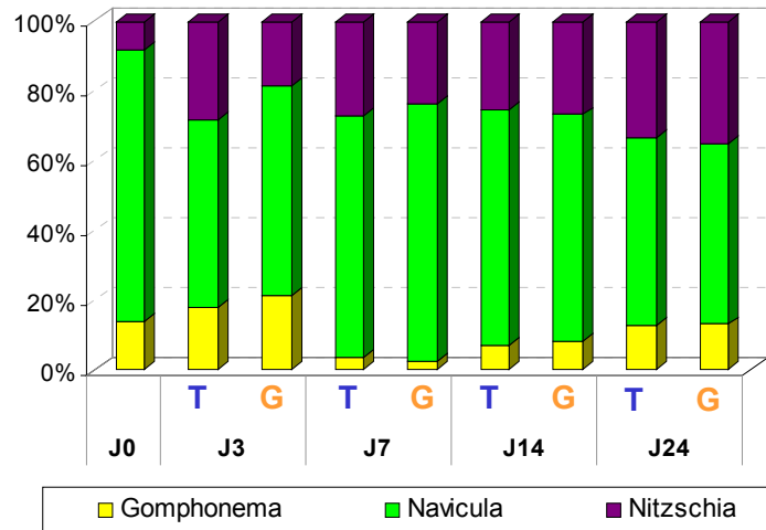
Figure D-33 : Evolution moyenne de la structure de la communauté algale lors de l'étude menée en mars 2003 dans les microcosmes témoins (T) et contaminés au glyphosate (G).
