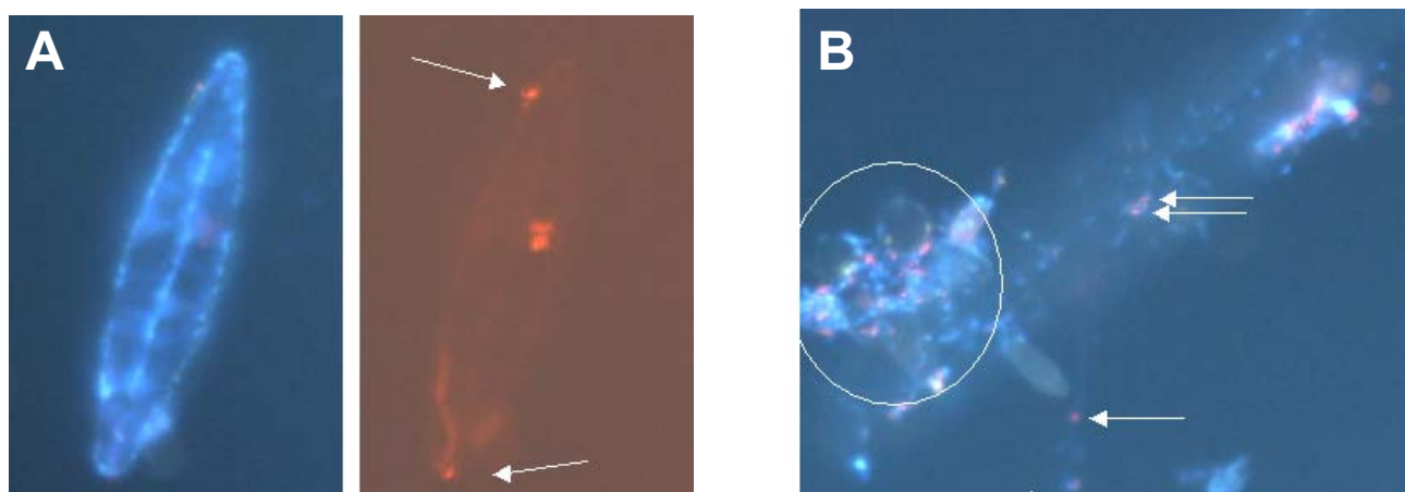
Figure D-17 : Visualisation de bactéries CTC-positives sur une cellule algale du genre Navicula ( A ) et sur un amas de débris organiques ( B ).
