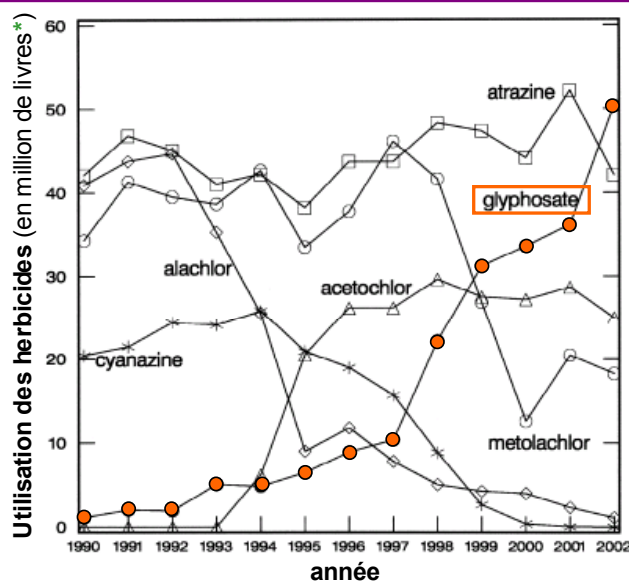
Figure A-15 : Evolution de l'utilisation estimée d'herbicides dans l'agriculture de 9 états de l'Ouest des Etats-Unis (Battaglin et al. , 2005) * 1 livre = 453,6 grammes.
