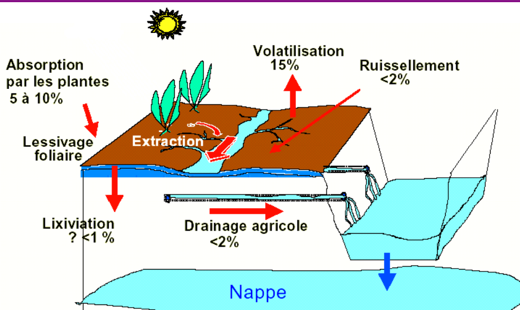
Figure A-2 : Schématisation du transfert des pesticides hors des parcelles agricoles (Garon-Boucher Margoum, 2003 d'après Voltz, 2001).
