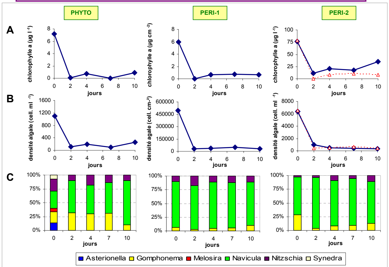
Figure D-4 : Evolution de la concentration en chlorophylle a (A), de la densité algale (B) et de la composition taxonomique (C) dans les trois types de microcosmes.
