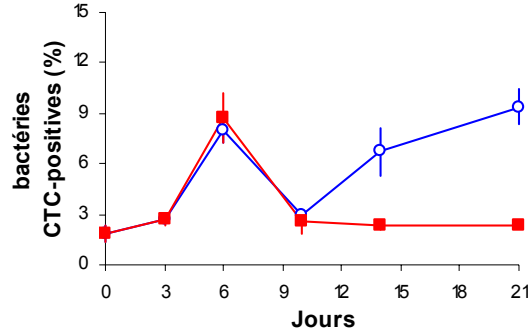
Figure D-11 : Evolution moyenne (et écarts-types) du pourcentage de bactéries CTC-positives dans les microcosmes témoins (○) et contaminés (■).
