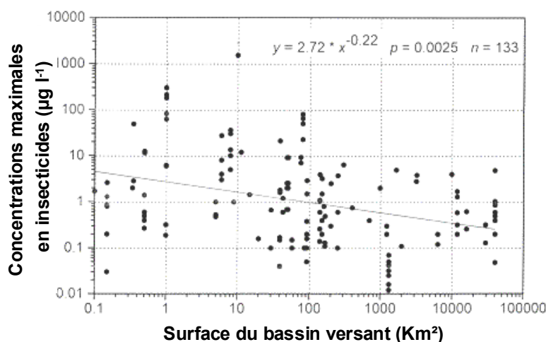
Figure C-1 : Relation entre la surface du bassin versant et les concentrations maximales en insecticides détectées dans des eaux de rivière (d'après Schultz, 2004).
