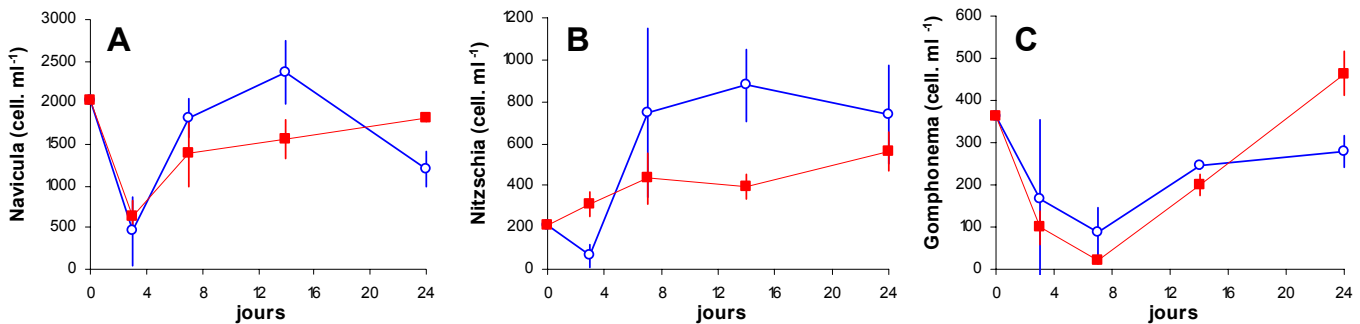
Figure D-22 : Evolution moyenne (et écarts-types) de l'abondance (cell. ml -1 ) des espèces appartenant aux genres Navicula (A), Nitzschia (B) et Gomphonema (C) dans les microcosmes témoins (○) et contaminés (■).
