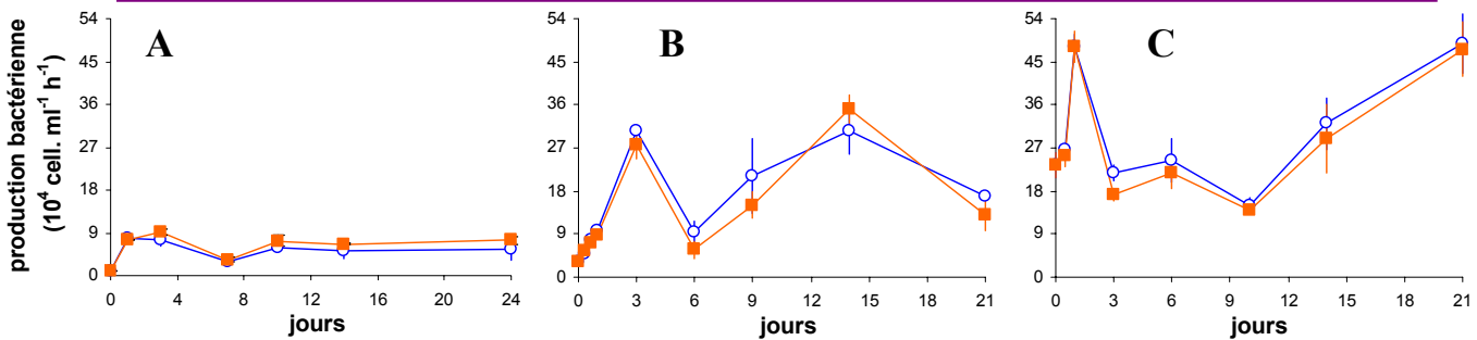
Figure D-35 : Evolution moyenne (et écarts-types) de la production bactérienne hétérotrophe ( 10^4 cell. \text{ml}^{-1} \text{h}^{-1} ) lors des études menées en mars 2003 (A), avril 2004 (B) et août 2004 (C).
