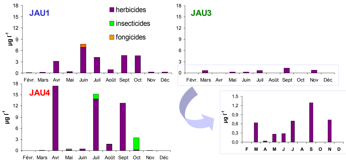
Figure C-5 : Evolution mensuelle des concentrations ( \mu\text{g l}^{-1} ) en pesticides aux stations JAU1, JAU3 et JAU4 en 2003.
