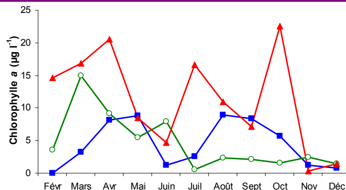
Figure C-18 : Evolution mensuelle des concentrations ( \mu\text{g l}^{-1} ) en chlorophylle a planctonique aux stations JAU1 (■), JAU3 (○) et JAU4 (▲) en 2004.
