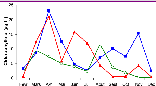
Figure C-6 : Evolution mensuelle des concentrations ( \mu\text{g l}^{-1} ) en chlorophylle a aux stations JAU1 (■), JAU3 (○) et JAU4 (▲) en 2003.
