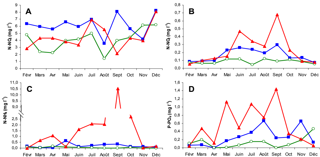
Figure C-4 : Evolution mensuelle des concentrations ( \text{mg l}^{-1} ) en \text{N-NO}_3 (A), \text{N-NO}_2 (B), \text{N-NH}_4 (C) et \text{P-PO}_4 (D) aux stations JAU1 (■), JAU3 (○) et JAU4 (▲) en 2003.
