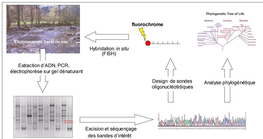
Figure B-7 : Exemples de possibilités offertes par les méthodes d'électrophorèse sur gel dénaturant dans l'étude de la structure des communautés bactériennes (modifié d'après Muyzer, 1999)
