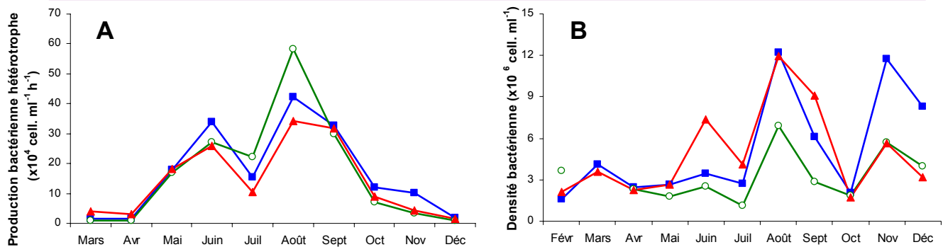
Figure C-9 : Evolution mensuelle de la production bactérienne hétérotrophe ( \times 10^4 cell ml^{-1} h^{-1} , A ) et des densités bactériennes ( \times 10^6 cell ml^{-1} , B ) aux stations JAU1 (■), JAU3 (○) et JAU4 (▲) en 2003.
