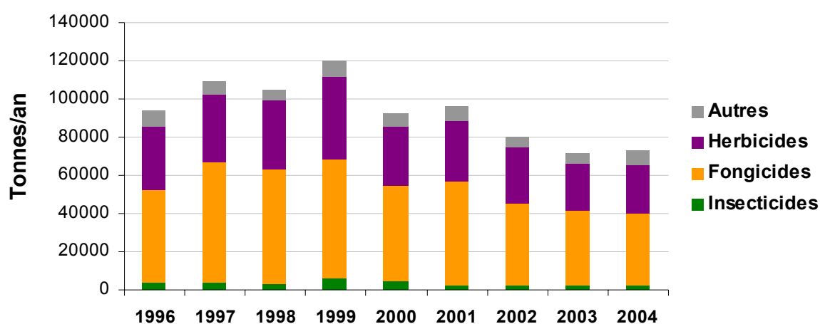
Figure A-1 : Évolution des quantités de pesticides commercialisées en France entre 1996 et 2004, (IFEN, 2004, 2006 ; données de l'Union des Industries de la Protection des Plantes, http://www.uipp.org/ ).
