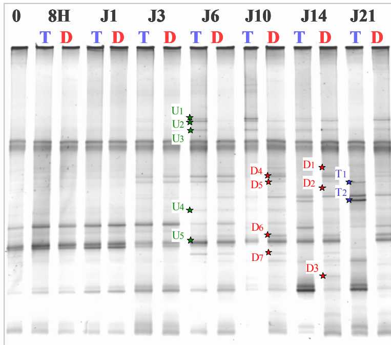
Figure D-14 : Choix des bandes d'intérêt excisées pour l'analyse phylogénétique.
