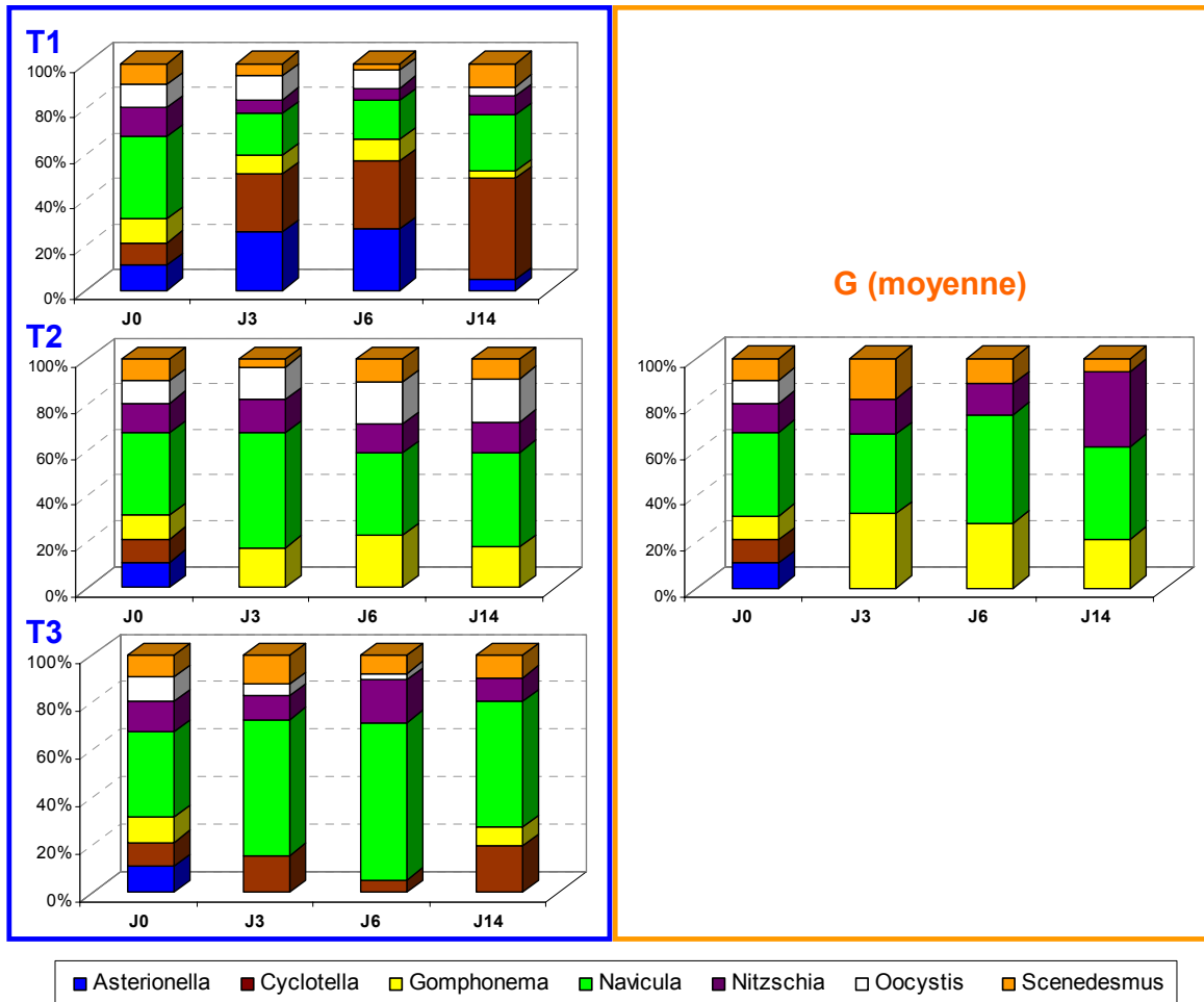
Figure D-34 : Evolution de la structure de la communauté algale lors de l'étude menée en août 2004 dans les trois microcosmes témoins ( T1, T2, T3 ) et, en moyenne, dans les microcosmes contaminés au glyphosate ( G ).
