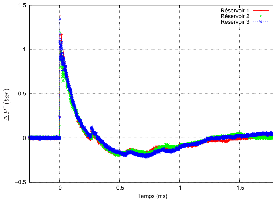
FIGURE 3.7 – Reproductibilité de la surpression réfléchi à 0^\circ pour des essais sur les trois réservoirs rigides (bulle de 6 cm à 40 cm)
