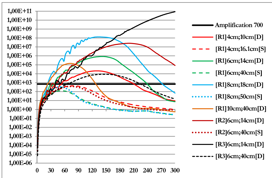
FIGURE 4.25 – Amplification maximale pour les différents essais réalisés (charge de rayon R_o à une distance d ) pour les différents réservoirs ([R1],[R2],[R3]) et type d'état après essai ([D] : Damaged (Flambé) ; [S] : Safe (Sain)).
