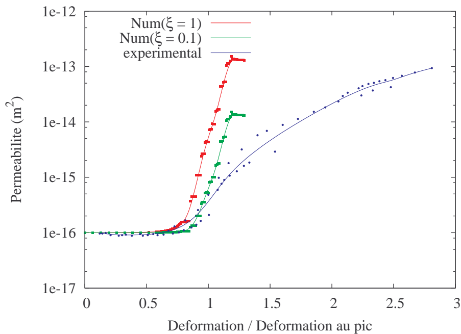
FIGURE 4.10 – Superposition de résultat numérique k_V en 2D avec le résultat expérimental de Choinska
