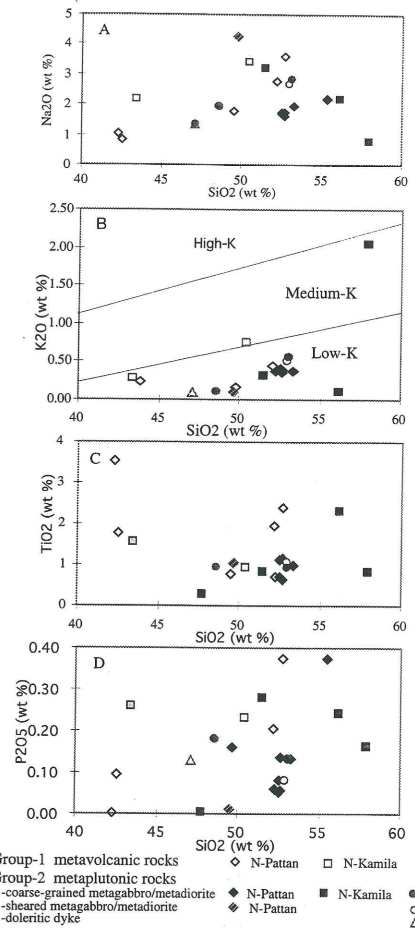
Figure 8. Harker variation diagrams for major elements in different facies of the Kamila Amphibolites. Diagrammes de Harker pour les différents faciès des amphibolites de Kamila.
