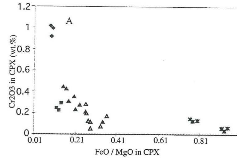
◆ Dunite ■ Ol-clinopyroxenite ▲ Websterite Δ Ga-websterite ✕ Ga-gabbro
