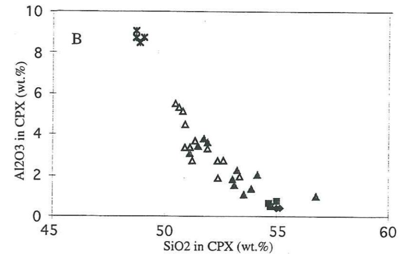
◆ Dunite ■ Ol-clinopyroxenite ▲ Websterite Δ Ga-websterite ✕ Ga-gabbro
