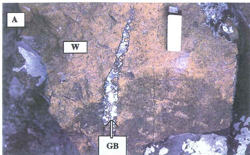
A = Anorthositic gabbro trapped in wehrlite/dunite body Photographie d'un gabbro à anorthose (GB) piégé dans une fente ouverte dans un massif de wehrlite/dunite.
