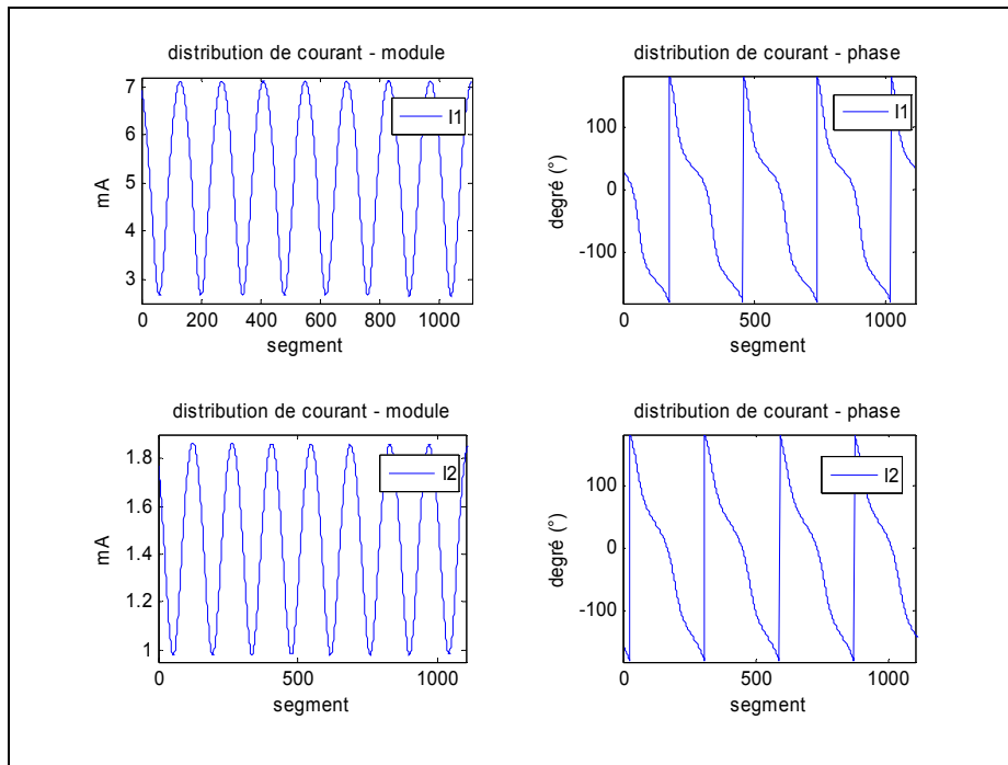
Figure III-25 : Distribution de courant – Câble bifilaire rectiligne (module/phase) théorie NMTL (F = 12 MHz, L = 100 m, h = 50 cm, diamètre = 2 mm, d = 10 cm)
