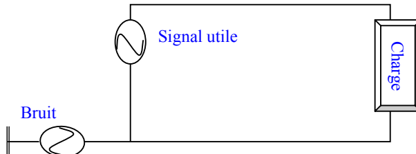
Figure I-8 : Modélisation du bruit de mode commun
