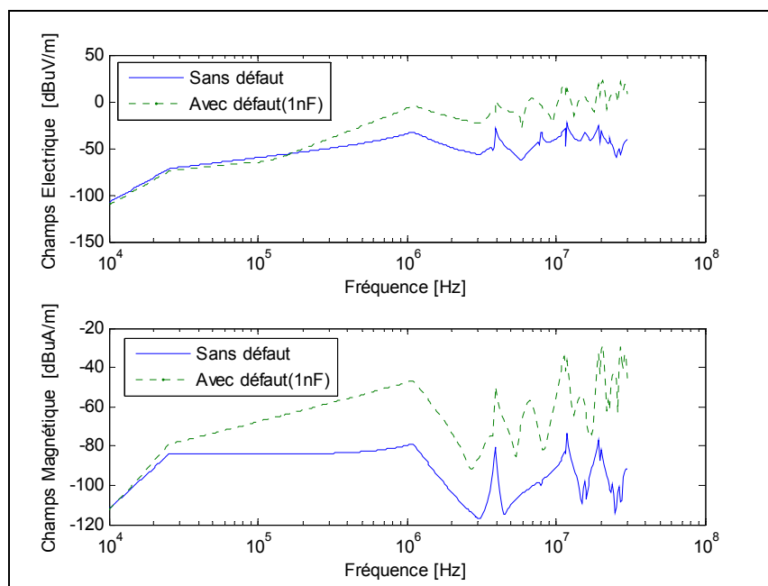
Figure IV-23 : Influence d'un défaut capacitif dans le câble sur les émissions rayonnées
