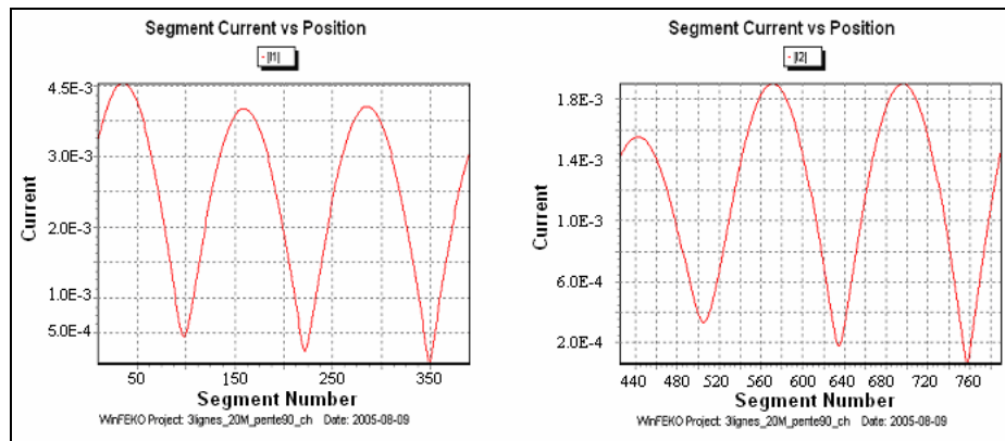
Figure III-39 : Distribution de courant – réseau complexe (module) théorie des antennes "FEKO" ( F = 12 MHz, L = 3 \cdot 10 m, h \neq cte, diamètre = 2 mm, d = 10 cm)
