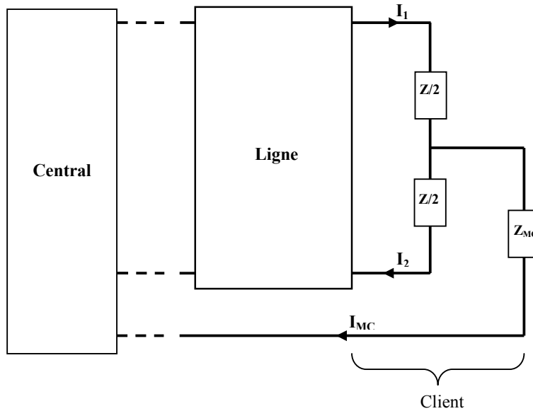
Figure IV-36: Schéma du dispositif d'adaptation simulé
