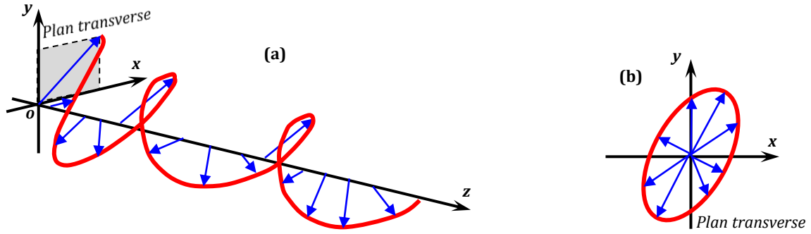
Figure 2.1. État de polarisation d'une vibration lumineuse suivant (a) le plan de propagation et (b) le plan transverse
