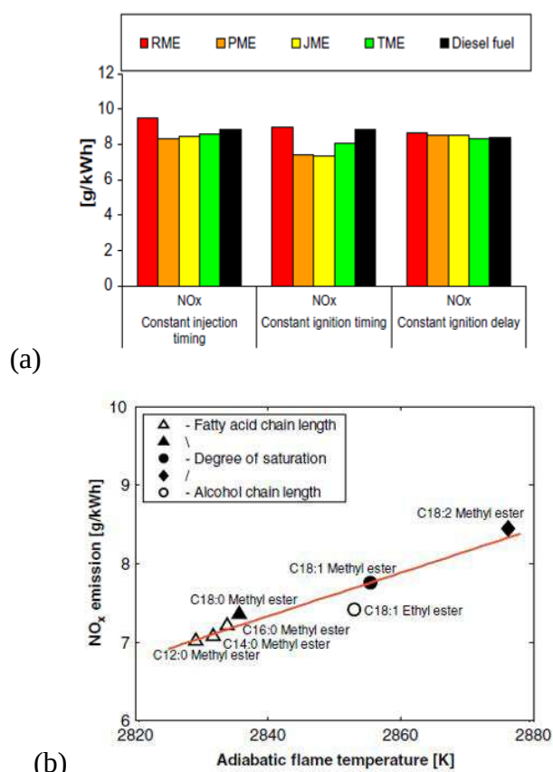
Figure 22. Emission de NOx (a) pour un gazole fossile et quatre différents types de bio-Diesel : ester méthylique d'huile de palme (PME), ester méthylique d'huile de jatropha (JME), ester méthylique de suif (TME) et ester méthylique d'huile de colza (RME) et (b) en fonction de la température de flamme adiabatique de différents esters d'acides gras. Schönborn 2009
