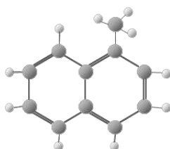
Figure 27. Molécule d'1-méthylnaphtalène
