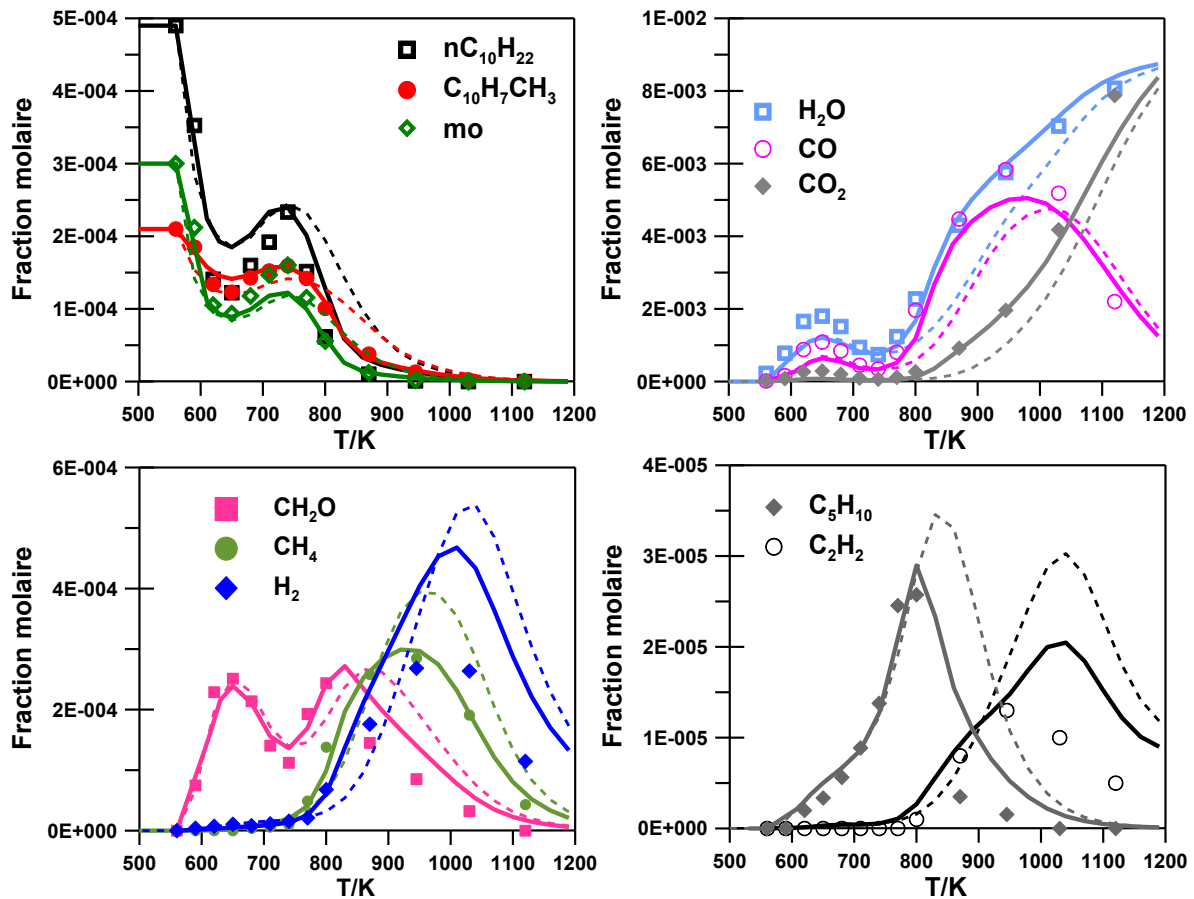
Figure 87. Oxydation du carburant modèle B30 en JSR : P = 10 bar, \tau = 1 s et \phi = 1 . Symboles: résultats expérimentaux. Lignes continues: mécanisme modifié, Lignes en pointillées: mécanisme précédent.
