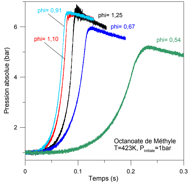
Figure 110. Evolution de la pression en fonction du temps de l'octanoate de méthyle pour un intervalle de rapports d'équivalence de 0,54 à 1,25.
