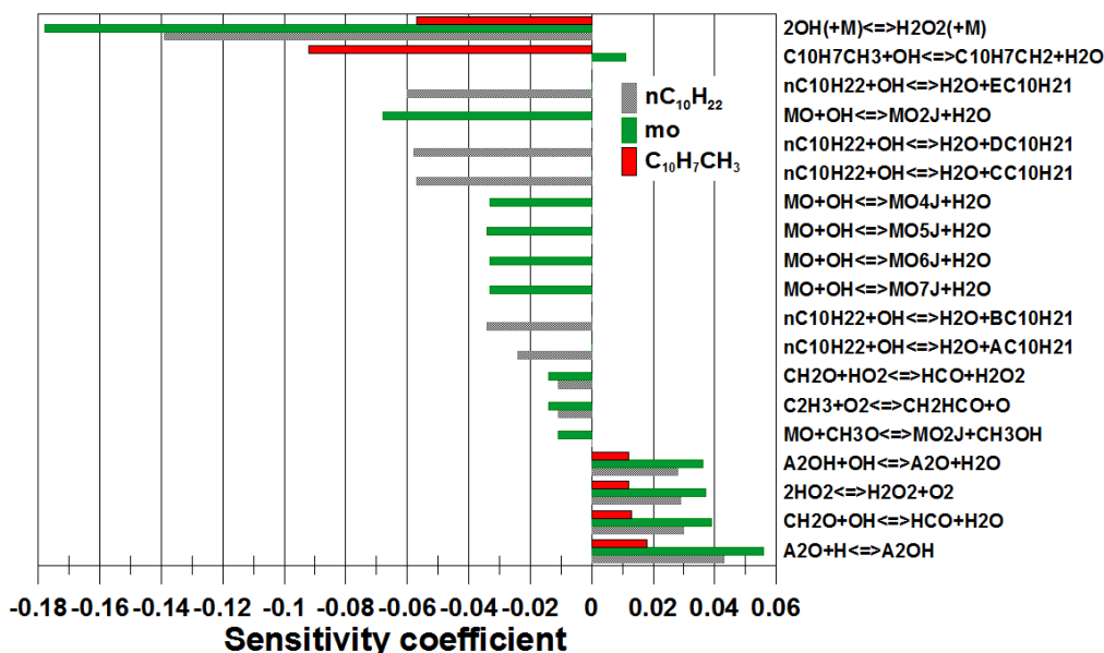
Figure 97. Analyse de sensibilité pour le B30 modèle à 910 K, \phi = 1 , 20 bar et une consommation de 21,69% du 1-méthyl-naphtalène, de 76,09% du n -décane et de 64,14% de l'octanoate de méthyle.
