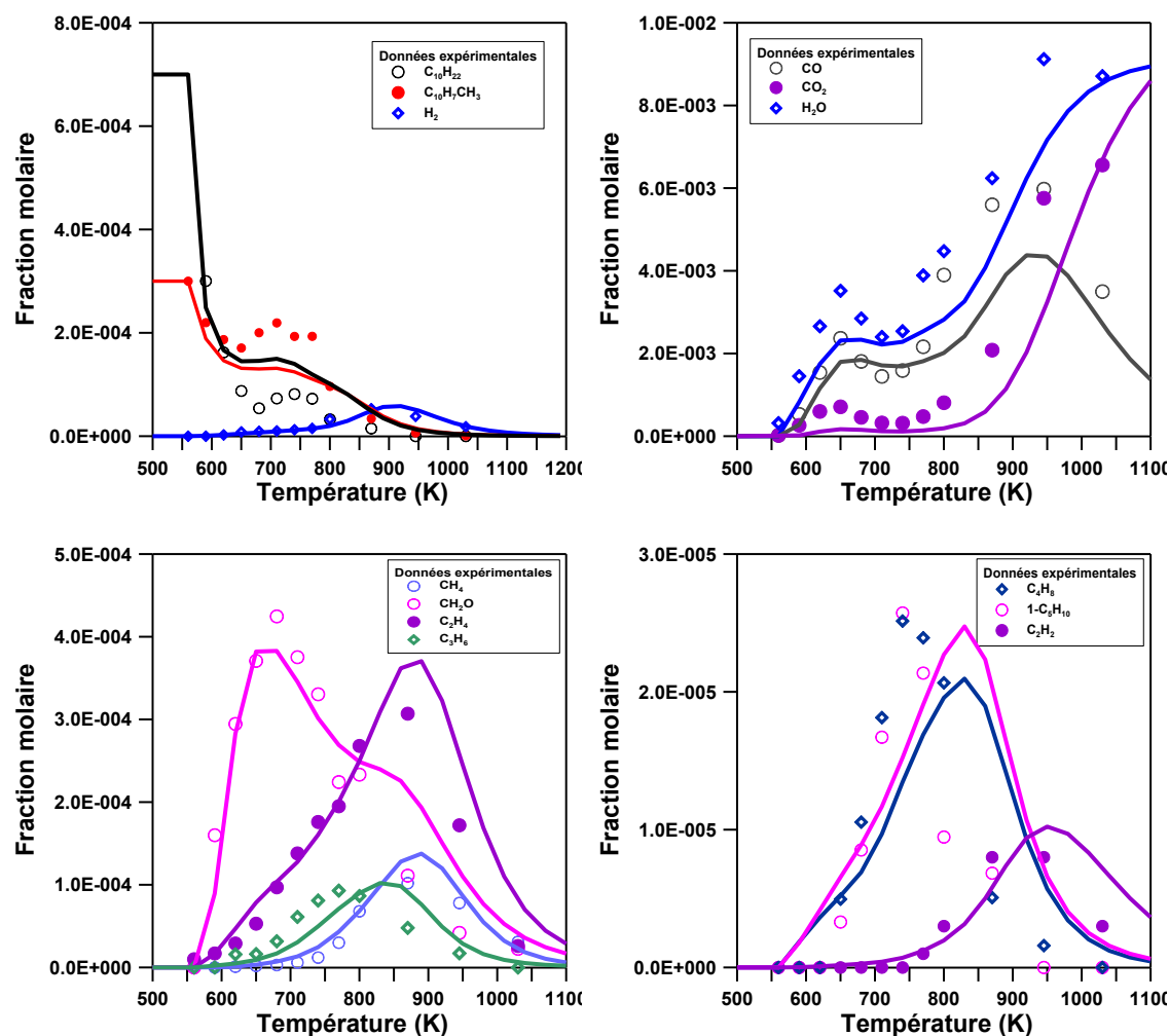
Figure 64. Confrontation du modèle (lignes) avec les expériences (symboles) lors de l'oxydation d'un carburant réel type gazole en JSR : \phi=0.25 , 10bar et \tau=1s . Les incertitudes estimées sont de l'ordre de \pm 10\% .
