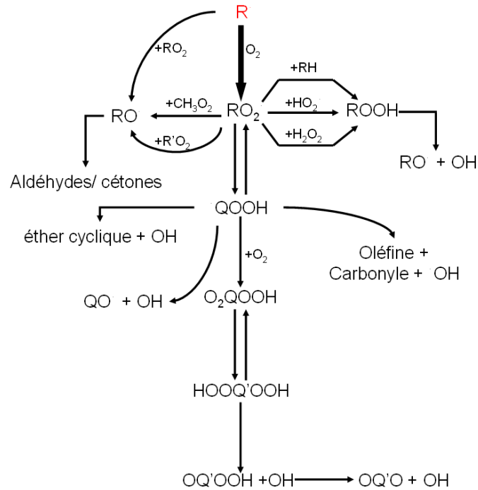
Figure 23. Voies de réaction à base température (Griffiths et al. 1995).
