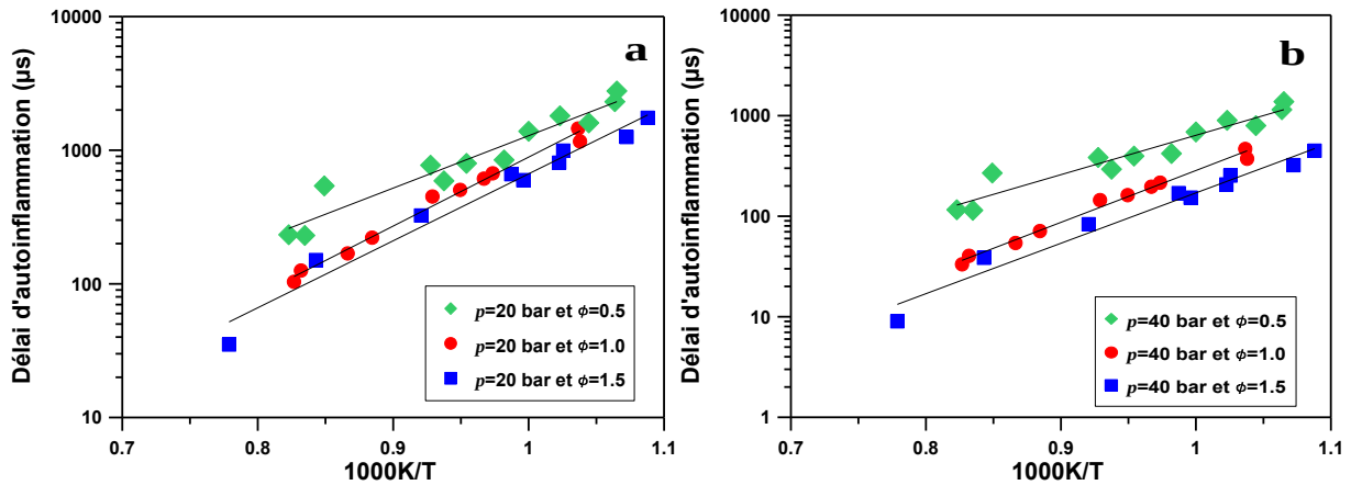
Figure 84. Délais d'auto-inflammation normalisés pour le carburant modèle B30 dans l'air à \phi=0,5 (losanges), \phi=1,0 (cercles) et \phi=1,5 (carrés), et deux différents pressions 20 bar (a) et 40 bar (b). Les lignes correspondent aux corrélations d'Arrhenius.
