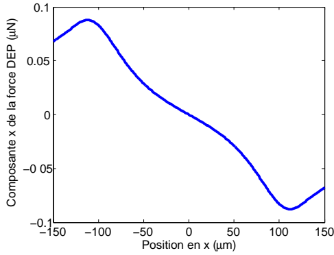
(a) Composante x de la force de diélectrophorèse calculée tout au long de l'axe ( y = 0, z = 50\mu m ) en appliquant une tension égale à U = [75V, 0, 75V] .
