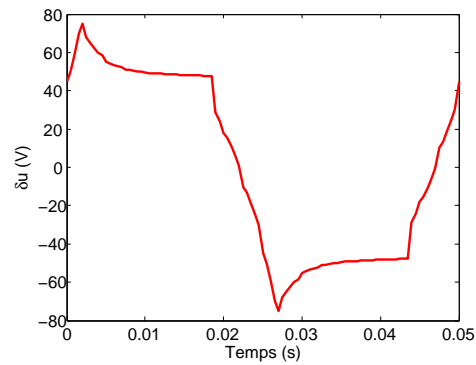
(b) La tension \delta u calculée pour le suivi d'une trajectoire sinusoïdale de période égale à 50\text{ms} dans la zone non-linéaire.
