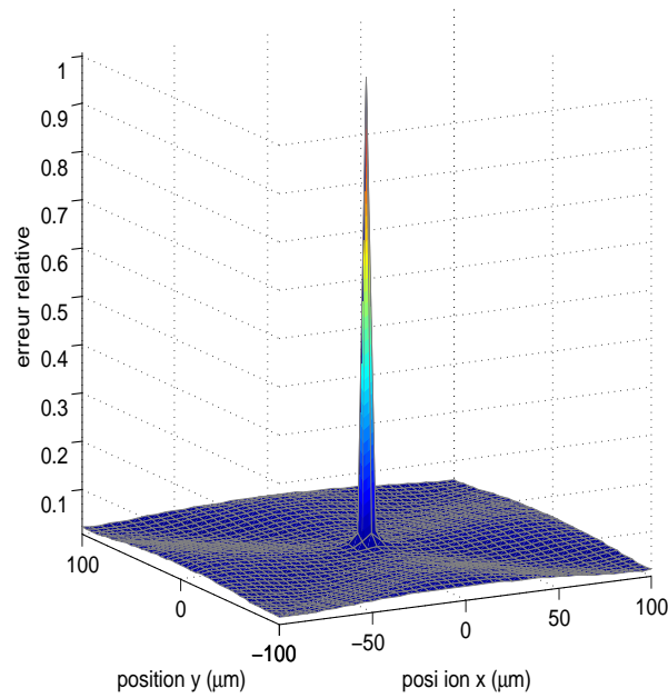
FIGURE 3.7 – Erreur relative du module de la force de diélectrophorèse calculée en considérant que la particule est élémentaire et la force de diélectrophorèse calculée en considérant que la particule est volumique.
