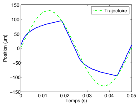
(a) Le suivi d'une trajectoire sinusoïdale de période égale à 50\text{ms} et d'amplitude égale à 130\mu\text{m} . La commande se fait dans une zone fortement non-linéaire.
