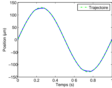
(a) Le suivi d'une trajectoire sinusoïdale de période égale à 1\text{s} et d'amplitude égale à 130\mu\text{m} . La commande se fait dans une zone fortement non-linéaire.
