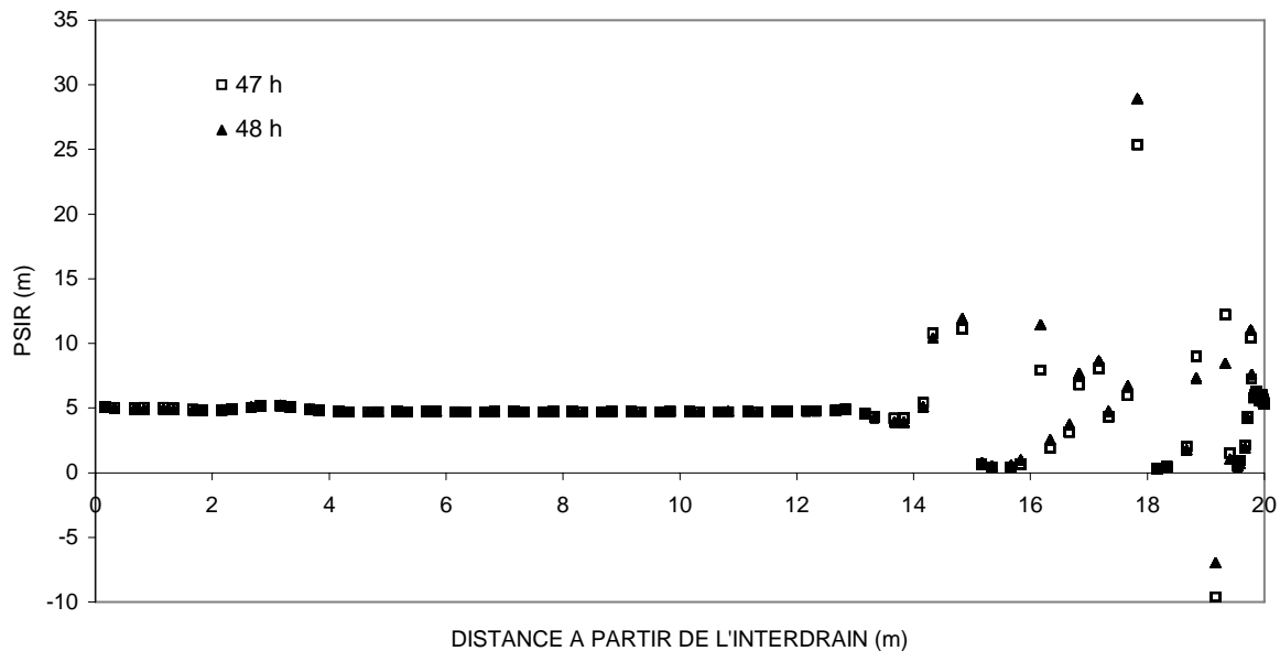
Figure 3-4 : Amplification des divergence de \Psi_r entre deux intervalles de temps.
