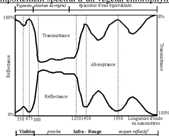
Figure 38: Comportement spectral d'un végétal chlorophyllien
