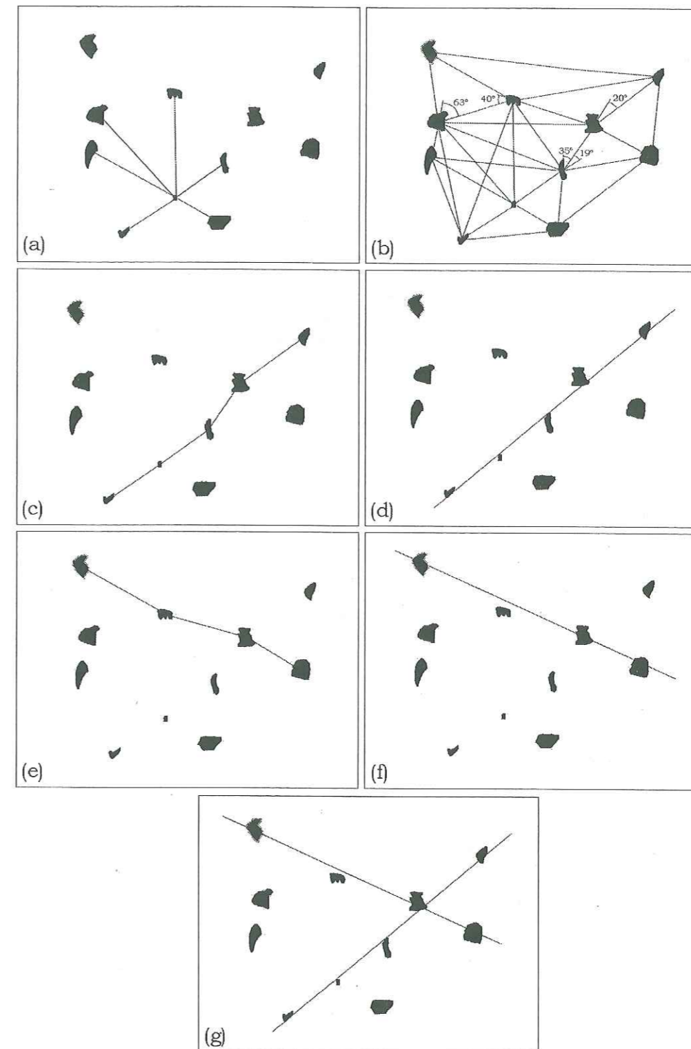
Figure III-10 Etapes de la méthode selligne utilisée pour déterminer un linéament. (a), connexion entre un diapirs et ses voisins (affleurants et non affleurants) par des lignes directes ; (b), réseau complet ; (c), choix d'une direction d'affleurement NE-SW avec écart \leq 20^\circ ; (d), linéament proposé pour l'exemple (c) ; (e), choix d'une autre direction WNW-ESE avec écart \leq 20^\circ ; (f), linéament proposé pour l'exemple (e) ; (g), Ensemble des linéaments retenus. Dans cet exemple, la présence d'un minimum de quatre affleurements de sel était requise pour la définition d'un linéament.
