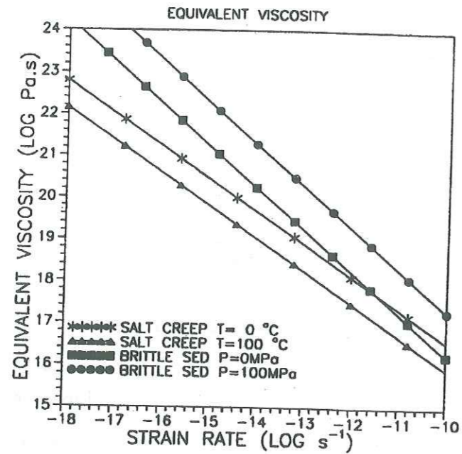
Figure I-16 Relation entre viscosité du sel et des sédiments non-évaaporites et la vitesse de déformation [Daudré & Clottingh, 1994]. La vitesse de la déformation augmente lorsque la viscosité diminue.
