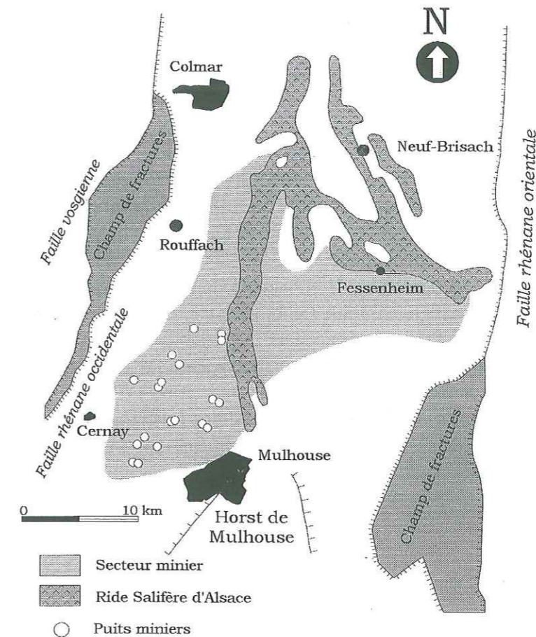
Figure II-3 Forme et position géographique de la ride salifère et des secteurs miniers d'Alsace.
