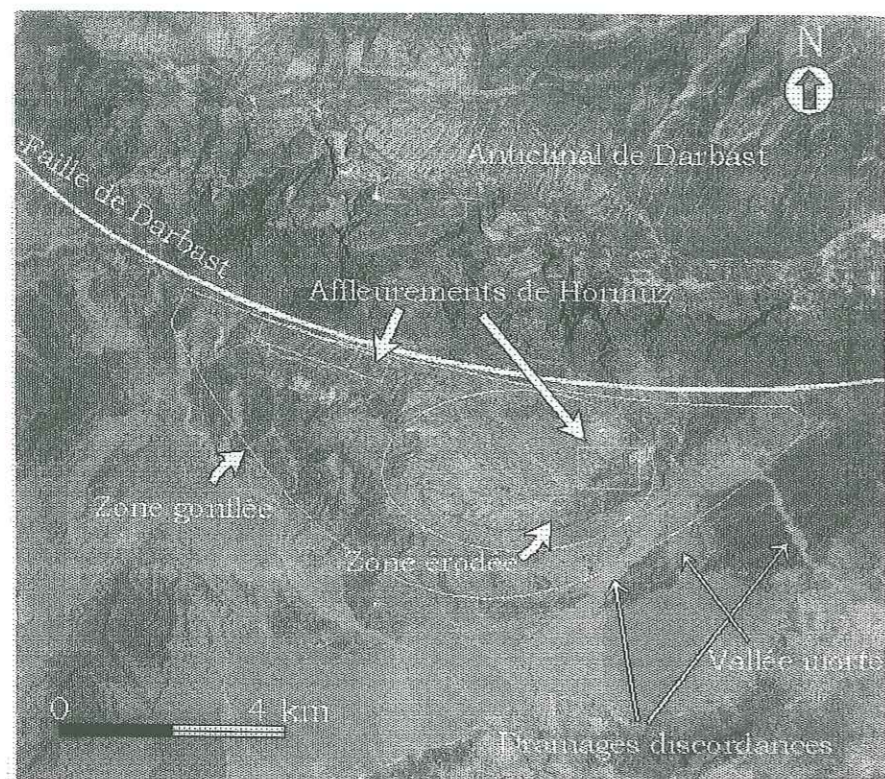
Figure III-146 Image SPOT du site de Darbast. Drainages ramifiés, vallée morte et zone d'inflation sont représentés sur la Figure.
