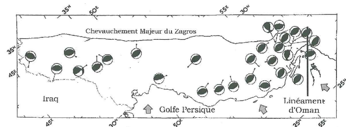
Figure III-24 Mécanismes aux foyers des séismes montrant la présence de chevauchements de fort pendage parallèles au chevauchement majeur du Zagros [Jackson, 1980 ; modifiée].
