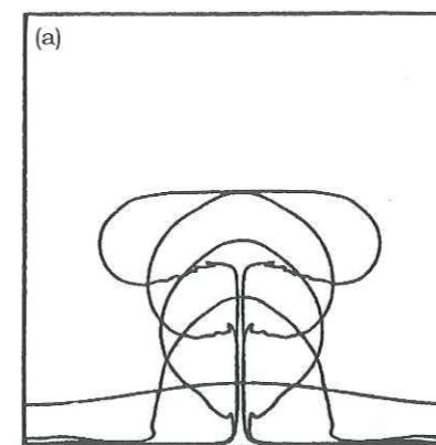
Figure I-15 Influence de la densité de la couverture sur la forme du diapir dans un modèle réalisé par Rômer & Neugebauer (1991).
