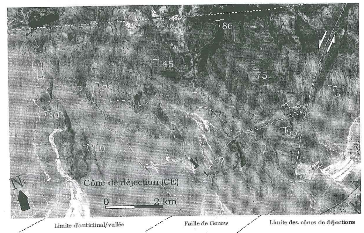
Figure III-77 Partie SE de l'anticlinal de Genow. Limite des cônes de déjection et zone supposée de l'activité de diapir représentée sur la Figure. Voir la localisation de cet extrait de scène SPOT sur la Figure III-70-c.
