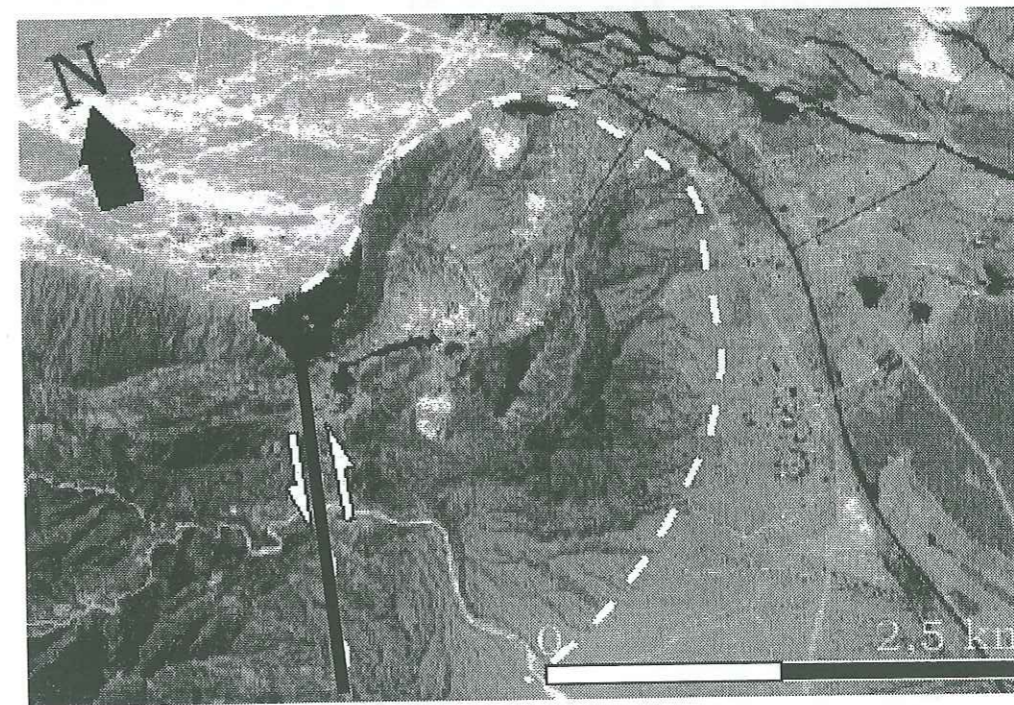
Figure III-74. Partie Est de l'anticlinal de Genow et terminaison de la faille de Genow. La courbure de la terminaison périantyclinale de Genow (ligne tiretée blanche) ainsi que la localisation de la faille de Genow (ligne noire) est représentée sur l'image. Les taches noires sont les terrains cultivés et les maisons. L'affleurement de Hormuz est si petit qu'il n'est pas visible sur l'image. Voir la localisation de cet extrait de scène SPOT sur la Figure III-70-b.
