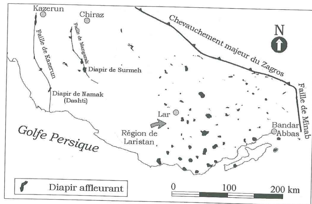
Figure III-4 Carte des affleurements de diapirs de la série de Hormuz au Zagros.
