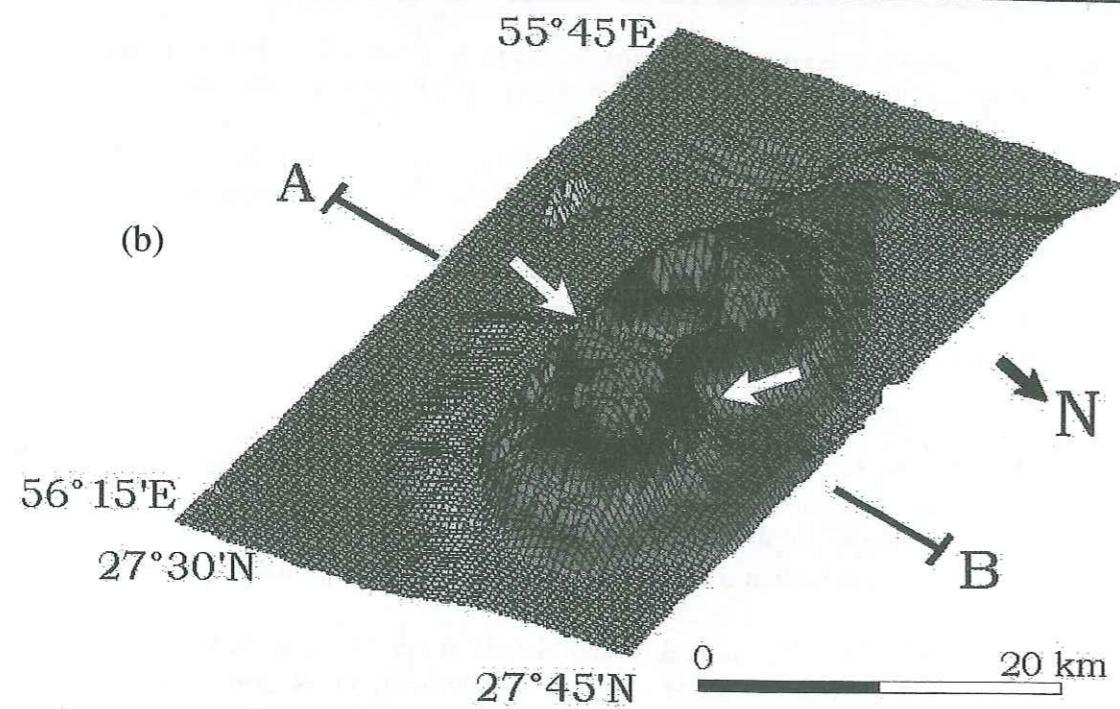
Figure III-128 Déflation de l'anticlinal de Handan. (a), extrait de scène SPOT. La ligne tiretée noire est la limite actuelle de l'anticlinal et la ligne tiretée blanche est la limite reconstituée de l'anticlinal avant la subsidence. Les taches noires, au centre de l'anticlinal, correspondent aux affleurements de sel ; (b), modèle numérique de terrain du site de Handan illustrant une déflation de la surface. Les flèches blanches indiquent la direction de subsidence.
