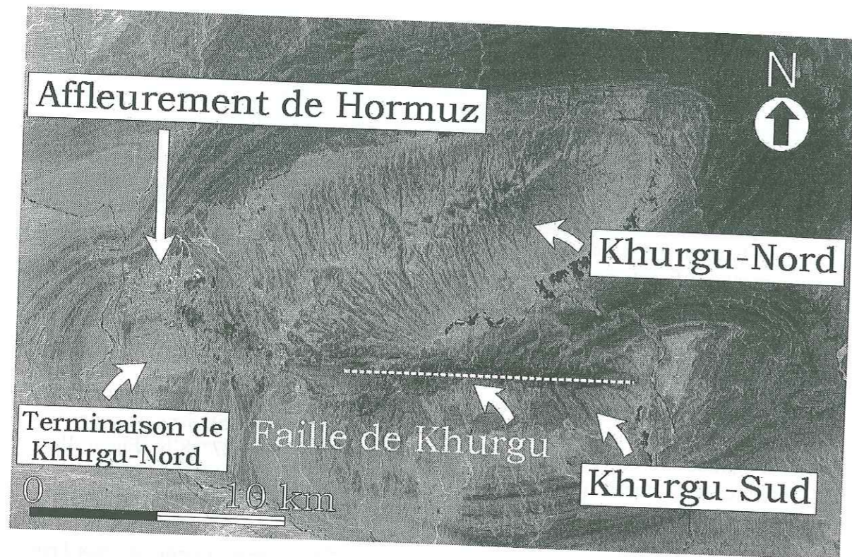
Figure III-83 Site de Khurgu (extrait de scène SPOT). Les anticlinaux de Khurgu-Nord et de Khurgu-Sud, la faille principale de Khurgu (E-W) et l'affleurement de la série de Hormuz sont visibles sur la Figure.
