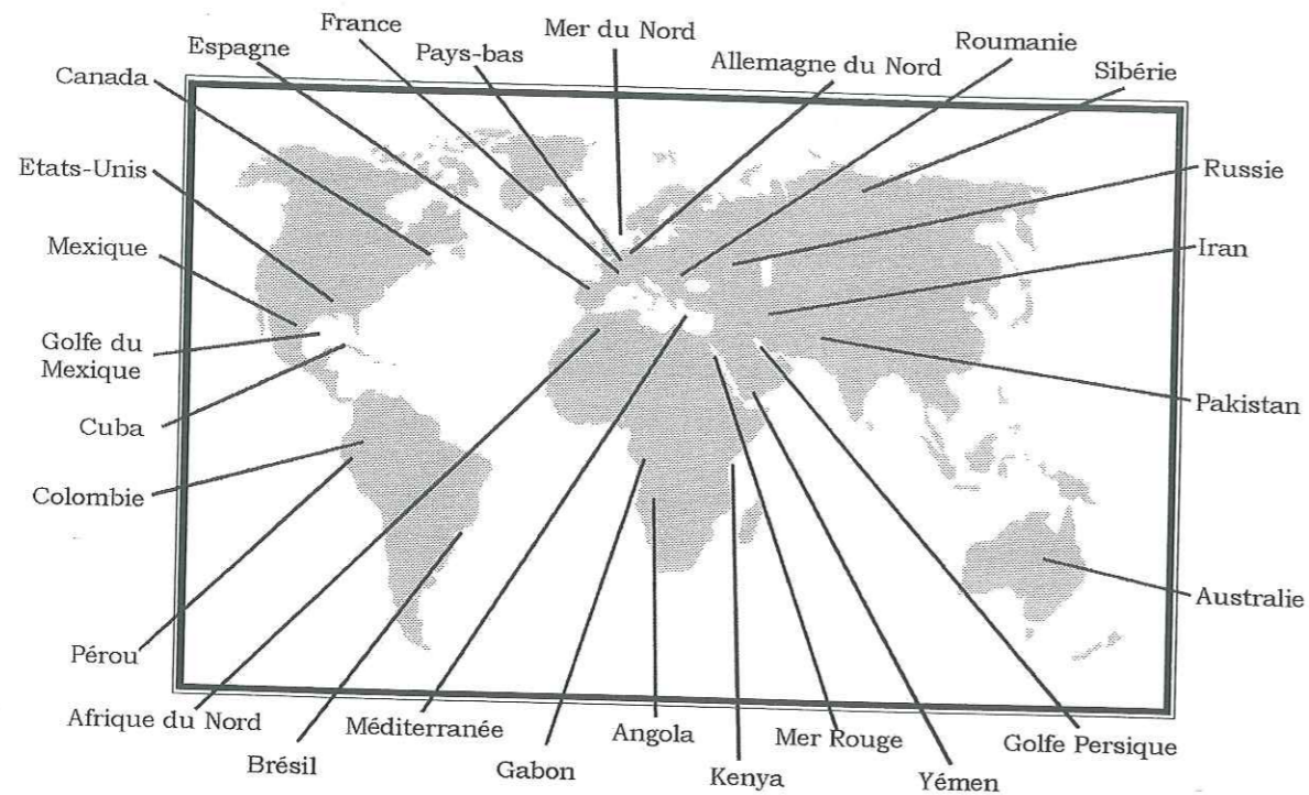
Figure I-1 Répartition des principaux gisements de sel dans le monde. Les plus connus sont les gisements du golfe du Mexique et du sud des Etats-Unis, d'Allemagne du Nord, de la mer du Nord, du golfe Persique et de l'Iran.
