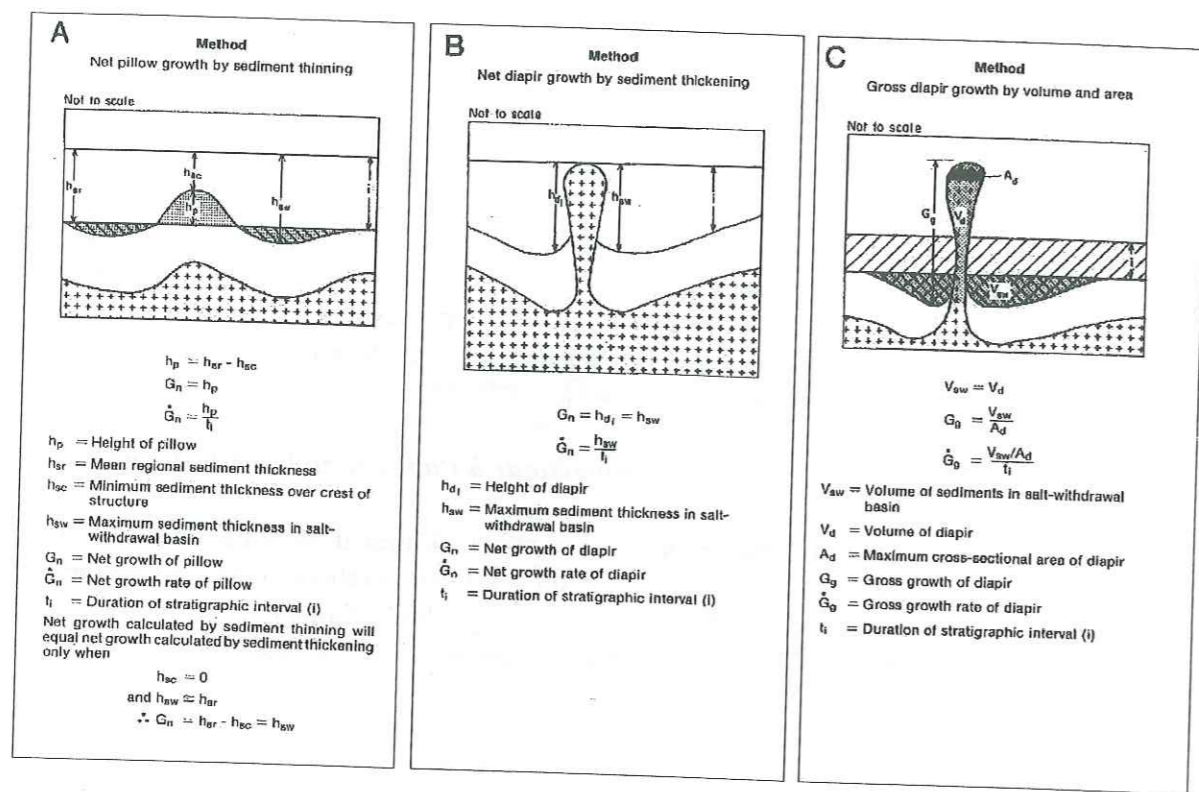
Figure I-29 Trois modèles proposés par Seni & Jackson (1984) pour estimer la vitesse de mouvement vertical des masses salifères. Pour pouvoir appliquer cette méthode, il est nécessaire de convertir en coupe profondeur les sections sismiques qui seules, permettent simplement d'imager la structure diapirique. (A), premier modèle pour estimer la vitesse de mouvement des rides salifères et des diapirs en phase immature (non-pénétrant). Cette méthode est valable pour une masse de sel dans l'étape d'évolution d'intumescence salifère. Dans ce modèle, on calcule le soulèvement du sel grâce aux paramètres détaillés ci-dessus et à la relation G_n = h_p . La vitesse de soulèvement du dôme de sel ( \dot{G}_n ) s'estime en datant les couches sus-jacente (i) : \dot{G}_n = h_p/t_i ; (B), deuxième modèle pour estimer la vitesse de mouvement vertical des rides salifères. Cette méthode est valable dans le cas d'un dôme de sel en phase mature et pénétrant. Dans ce modèle, le soulèvement de la masse de sel a provoqué un synclinal dans les couches sédimentaires autour du dôme de sel. On estime les paramètres marqués ci-dessus et la vitesse ascensionnelle est estimée en utilisant la formule \dot{G}_n = h_{sw}/t_i ; (C), troisième modèle pour estimer la vitesse de mouvement vertical des dômes de sel. Cette méthode est applicable dans le cas d'une masse de sel en phase mature, pénétrant et affleurant à la surface. Dans ce modèle, le soulèvement de la masse de sel est calculé à partir de la mesure de la surface d'affleurement de sel ( A_d ) et du volume de diapir ( V_d ) ou du volume du synclinal autour de dôme de sel ( V_{sw} ). On estime la vitesse de soulèvement de dôme de sel en ayant les âges de sédimentation ( t_i ) des couches sus-jacentes par la formule : \dot{G}_g = (V_{sw}/A_d)/t_i .
