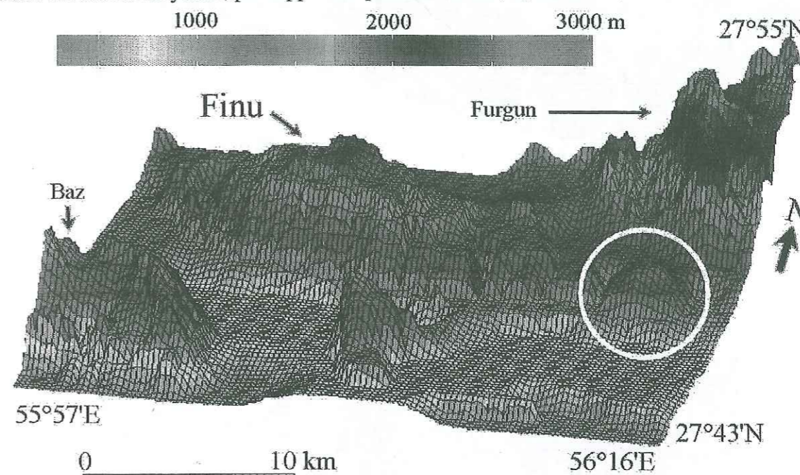
Figure III-55 Morphologie du site de Finu en vue perspective. La position de l'affleurement de sel est encadrée.
