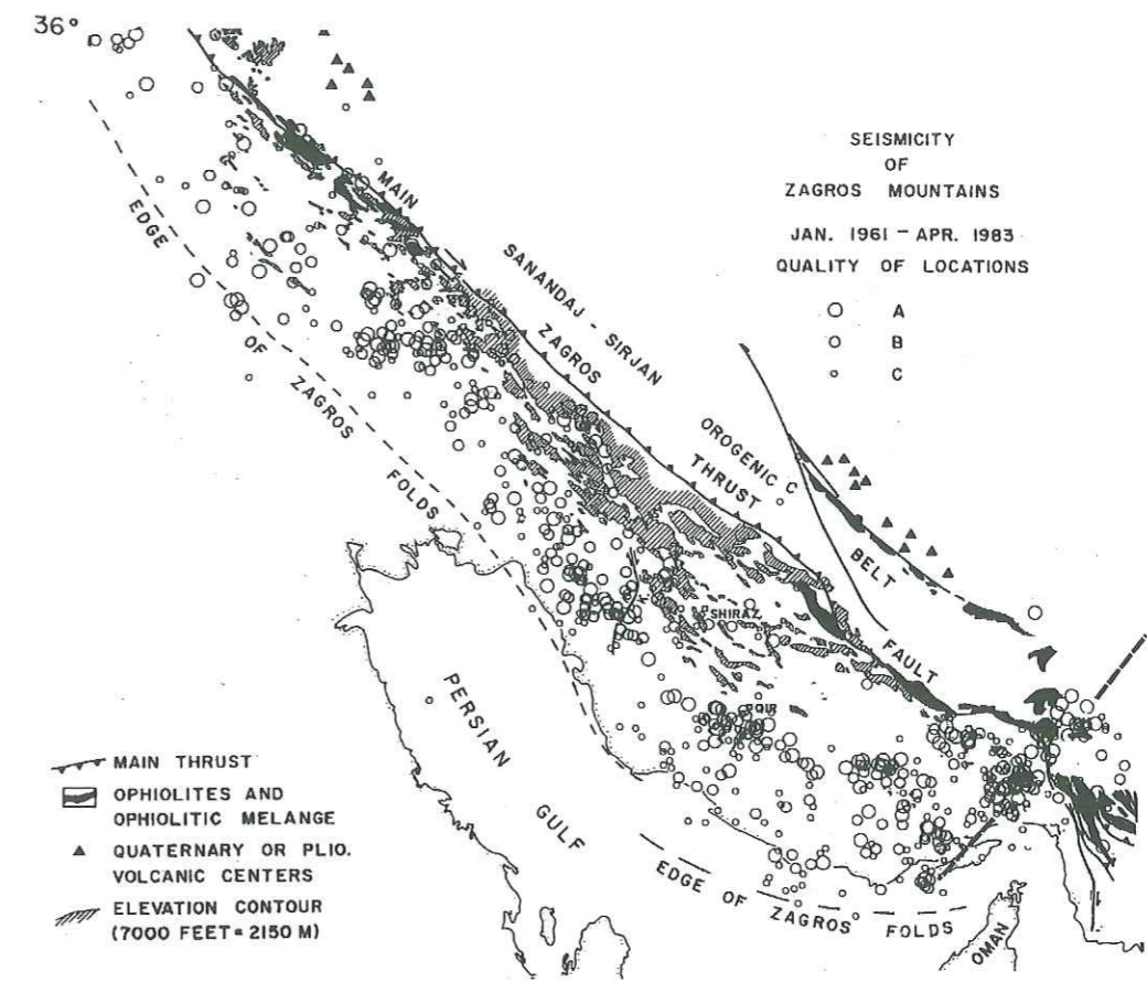
Figure III-23 Topographie supérieure à 2000 m et épicentres des séismes de 1961 à 1983 [Ni & Barazangi, 1986 ; modifiée].
