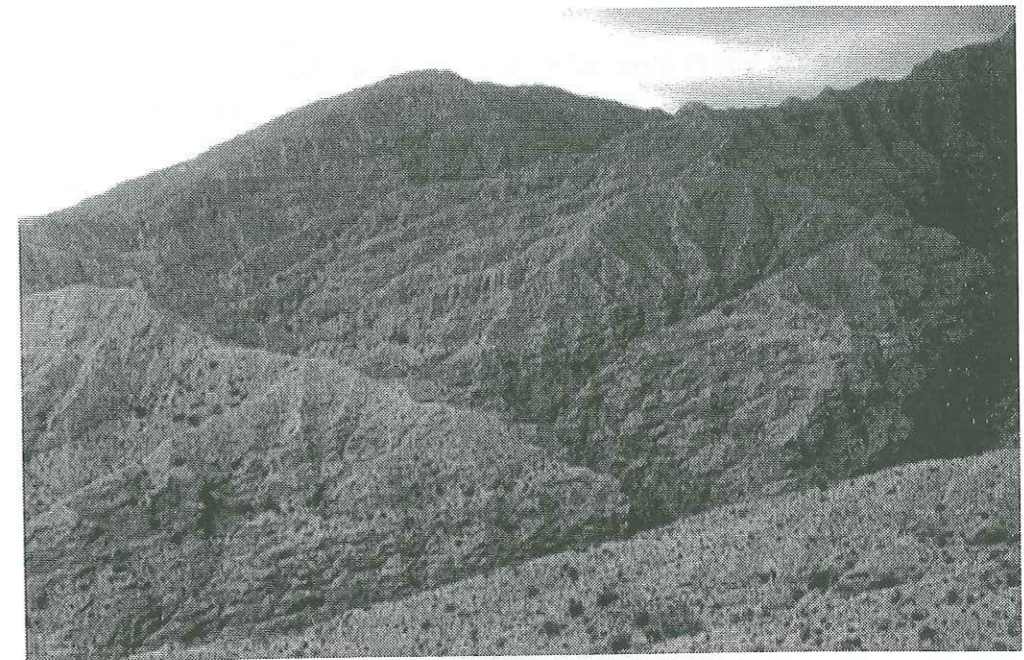
Figure III-76 Formation de Bakhtiyarie et ses vallées encaissées à l'Ouest de la faille de Genow.
