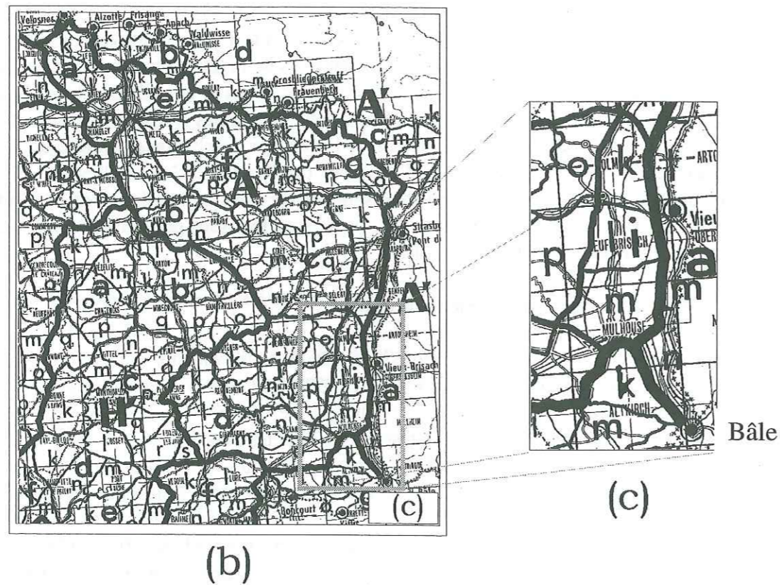
Figure II-8 (a), Réseau de nivellement IGN en France (Levallois & Maillard, 1970); (b), réseau de nivellement au Nord-Est de la France (maille 'A'); (c), agrandissement de notre réseau de nivellement (mailles 'Alk', 'Ali' et 'Alm').
