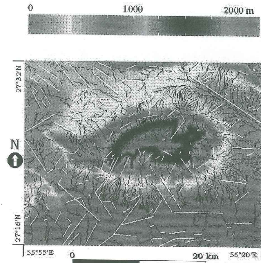
Figure III-108 Superposition du réseau hydrographique du site de Genow à son MNT d'altitude. Les anomalies hydrographiques sont représentées par les lignes blanches.
