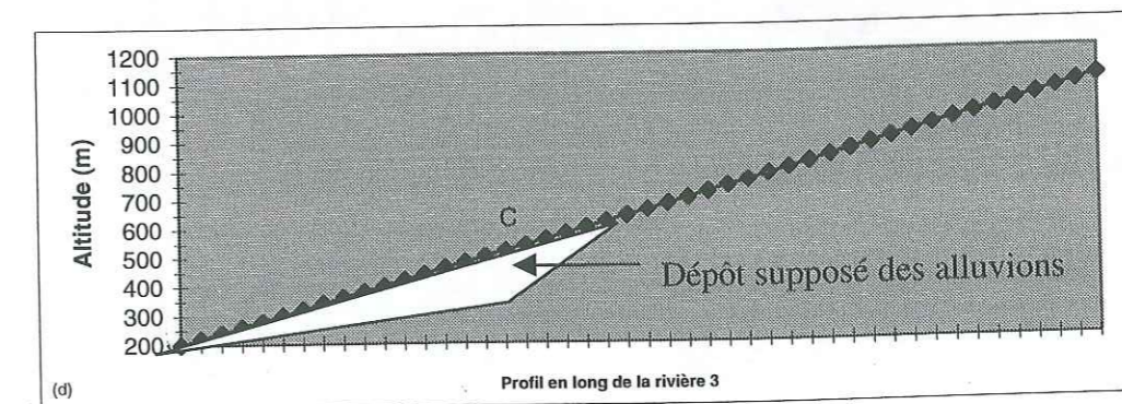
Figure III-78 Profils en long de trois rivières (1 à 3) sur le flanc Sud de l'anticlinal de Genow. (a), rivières sélectionnées ; (b) et (c), profils en long des rivières 1 et 2 montrant une rupture de pente à la limite sud de Genow ; (d), profil en long de rivière 3 ne montrant pas de rupture de pente à la limite anticlinal/vallée. Le dépôt supposé des alluvions est représenté sur le profil.
