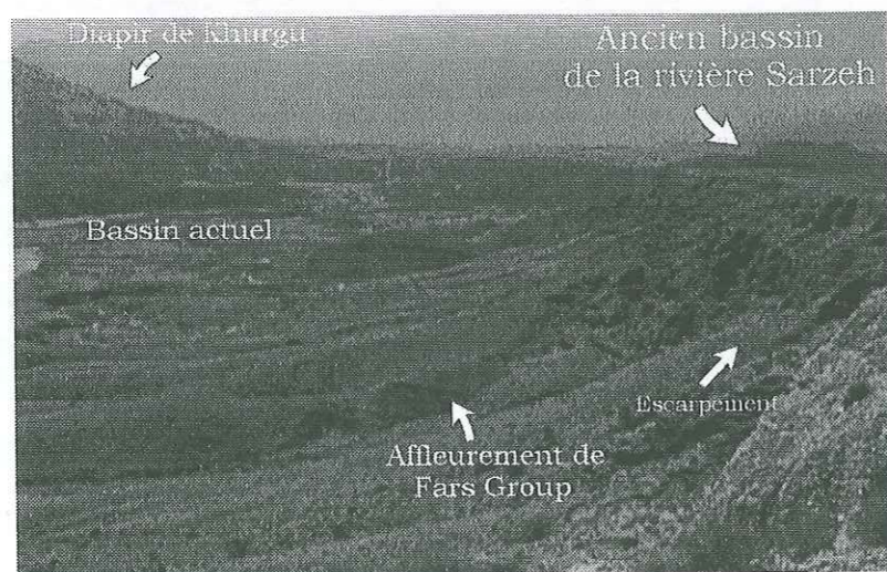
Figure III-144 Cours actuel de la rivière Sarzeh. L'escarpement burdier au N du bassin résulte de l'érosion des couches du Fars Group.
