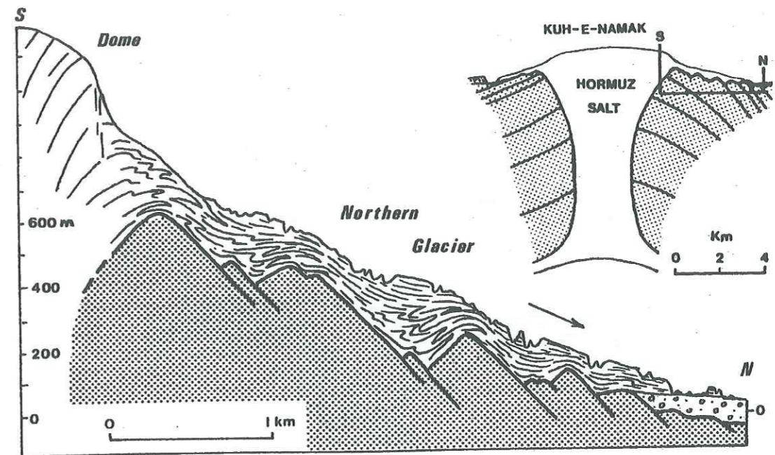
Figure I-9 Coupe du diapir de Kuh-e Namak (Iran) et du glacier de sel situé au nord de celui-ci [Talbot, 1979].
