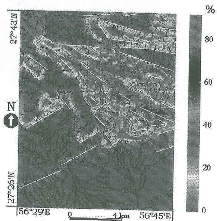
Figure III-107 Superposition du réseau hydrographique du site de Darbast à son MNT de pente. Les anomalies hydrographiques sont représentées par les lignes blanches.
