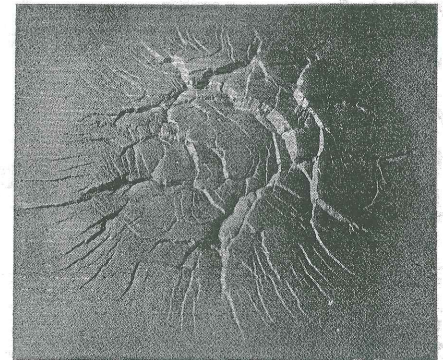
Figure I-24 Système de fracturation radial sur un modèle analogique à couverture d'argile [Lowell, 1985]. Dans ce modèle, la force verticale vient du gonflement d'un ballon.
