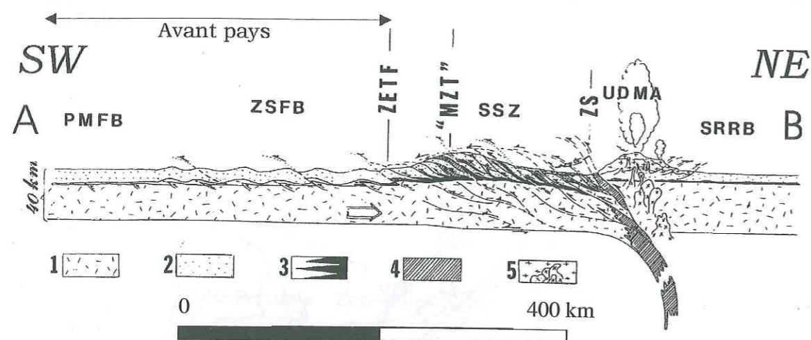
Figure III-21 Coupe crustale schématisique perpendiculaire à la direction des plis du Zagros [Alavi, 1994]. PMFB (Persian Gulf-Mesopotamian Foreland Basin), bassin mésopotamien du golfe Persique ; ZSFB (Zagros Simply Folded Belt), chaîne de simples plissements du Zagros ; ZETF (Zagros Exposed Thrust Front), front de chevauchement exposé du Zagros ; MZT (Main Zagros Thrust), chevauchement majeur du Zagros ; SSZ (Sanandaj-Sirjan Zone), zone de Sanandaj-Sirjan ; ZS (Zagros Suture), suture du Zagros ; UDMA (Uremieh-Dokhtar Magmatic Zone), zone magmatique d'Urmia-Dokhtar ; SRRB (Saveh-Rafsanjan Retroarc Basin), Iran Central ; 1, croûte continentale ; 2, sédiments phanérozoïques ; 3, évaporite et dolomite à la base de la couverture sédimentaire ; 4, croûte océanique ; 5, intrusion et extrusion de roches magmatiques.
