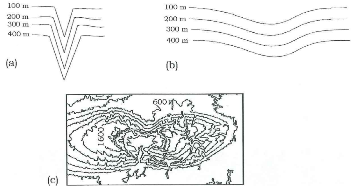
Figure III-129 Forme des courbes de niveau dans une zone d'érosion et dans une zone de déflation. (a), courbes de niveau résultant d'une érosion locale ; (b), courbes de niveau résultant d'une subsidence locale ; (c), courbes de niveau de l'anticlinal de Handan. Ce dernières ressemblent au cas (b) : déflation locale.
