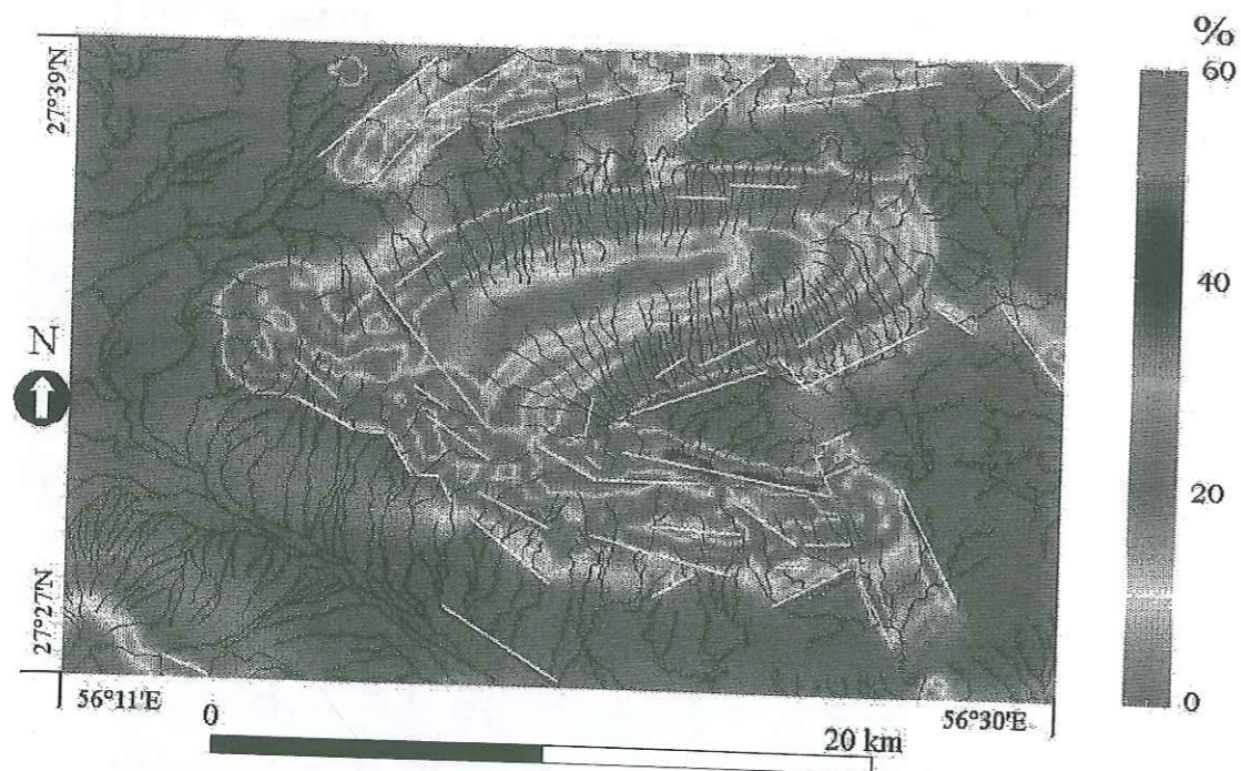
Figure III-111 Superposition du réseau hydrographique du site de Khurgu à son MNT de pente. Les anomalies hydrographiques sont représentées par les lignes blanches.
