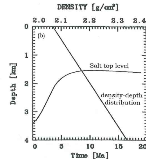
Figure I-15 Influence de la densité de la couverture sur la forme du diapir dans un modèle réalisé par Rômer & Neugebauer (1991).
