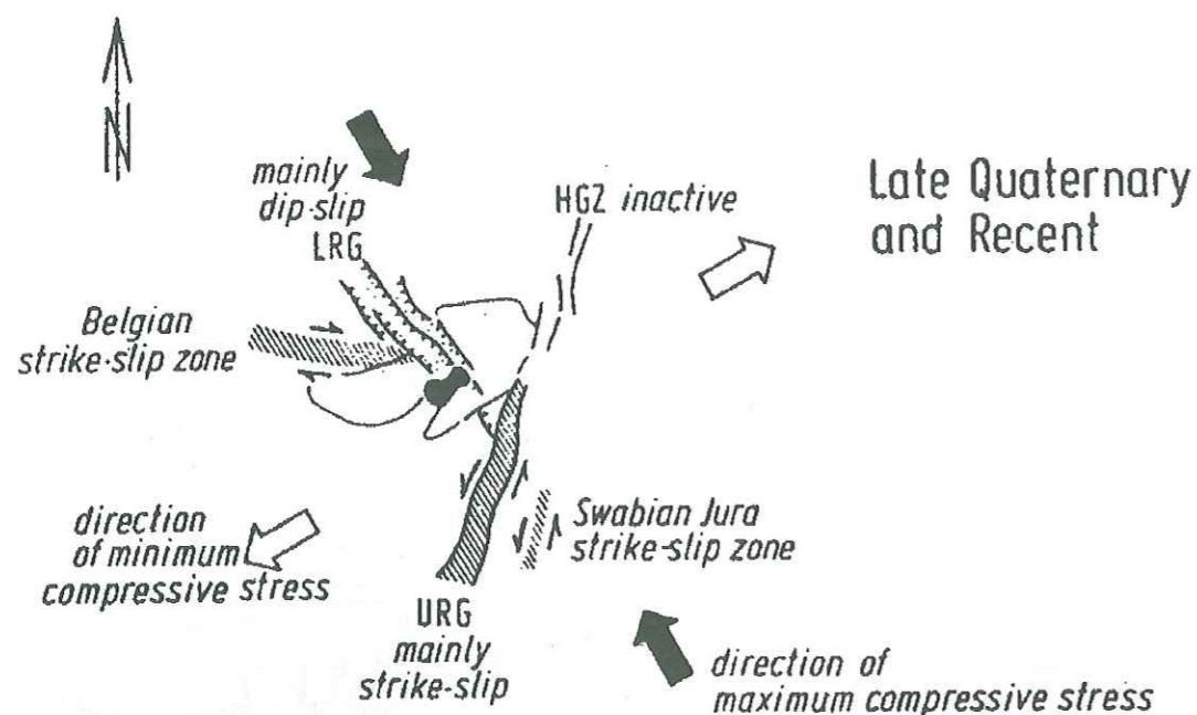
Figure II-6 Direction principale du champ de contrainte actuel dans la région du fossé rhénan [Ahorner, 1975, simplifiée].
