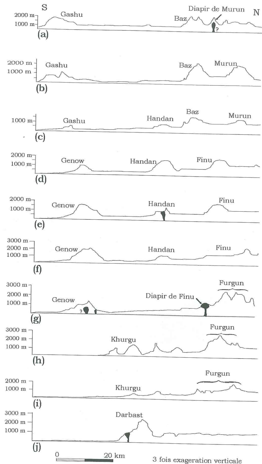
Figure III-51 Dix coupes topographiques (N-S) localisées sur la Figure III-50.
