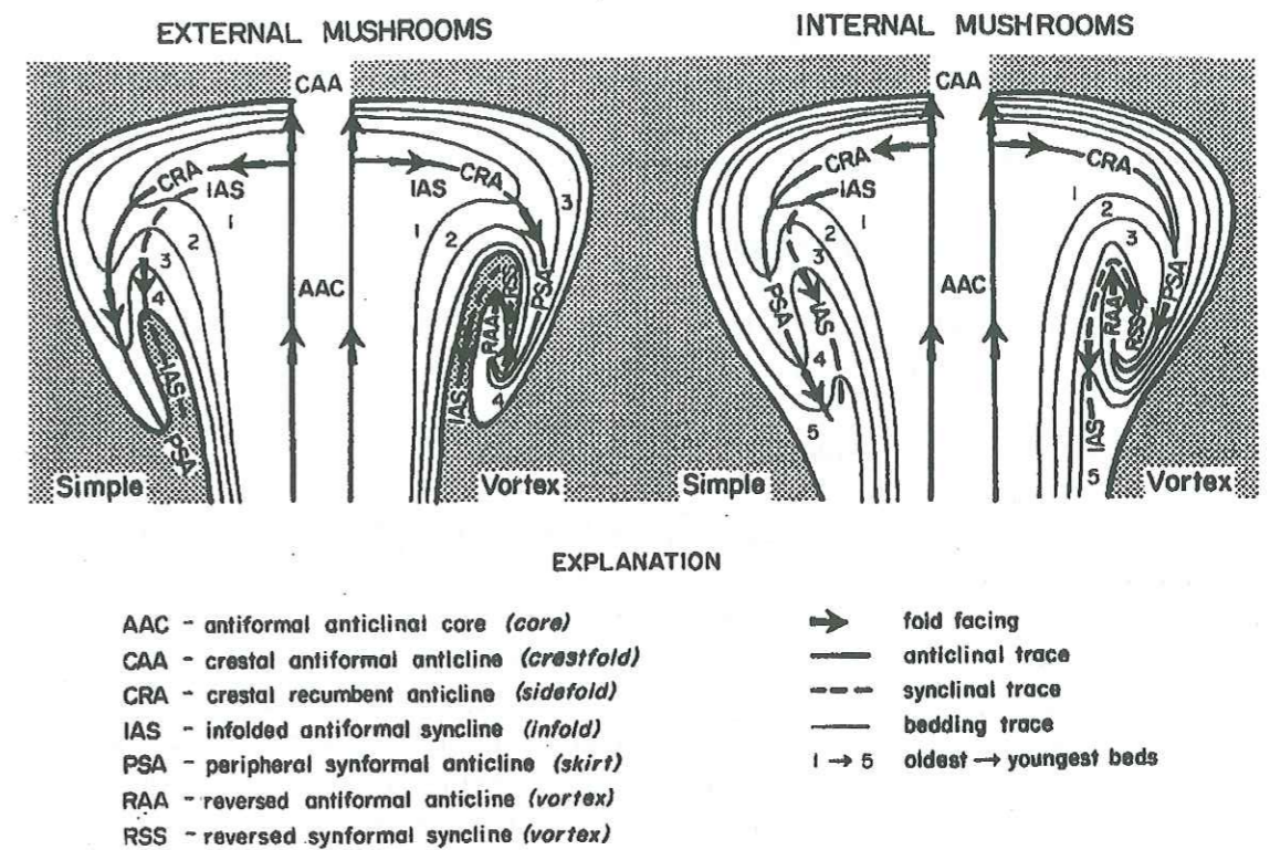
Figure I-11 Schémas structuraux de deux diapirs d'anatomies simples et présentant un vortex, réalisés par centrifugation [Jackson & Talbot, 1989]. Le cheminement du mouvement de sel à l'intérieur de diapir est représenté par les flèches.
