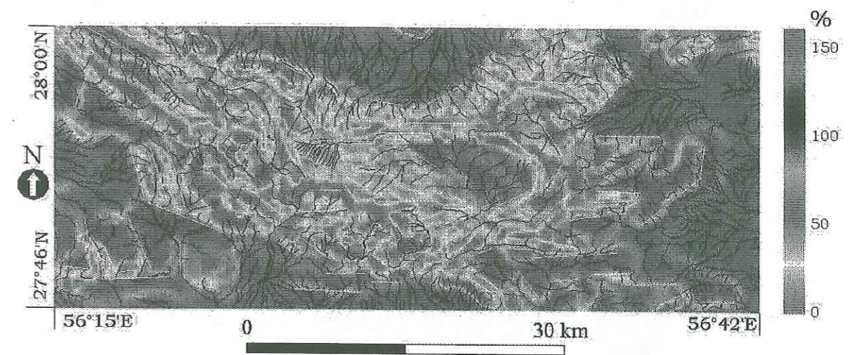
Figure III-105 Superposition du réseau hydrographique de la zone de Furgun à son MNT de pente. Les anomalies hydrographiques sont représentées par les lignes blanches.
