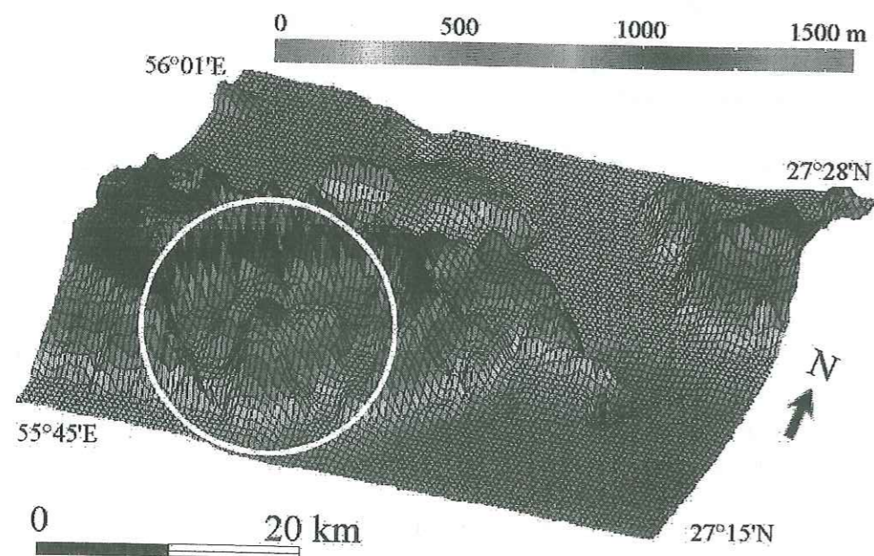
Figure III-54 Morphologie du site de Gashu en vue perspective. La position de l'affleurement de sel de Hormuz est encadrée.
