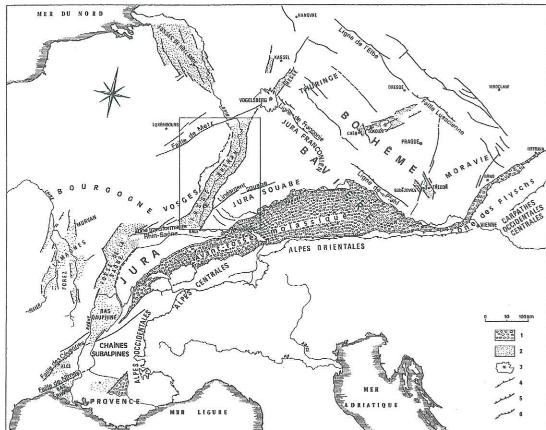
Figure II-1 Rift Ouest-Européen [Bergerat & Geysant, 1980].
