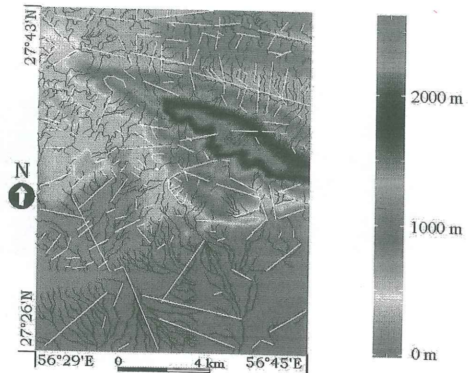
Figure III-106 Superposition du réseau hydrographique du site de Darbast à son MNT d'altitude. Les anomalies hydrographiques sont représentées par les lignes blanches.
