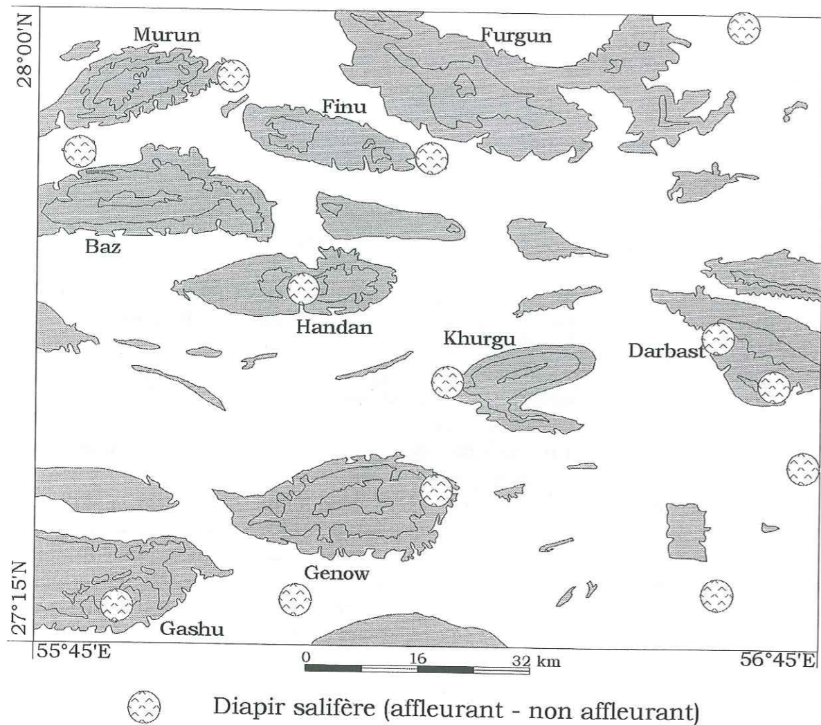
Figure III-89 Positionnement des diapirs (affleurants et non affleurant) de la région de Bandar Abbas. Les noms des anticlinaux sont signalés.
