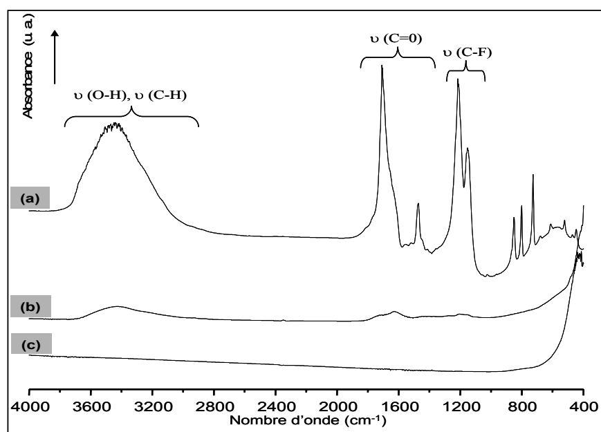
Figure II.38 : Spectres IR de LiGdF 4 (a) xérogel, (b) traité à 300°C et (c) à 500°C sous N 2
