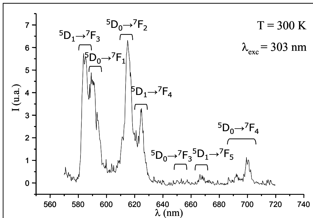
Figure III.6 : Spectre d'émission de LiGdF 4 :Eu 3+ (2%) après excitation à 303 nm ( 8 S 7/2 → 6 P 5/2 ) des ions Gd 3+ enregistré à 300 K
