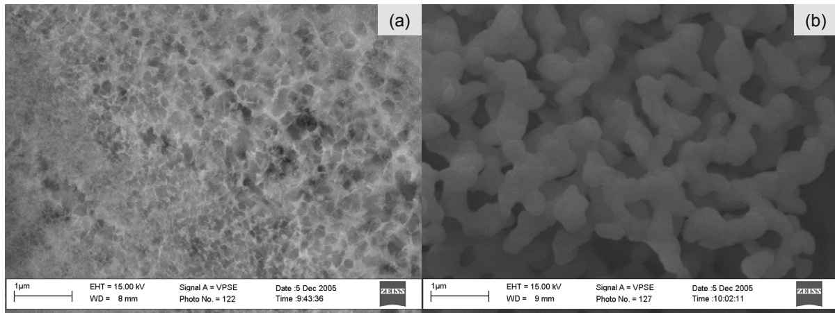
Figure II.31 : Images MEB d'un film \text{LiGdF}_4:\text{Eu}^{3+} (0,5%) déposé par spray (a) non traité et (b) calciné 10h à 550°C sous \text{F}_2 enregistrées avec un agrandissement de 50000X
