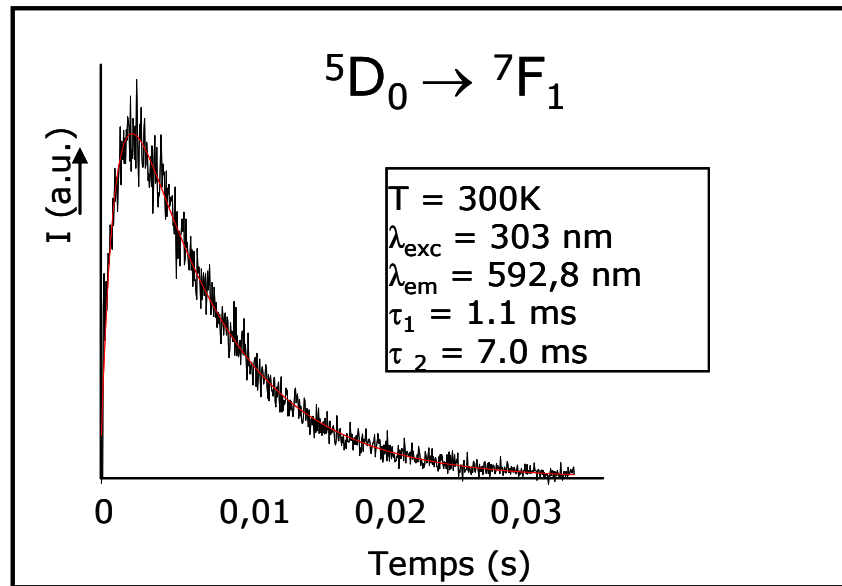
Figure III.7 : Déclin de la fluorescence {}^5\text{D}_0 \rightarrow {}^7\text{F}_1 des ions \text{Eu}^{3+} dans \text{LiGdF}_4:\text{Eu}^{3+} (2%) après excitation du niveau {}^6\text{P}_{5/2} des ions \text{Gd}^{3+}
