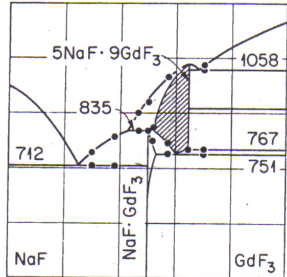
Figure IV.8 : Diagramme de phase du système NaF-GdF 3
