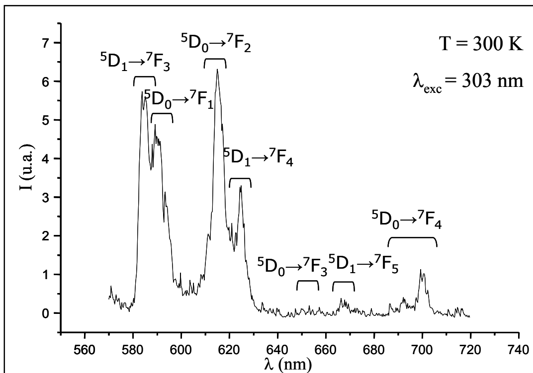
Figure III.6 : Spectre d'émission de \text{LiGdF}_4:\text{Eu}^{3+} (2%) après excitation à 303 nm ( {}^8S_{7/2} \rightarrow {}^6P_{5/2} ) des ions \text{Gd}^{3+} enregistré à 300 K
