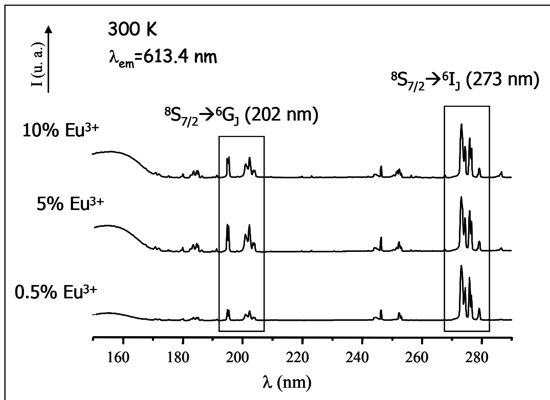
Figure III.11 : Spectres d'excitation enregistrés à 300 K en monitorant la raie d'émission {}^5\text{D}_0 \rightarrow {}^7\text{F}_2 de l'ion \text{Eu}^{3+} pour les composés \text{LiGd}_{1-x}\text{Eu}_x\text{F}_4 ( x = 0,005 ; 0,05 et 0,01 )
