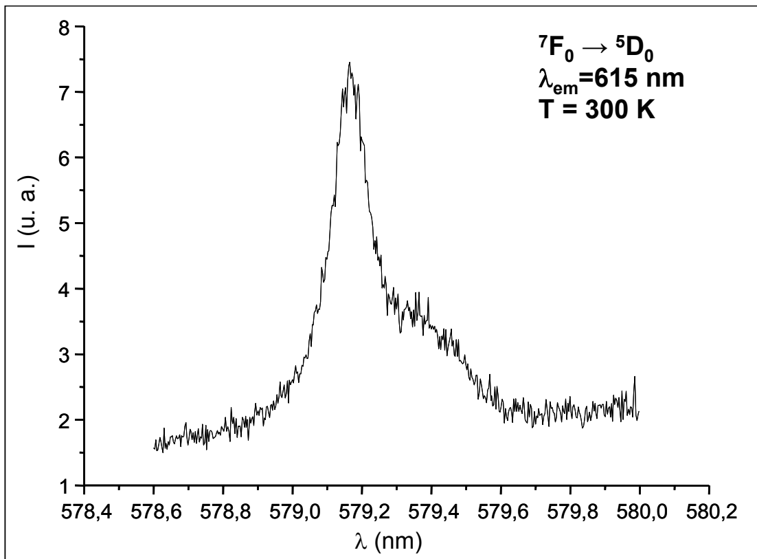
Figure III.20 : Spectre d'excitation {}^7F_0 \rightarrow {}^5D_0 à 300 K de la fluorescence {}^5D_0 \rightarrow {}^7F_2 de l'ion \text{Eu}^{3+} dans la matrice \text{NaGd}_{0,95}\text{Eu}_{0,05}\text{F}_4
