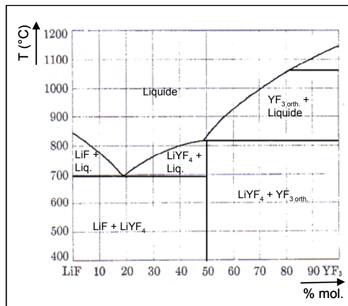
Figure IV.5 : Diagramme de phase du système \text{LiF}-\text{YF}_3
