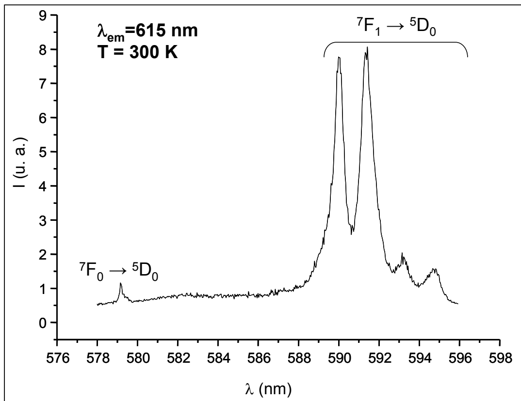
Figure III.19 : Spectre d'excitation de la fluorescence de l'ion \text{Eu}^{3+} dans la matrice \text{NaGd}_{0,95}\text{Eu}_{0,05}\text{F}_4 enregistrés à 300 K en monitorant la transition {}^5\text{D}_0 \rightarrow {}^7\text{F}_2 des ions \text{Eu}^{3+}
