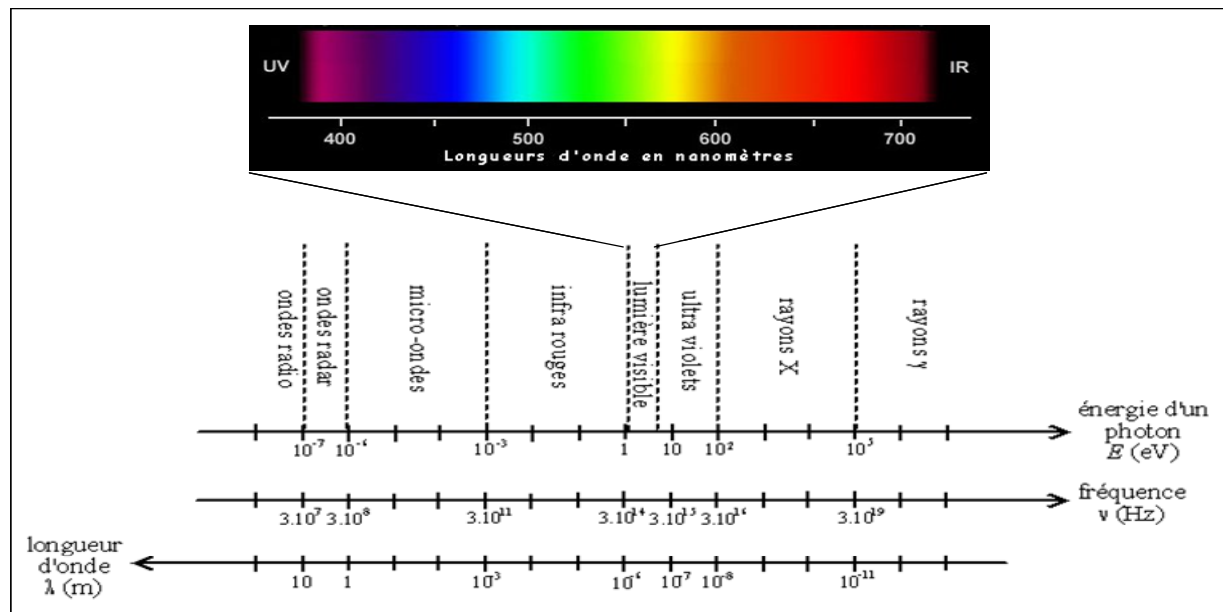
Figure IV.1 : Spectre électromagnétique
