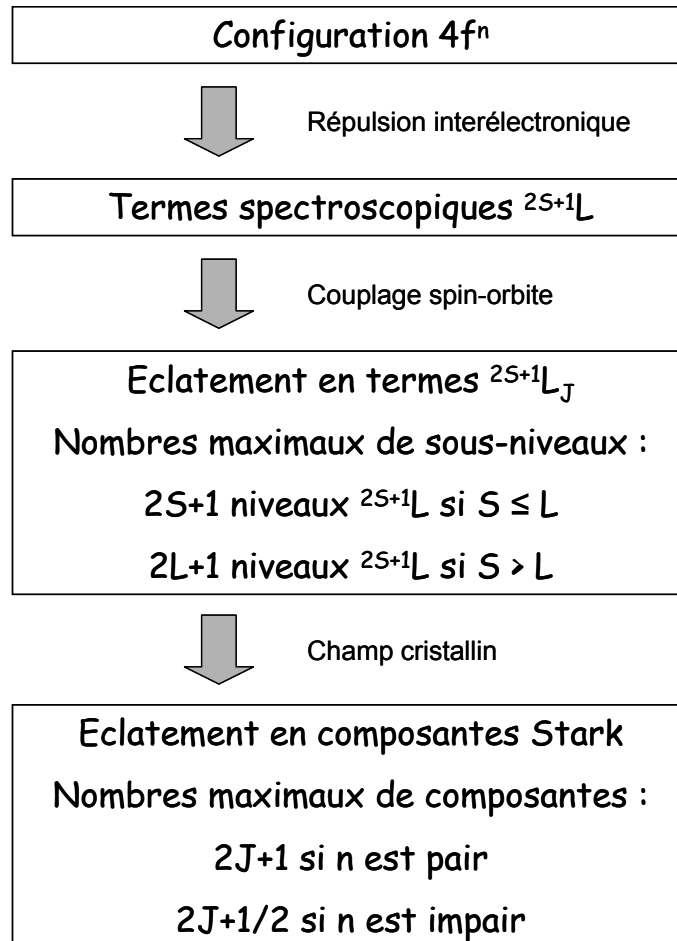
Figure IV.4 : Perturbations dans l'hamiltonien H
