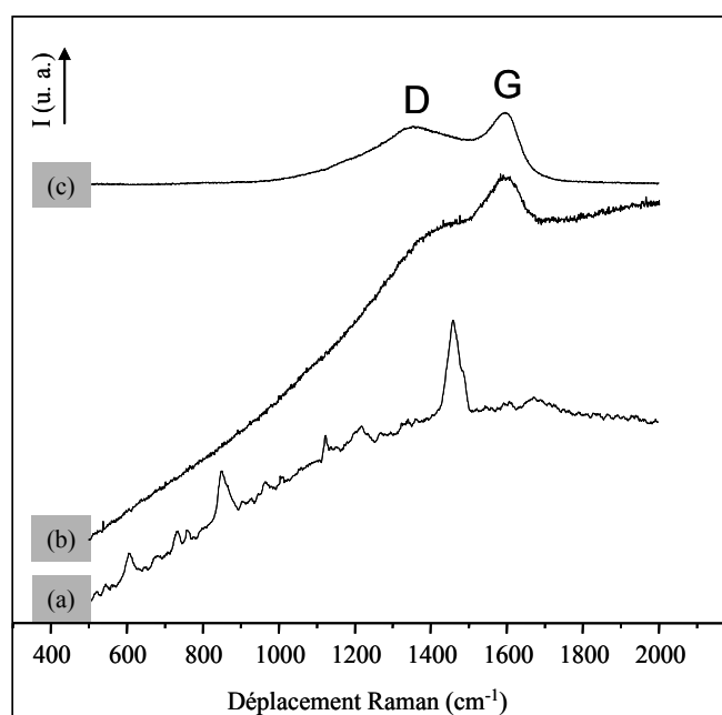
Figure II.39 : Spectres de diffusion Raman de \text{LiGdF}_4 (a) xérogel, (b) traité à 300°C et (c) à 500°C sous \text{N}_2
