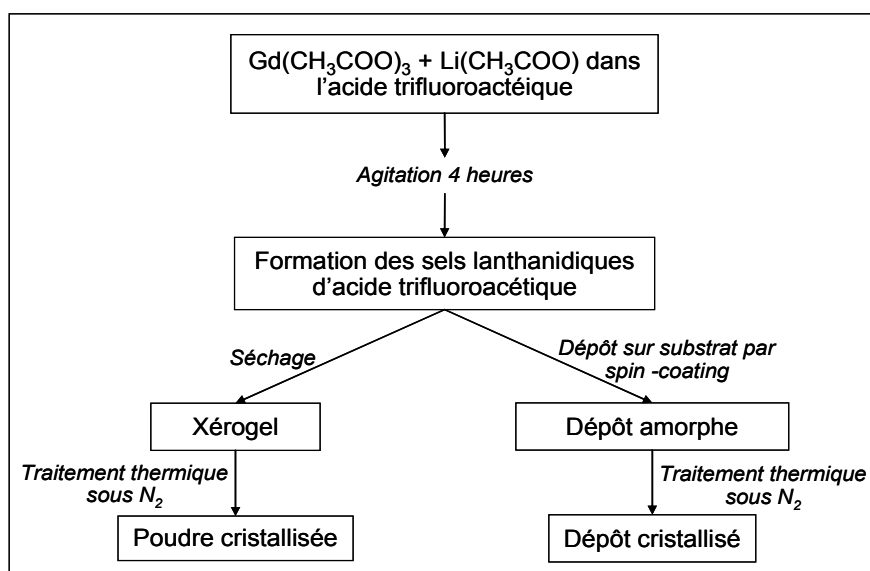
Figure II.34 : Schéma du protocole de synthèse pour l'élaboration de fluorures de formulation \text{LiGdF}_4 à partir d'acétates métalliques
