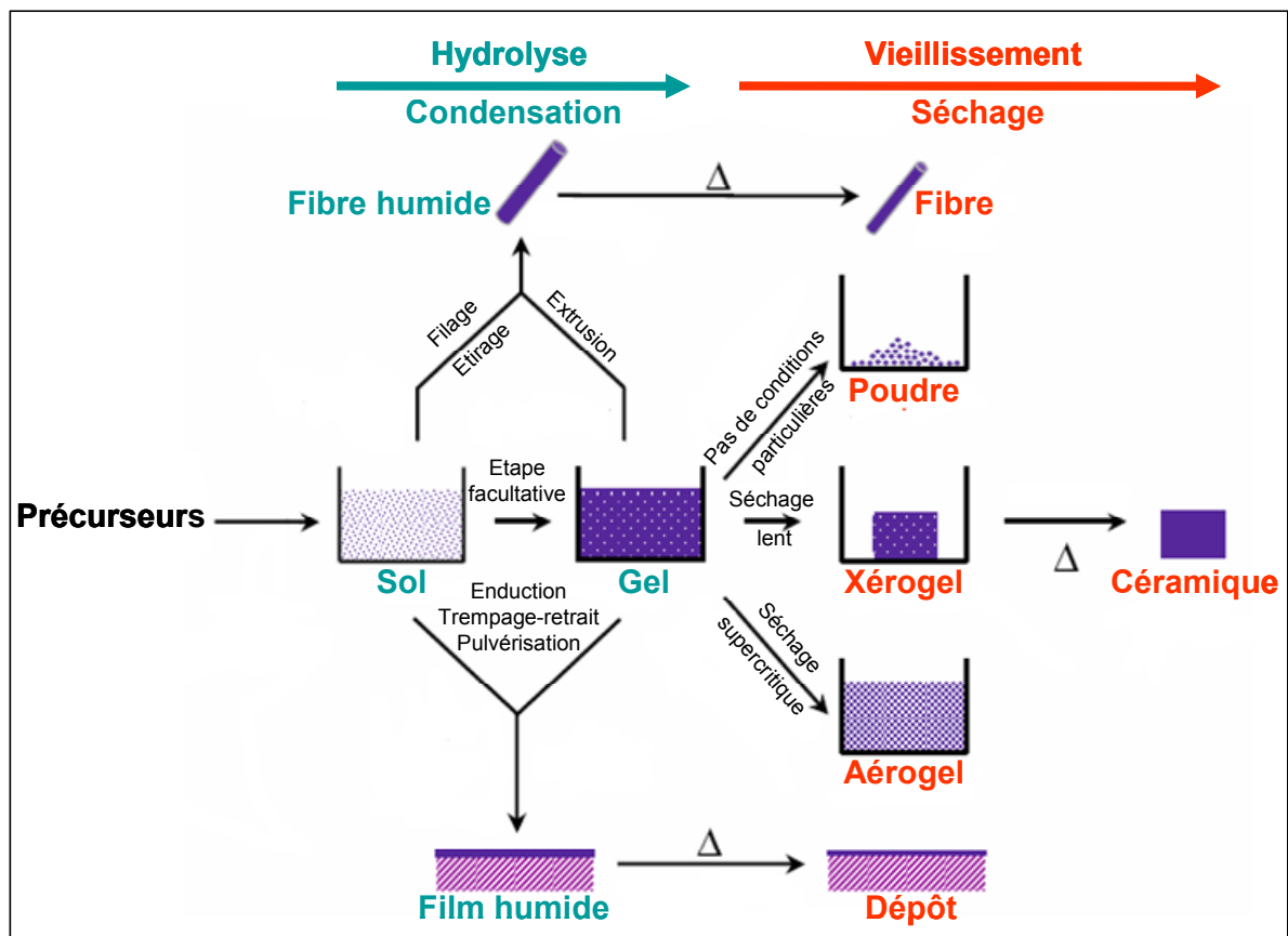
Figure I.16 : La transition sol-gel et ses produits
