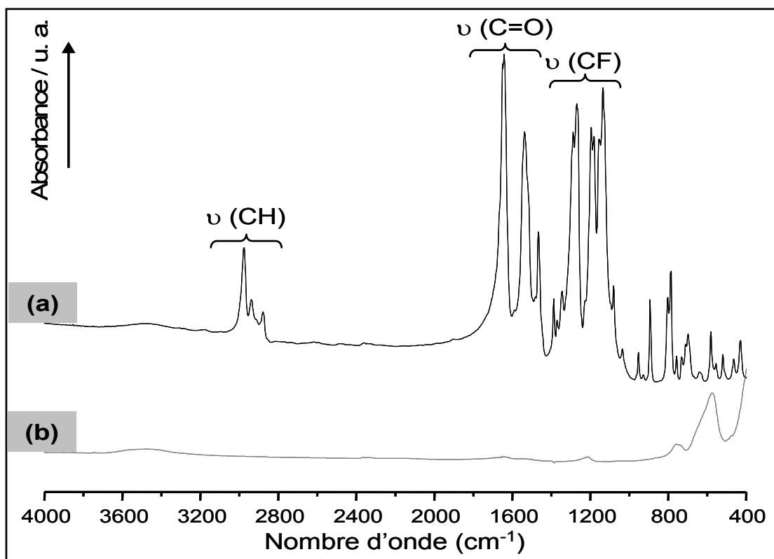
Figure II.56 : Spectres IR du composé Na 1,5 Gd 1,5 F 6 (a) xérogel et (b) traité à 550°C
