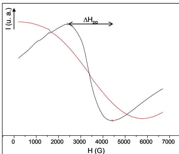
Figure II.17 : Spectres RPE des échantillons \text{LiGdF}_4 xérogel (courbe noire) et traité à 550^\circ\text{C} (courbe rouge) sous \text{F}_2
