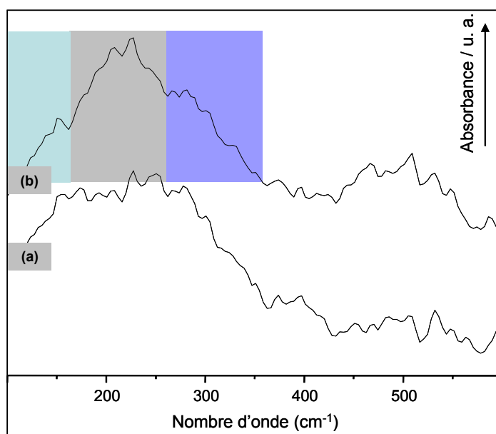
Figure II.57 : Spectres en infrarouge lointain (a) du xérogel de NaGdF 4 et (b) du composé cristallisé traité à 550°C sous F 2
