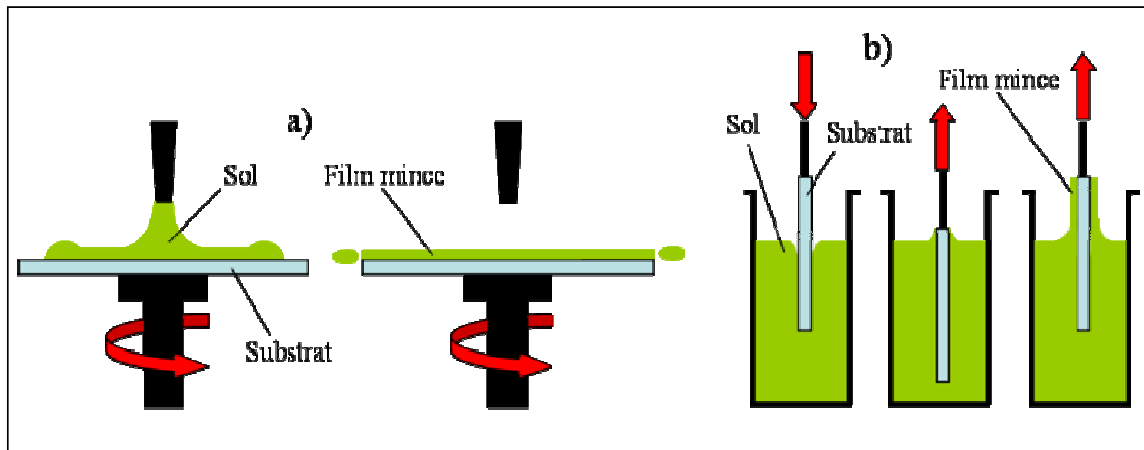
Figure I.17 : Schéma représentant le principe a) de l'enduction centrifuge et b) du trempage-retrait pour la préparation de film mince 1
