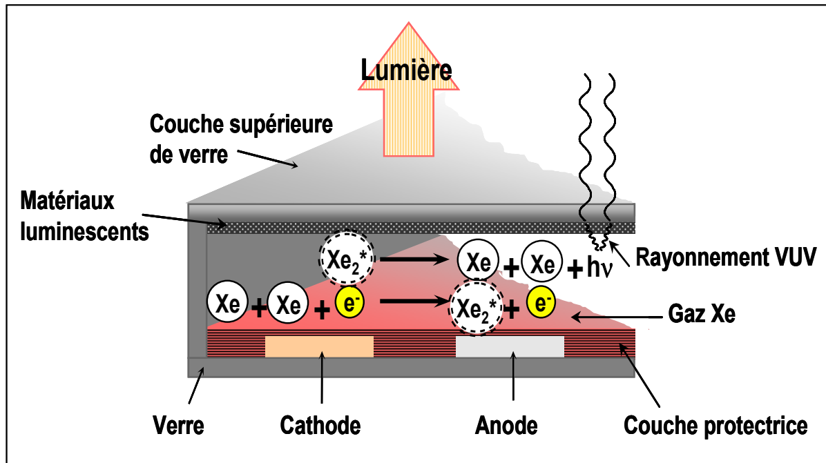
Figure I.5 : Représentation schématique d'une lampe à décharge de xénon
