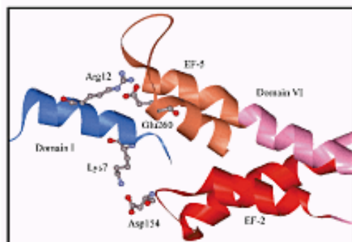
Figure N°9: Structure schématique 3D des domaines I et VI de la m-calpaïne humaine en absence de calcium. Les résidus Lys7 et Arg12 (en bleu) du domaine 1 interagissent respectivement avec les résidus Asp154 dans la boucle du motif EF-hand 2 (rouge) et Glu260 de l' \alpha -hélice du motif EF-hand 5 (orange) du domaine VI de la petite sous-unité (Nakagawa et al. , 2001).
