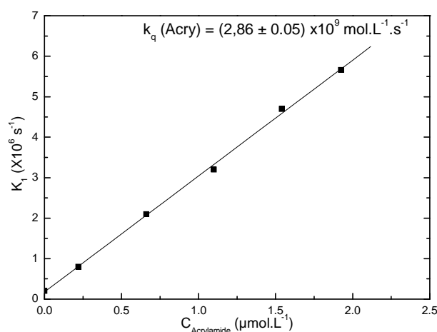
Figure A-58 : Evolution de constante de disparition du triplet du cyanophos _1 , k_1 , en fonction de [acrylamide]. [CYA] = 1,1 \times 10^{-4} \text{ mol.L}^{-1} , \text{pH} = 5,5 , milieu désoxygéné.
