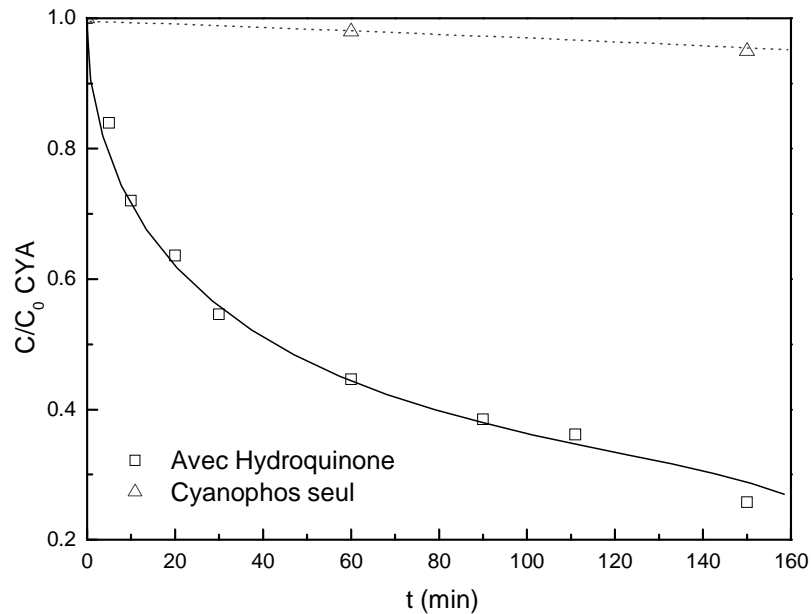
Figure A-79 : Cinétiques de dégradation du CYA en absence et en présence d'HQ ([HQ] = 9 \times 10^{-4} mol.L -1 ), \lambda_{excitation} = 300 nm.
