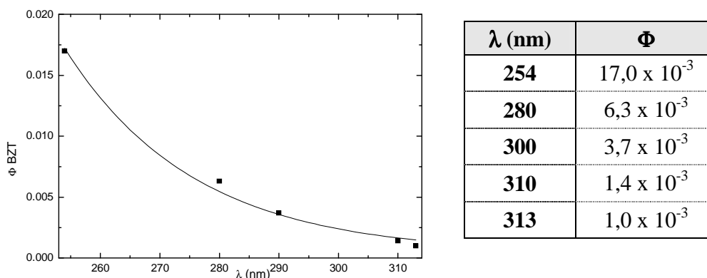
Figure A-38 : Evolution du rendement quantique de BZT en fonction de longueur d'onde d'excitation, milieu aéré, pH = 11.
