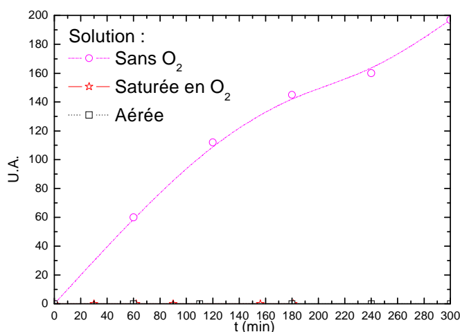
Figure 0-7 : Effet de l'oxygène sur la formation du 4 CDT. Irradiation d'une solution de CYA ( C = 1,2 \times 10^{-4} \text{ mol.L}^{-1} , \text{pH} = 5,3 ) à 310\text{nm} .
