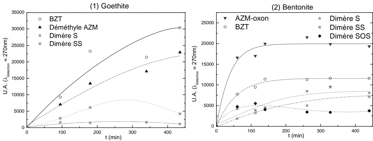
Figure B-38 : Cinétiques d'apparition des photoproduits de l'AZM dans la goethite (1) et la bentonite (2). Irradiation en Suntest (765 W/m 2 , 15°C), Z = 23 μm, 1,3 mg d'AZM par g de support. \lambda_{\text{detection}} = 270 \text{ nm} .
