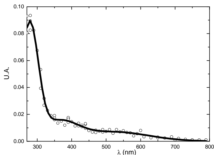
Figure A-55 : Spectre d'absorbance de T_1 , en présence de N_2O , juste après l'impulsion laser.
