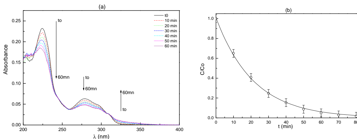
Figure A-37 : Photodégradation de l'AZM dans l'eau à 254 nm, [BZT]=1,2 \times 10^{-5} \text{ mol.L}^{-1} , milieu aéré, pH=5,7.
