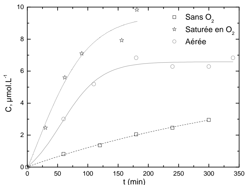
Figure A-73 : Effet de l'oxygène sur la vitesse de formation du cyanophénol. [CYA] = 1,2 \times 10^{-4} \text{ mol.L}^{-1} , pH = 5,3 , à 310 \text{ nm} (polychromatique 280 - 350 \text{ nm} ).
