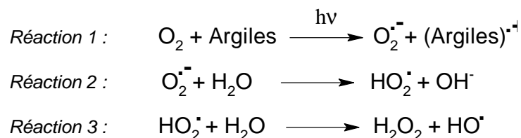
Figure B-9 : Production de radicaux Hydroxyles à partir de l'irradiation d'une argile, [141].
