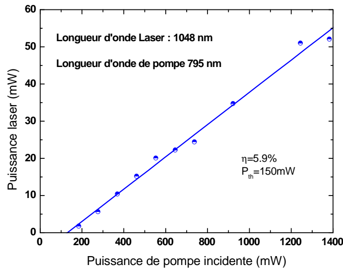
Figure II.F.6 : Courbe de rendement laser en pompage Sa :Ti d'un cristal de \text{CaF}_2 : 2\%\text{Yb}^{3+} , 1\%\text{Nd}^{3+} , e_p = 5\text{mm} .
