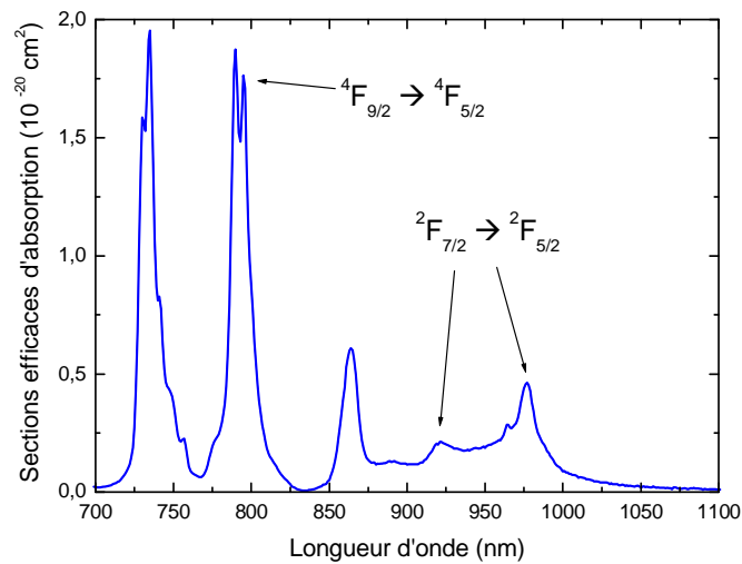
Figure II.F.2 : Spectre d'absorption à température ambiante d'un cristal de CaF 2 :1% Nd 3+ ,2% Yb 3+ .
