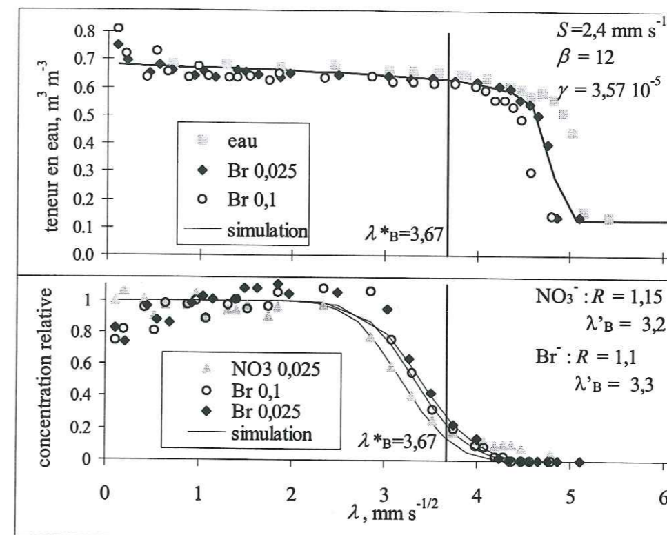
Figure III-13 : Profils de teneurs en eau et de concentrations adimensionnelles, mesurés et calculés.
