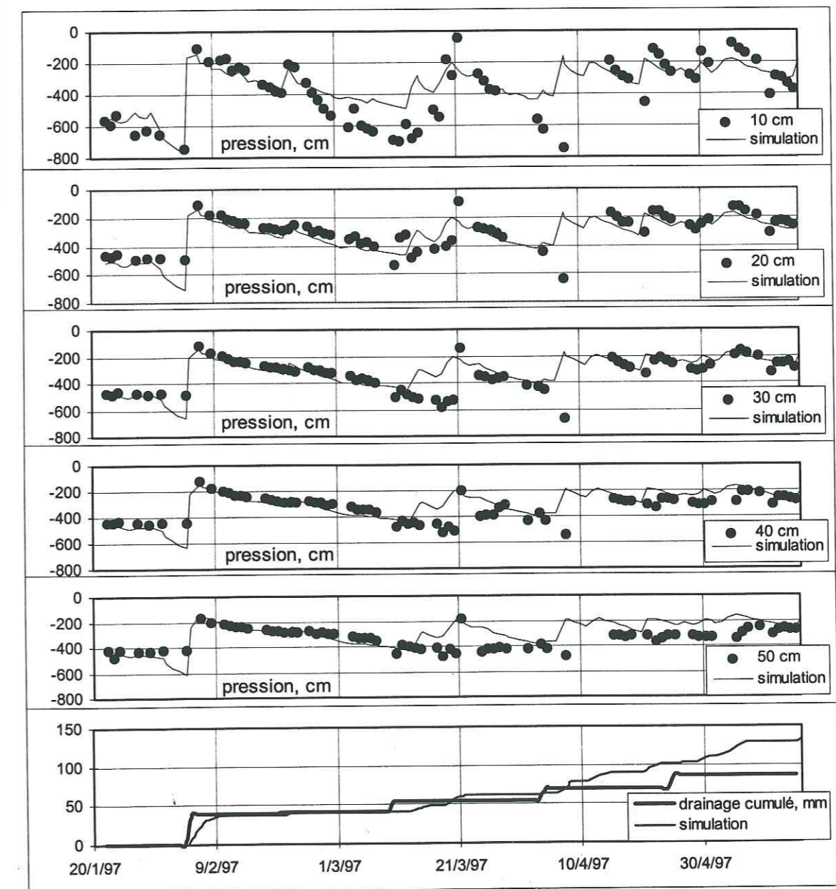
Figure V-8 : Pressions mesurées et simulées, drainage cumulé calculé et simulé, sur la parcelle B en 1997
