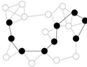
FIG. 2.3 – La construction d'un ensemble dominant connecté.
