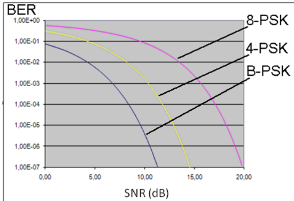
Figure 2. 19 Evolution du BER en fonction du SNR pour 3 types de modulation
