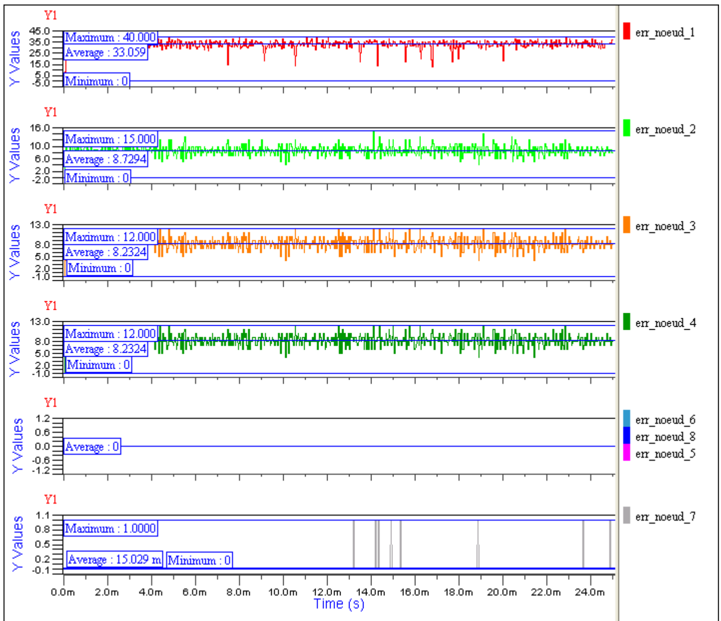
Figure 3.3 Nombre d'erreurs par frame, première simulation
