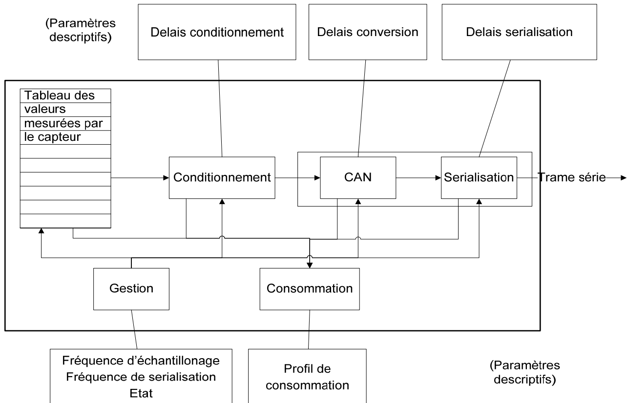
Figure 2. 3 Modèle général du capteur
