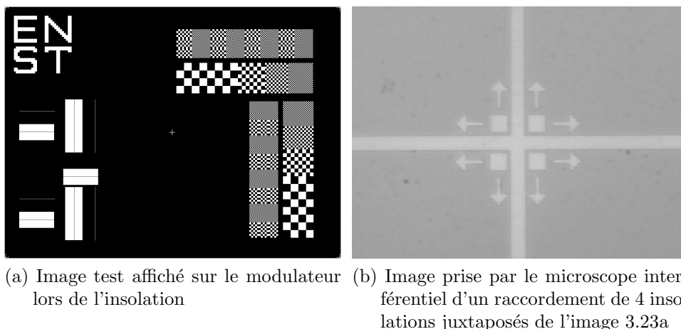
FIGURE 3.23 – Élimination de l'effet de bord de SLM avec le micro-écran Epson à comparer à la figure 3.12.
