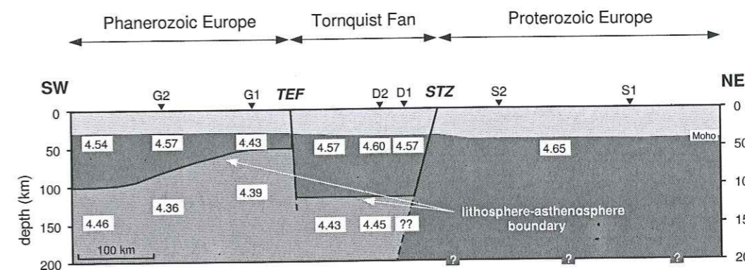
FIG. 1.4 – Coupe d'échelle lithosphérique le long du réseau TOR d'après l'analyse des ondes de surface [Cotte & Pedersen, 2002].
