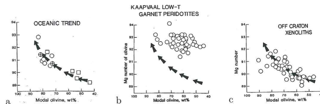
FIG. 1.2 – Différences géochimiques entre a) une séquence de résidus de basaltes océaniques; b) les xénolites du craton Kaapvaal et c) des xénolites trouvées hors craton. L'abscisse est la quantité d'olivine modale dans les échantillons en pourcentage du poids, l'ordonnée est le rapport Mg/(Mg+Fe) [figure 1, 2 et 4 de Boyd, 1989].
