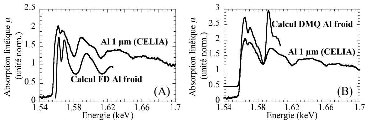
FIGURE 4.22 – (A) Comparaison des spectres d’absorption de l’aluminium froid mesuré et calculé par la méthode FD, développée au CELIA par Olivier Peyrusse [9]. (B) Comparaison des spectres d’absorption de l’aluminium mesuré et calculé par le code DMQ, développé au CEA par V. Recoules et S. Mazevet [11].
