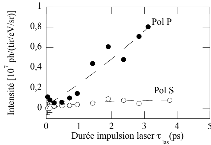
FIGURE 3.9 – Intensité maximale de la raie He_{\alpha} en fonction de la durée d’impulsion laser pour des polarisations P et S et pour une cible polie. L’énergie sur cible est de 3.75 mJ. L’incertitude sur la mesure est comprise dans la grosseur de points.
