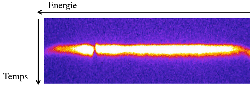
FIGURE 3.26 – Spectre d'émission de l'erbium résolu en temps, obtenu pour une durée \tau_{las} = 2.7 ps, pour E_{las} \sim 5 mJ et pour une accumulation de 360 s au kHz.
