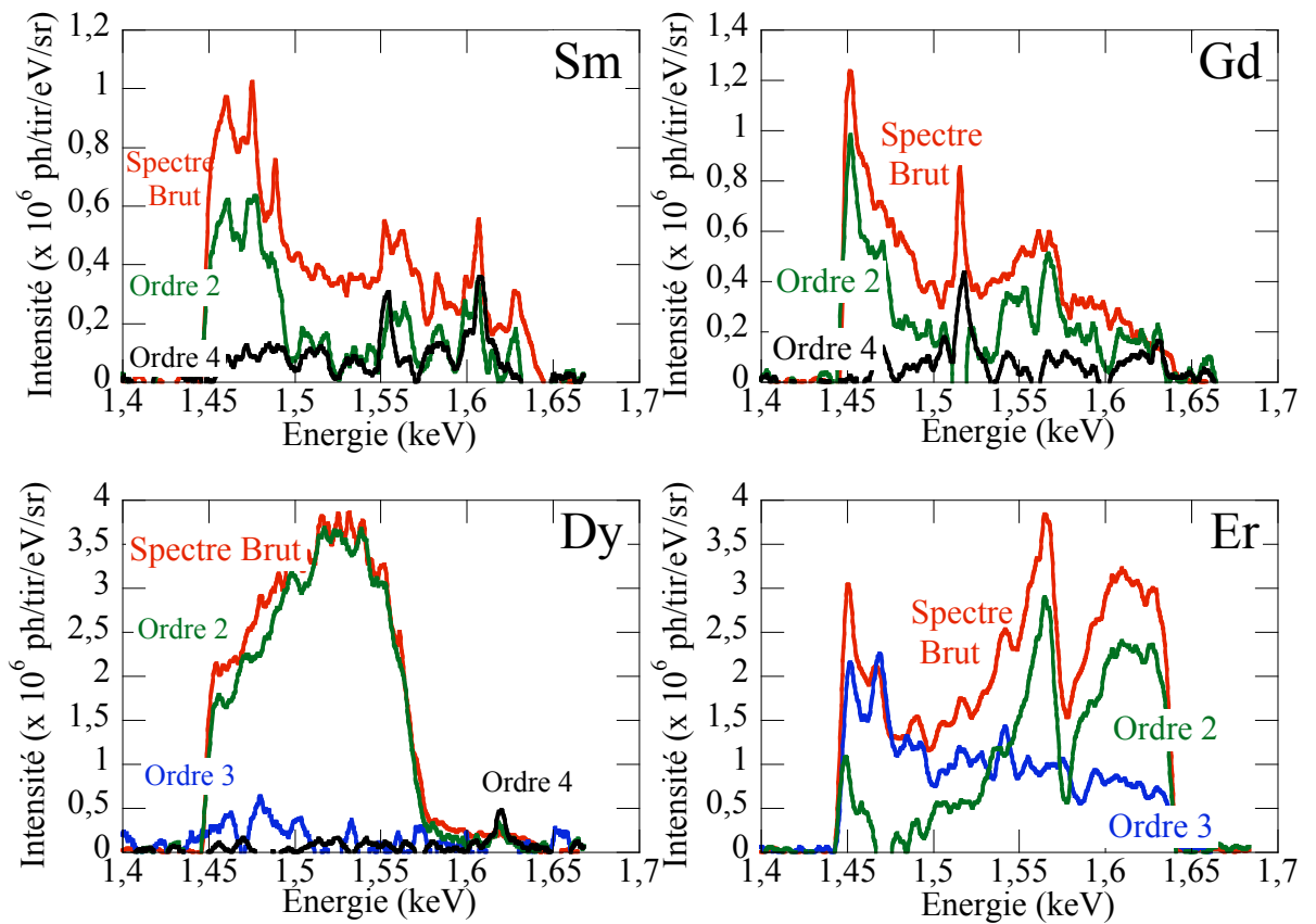
FIGURE 2.19 – Spectres des ordres 2 et supérieurs des émissions du Sm, Gd, Dy et Er, réalisés avec le spectromètre MICA et corrigés selon la formule 2.16. Les paramètres lasers utilisés sont E_{las} = 3.7 \text{ mJ} et \tau_{las} = 3 \text{ ps} .
