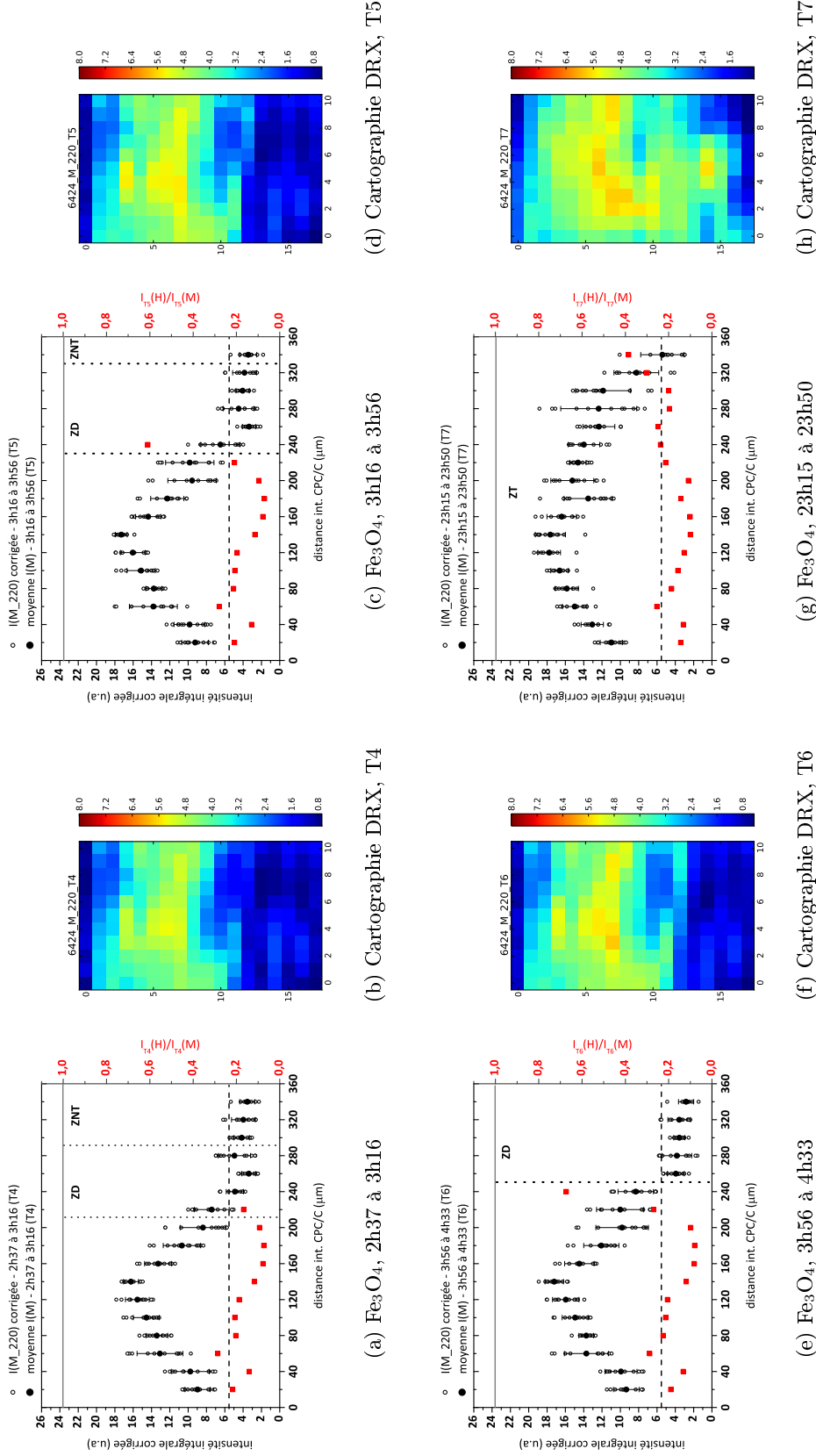
Fig B.16 – Evolution structurale de \text{Fe}_3\text{O}_4 entre 2h37 et 23h50 de traitement en milieu aéré, SM9-6424, zone AOI-01 ; la ligne horizontale 0 équivaut à l'interface CPC / Canal, taille du pixel = 100 \times 20 \mu\text{m}^2
