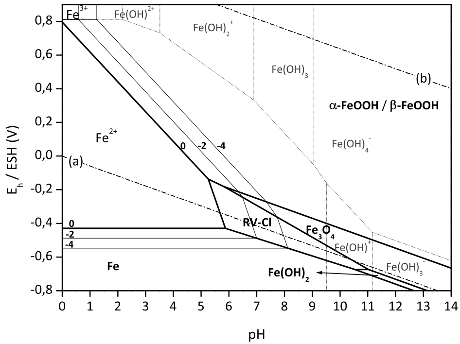
Fig 4.8 – Diagrammes de Pourbaix E-pH du fer en milieu chloruré à 25°C ; a(Cl^-) = 0,35 et différentes activités de Fe^{2+} en présence de l'ensemble des phases rencontrées durant l'étape de traitement, domaine de stabilité de l'eau compris entre les droites (a) et (b)
