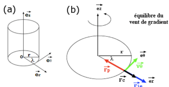
Figure 1.7 – (a) Repère cylindrique, (b) Equilibre des forces définissant le vent gradient. Cet équilibre est vérifié à l'extérieur du mur de l'œil.
