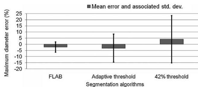
Fig. 6. Erreur moyenne et écart-type par rapport au diamètre de la tumeur mesuré en histologie, pour l'ensemble des 18 tumeurs et les différentes approches de segmentation des images.
