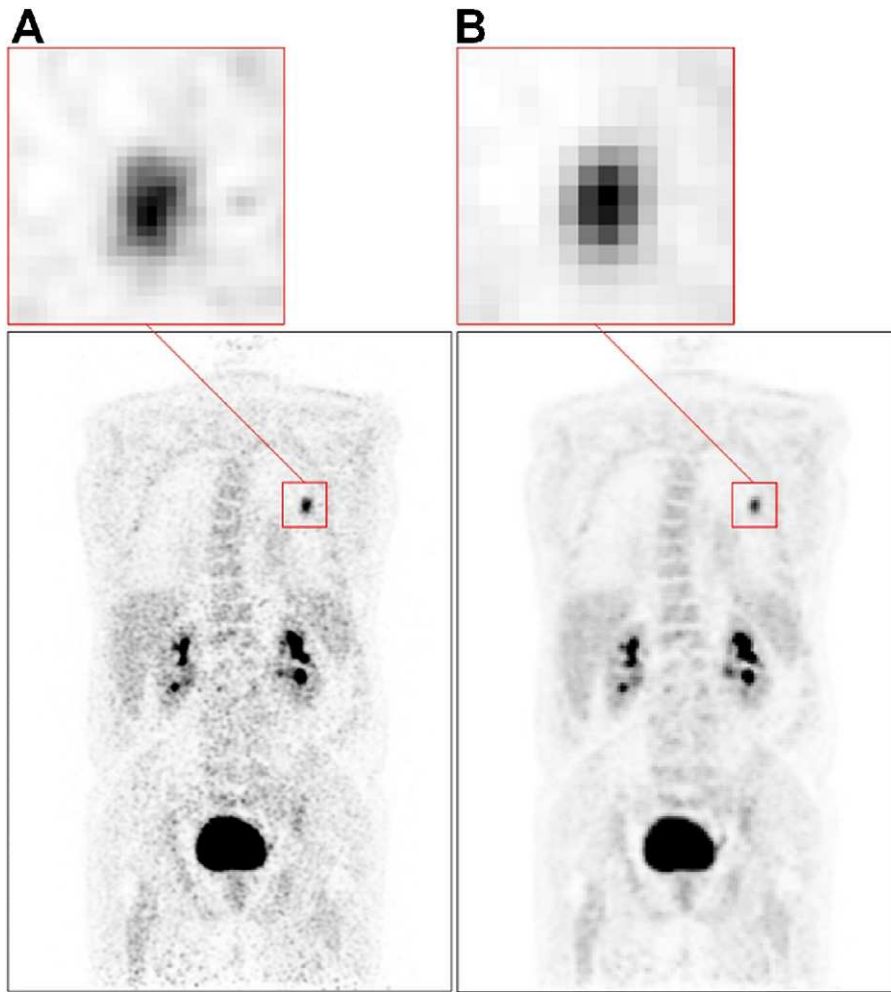
Fig. 2. Acquisition de tomographie par émission de positons (TEP) corps entier au (^{18}\text{F})\text{-FDG} reconstruite avec des voxels de A : 2 \times 2 \times 2 \text{ mm}^3 et B : 4 \times 4 \times 4 \text{ mm}^3 .
