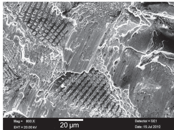
Fig 14. Image MEB qui montre l'état des micro-grilles après déformation à 1050°C et 10s-1, les micro-grilles s'avèrent inexploitablement pour déterminer des champs de déformation.
