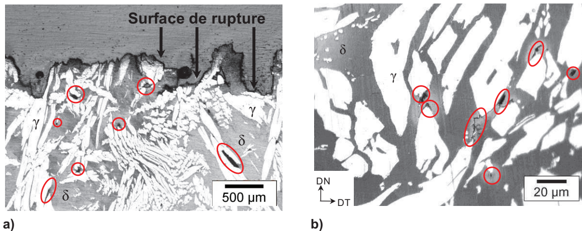
Fig 8. Micrographies optiques qui montrent que les cavités germent par décohésion partielle au niveau des interfaces \delta/\gamma et que les fissures ne se propagent jamais dans la phase austénitique; a) micrographie proche de la rupture d'une éprouvette pré-entallée; b) micrographie proche des rives, c'est-à-dire des zones endommagées sur une tôle industrielle. Les sites d'endommagement sont entourés en rouge.
