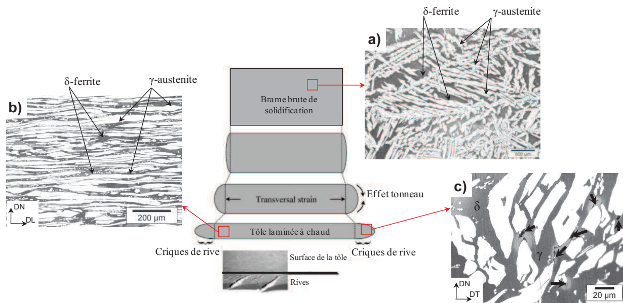
Fig 3. Illustration avec l'acier D2 des microstructures présentes aux différentes étapes du procédé de laminage à chaud industriel ; a) microstructure typique de la brame brute de coulée ; b) microstructure typique au centre de la tôle laminée à chaud avec un alignement des îlots d'austénite dans la direction de laminage ; c) microstructure de la tôle laminée proche des rives (zone endommagée) les cavités sont pointées par des flèches.
