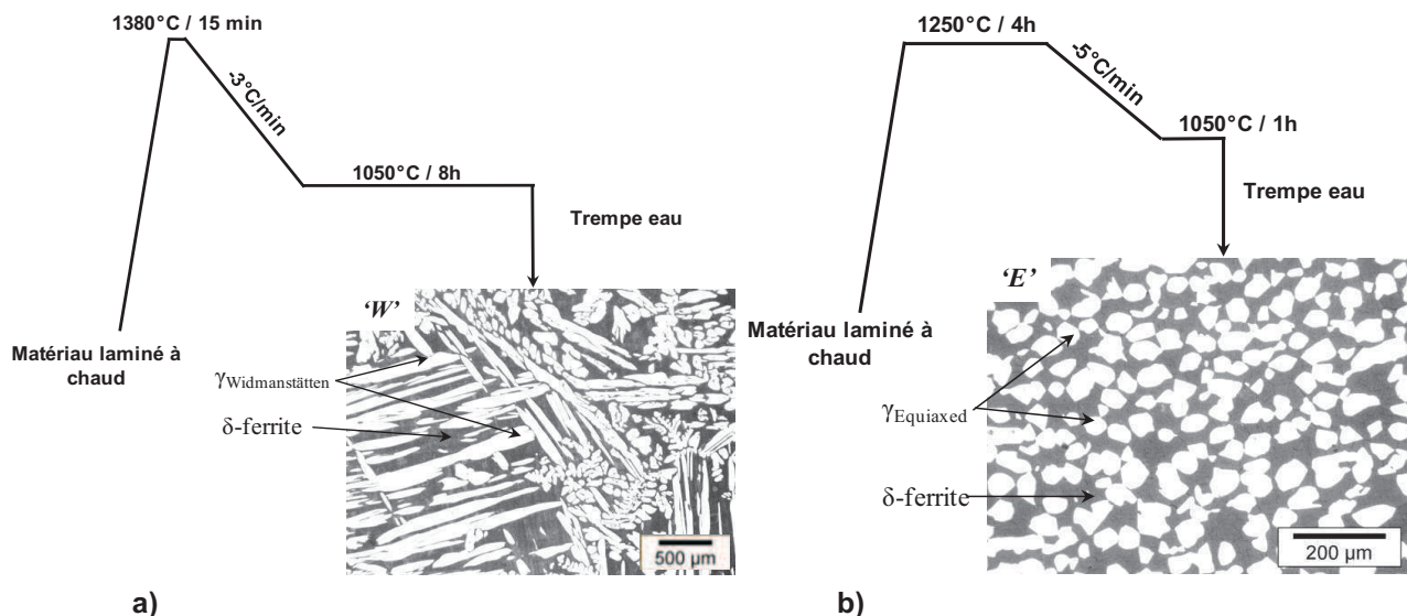
Fig 9. Chemins thermiques permettant de générer des microstructures modèles, exemple avec l'acier D2; a) chemin thermique pour fabriquer une morphologie d'austénite de Widmanstätten; b) chemin thermique pour générer une austénite équiaxe.
