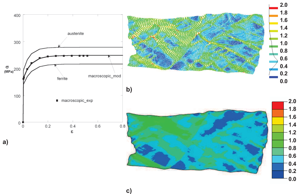
Fig 15. Quelques résultats obtenus sur l'acier D2 avec la stratégie développée en collaboration avec l'Université catholique de Louvain (échantillon déformé à 850°C et 1s -1 ) ; a) courbe contrainte-déformation macroscopique de l'acier D2 et rhéologies de la ferrite et de l'austénite déterminées via l'approche développée ; b) champ de déformation expérimental ; c) champ de déformation simulé.
