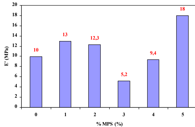
Figure III. 34: Evolution du module de conservation E' du matériau nanocomposite (contenant 4 % whiskers) en fonction du taux de MPS à une température de 50°C
