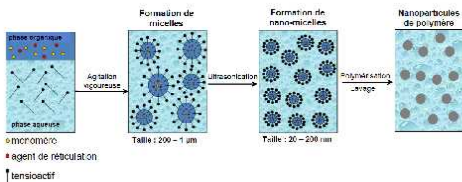
Figure III. 1: Mécanisme de la polymérisation en miniémulsion
