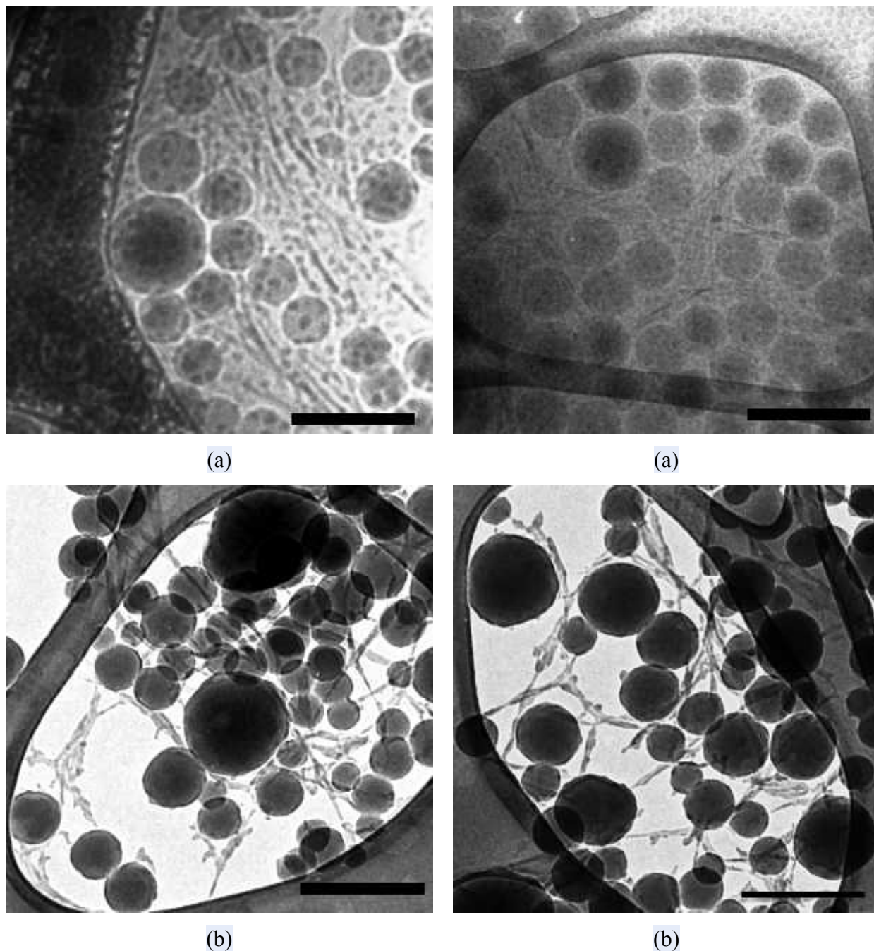
Figure III. 20: Observation par microscope électronique à transmission (a) de dispersion de nanocomposites contenant 2% en masse de nanocristaux d'alfa, (b) dispersion de nanocomposite contenant 2% de nanocristaux d'alfa, en présence de silane.
