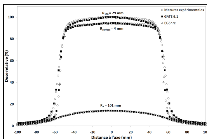
Figure IV-11 : Comparaison des profils de dose dans l'eau pour le faisceau de 20 MeV (DSP 108 cm, 10 \times 10 cm 2 ) à différentes profondeurs ( R_{surface} = 4 mm, R_{100} = 29 mm et R_p = 101 mm) mesurés par diode et simulés avec GATE 6.1 et EGSnrc.
