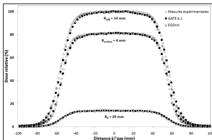
Figure IV-10 : Comparaison des profils de dose dans l'eau pour le faisceau de 6 MeV (DSP 108 cm, 10 \times 10 cm 2 ) à différentes profondeurs ( R_{surface} = 4 mm, R_{100} = 14 mm et R_p = 29 mm) mesurés par diode et simulés avec GATE 6.1 et EGSnrc.
